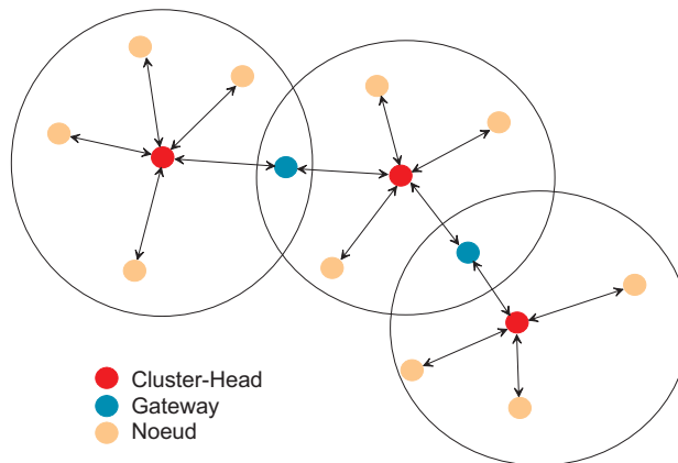
Figure 2.14 – Les différents types de noeuds dans le protocole CBRP
