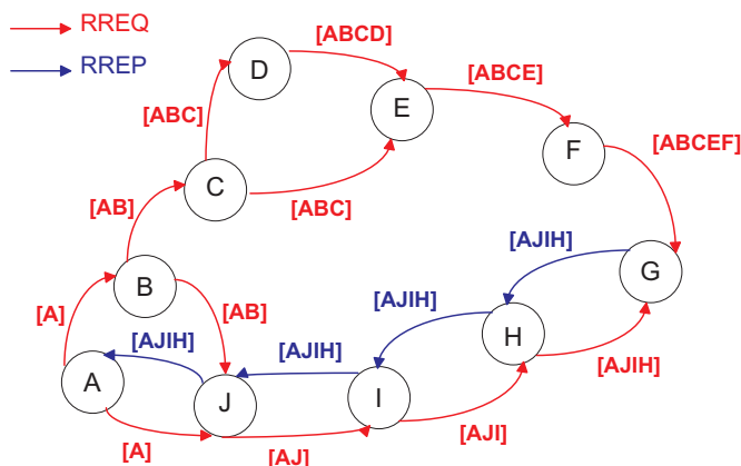
Figure 2.11 – Le principe de découverte de route dans le protocole DSR
