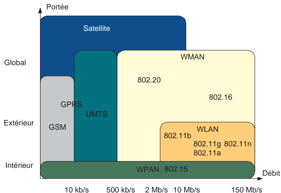
Figure 2.1 – La portée et le débit des différents standards de communication sans fil [Pujolle 03]
