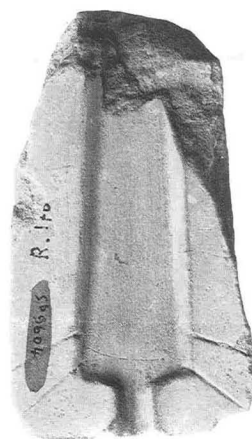
172. Suse. Moule de flèche de type F 2.E. Grès (D'après Tallon 1987 (B), p. 345.II).
