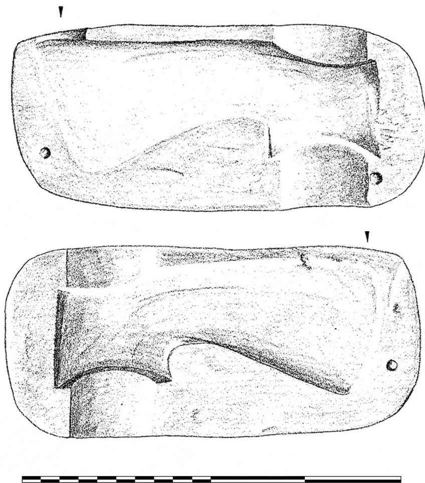
132. Kültepe. Acropole. Moule hache à collet (type H 2) (BA final). (D'après Müller-Karpe 1994, pl. 41.1 et Özgüç 1986, pl. 89.2a-b).
