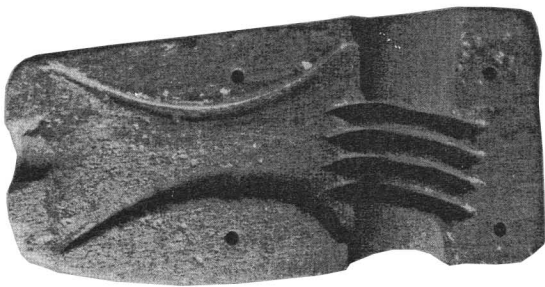
136. Kültepe. Karum Ib. Moule de hache à collet H 2.O.g. (D'après Ozgüç 1986, pl. 134.2b). Echelle approximative.
