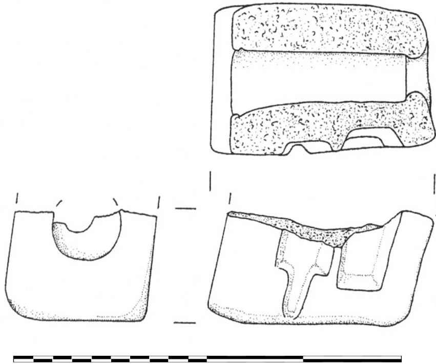
177. Tell Brak. Moule en grès pour plusieurs objets dont un poignard (2100-2000 av. J.-C). (D'après McDonald et al. 2001, p. 581, fig. 482.169).
