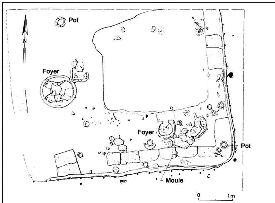
18a. Norsuntepe. Atelier du niveau XIX (2700 av. J.-C.). (D'après Müller-Karpe 1994, p. 29, fig. 13).
