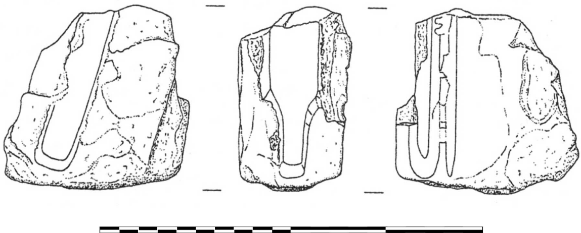
178. Tell Brak. Moule en grès pour plusieurs objets dont un poignard (2150 av. J.-C). (D'après McDonald et al. 2001, p. 581, fig. 482.170).
