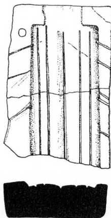
184. Tell el-Dab'a. Str. G/1-3. En contexte secondaire : probablement G/4 à l'origine, dans la partie artisanale du palais (Philip 2006, p. 195). (BM I). Deux fragments d'une moitié de moule bivalve en stéatite ou chlorite. Matrice pour poignard nervuré de type P 8.A.a. (D'après Philip 2006, p. 195, fig. 78.1).
