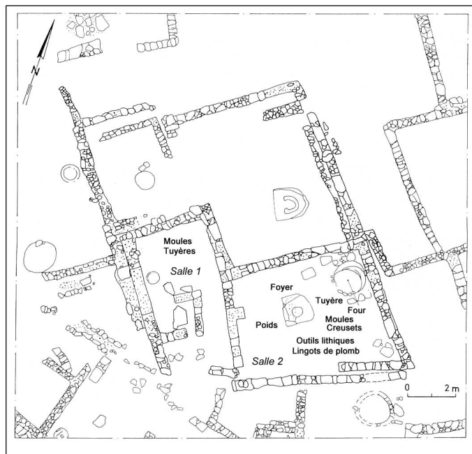
85. Kültepe. Plan de l'atelier 7 du karum (niveau II). (D'après Müller-Karpe 1994, p. 51, fig. 29).
