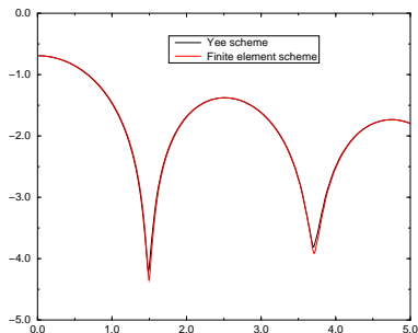
FIG. 10.5 – Amortissement de l'énergie du mode principal du champ électrique.
