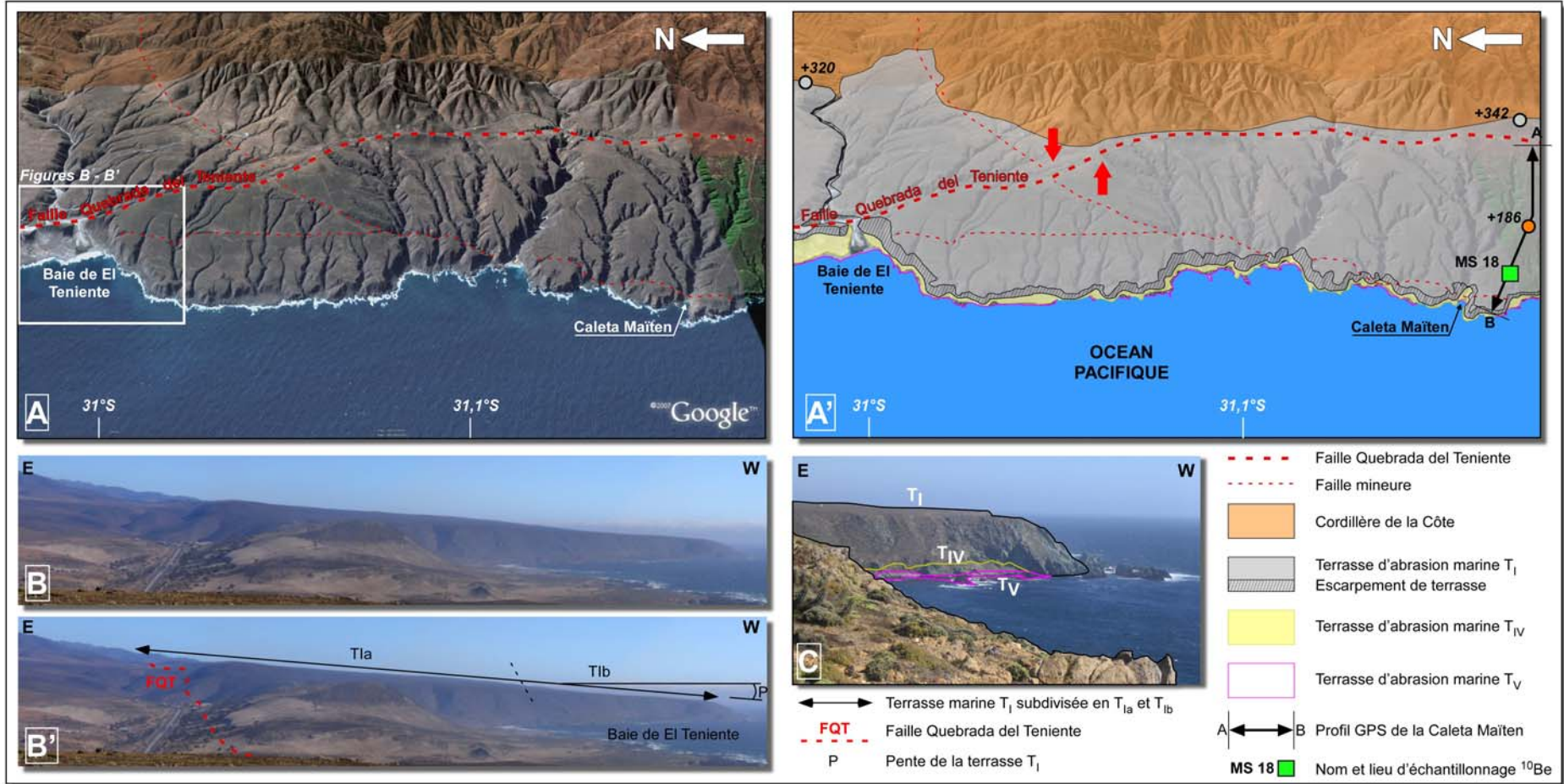
Figure 46 : A – Image satellite issue de Google Earth de la zone au sud de la Baie de El Teniente (31°S). A' – Cartographie de la morphologie côtière dans cette même zone. Au sud de 31°S, on distingue trois niveaux de terrasses marines seulement : T_V , T_{IV} et T_I (composite). Les chiffres associés aux cercles correspondent à l'altitude des pieds de falaise : +320 m à T_I , +342 m à T_{Ia} et +186 m à T_{Ib} . B et B' – Panorama de la terrasse marine composite T_I . A noter, la forte pente de T_I vers la mer. C – Photographie de l'escarpement de T_I qui plonge parfois directement dans la mer. Photographie prise vers le Sud et depuis le cap au sud de la Caleta Maïten.
