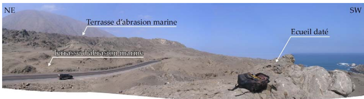
Figure 82 : Panorama d'une section du cap entre Tanaka et la baie de Chala, au sud de la ville de Tanaka. On y observe les différents niveaux de terrasses d'abrasion marine et les nombreux écueils rocheux présents sur les terrasses.
