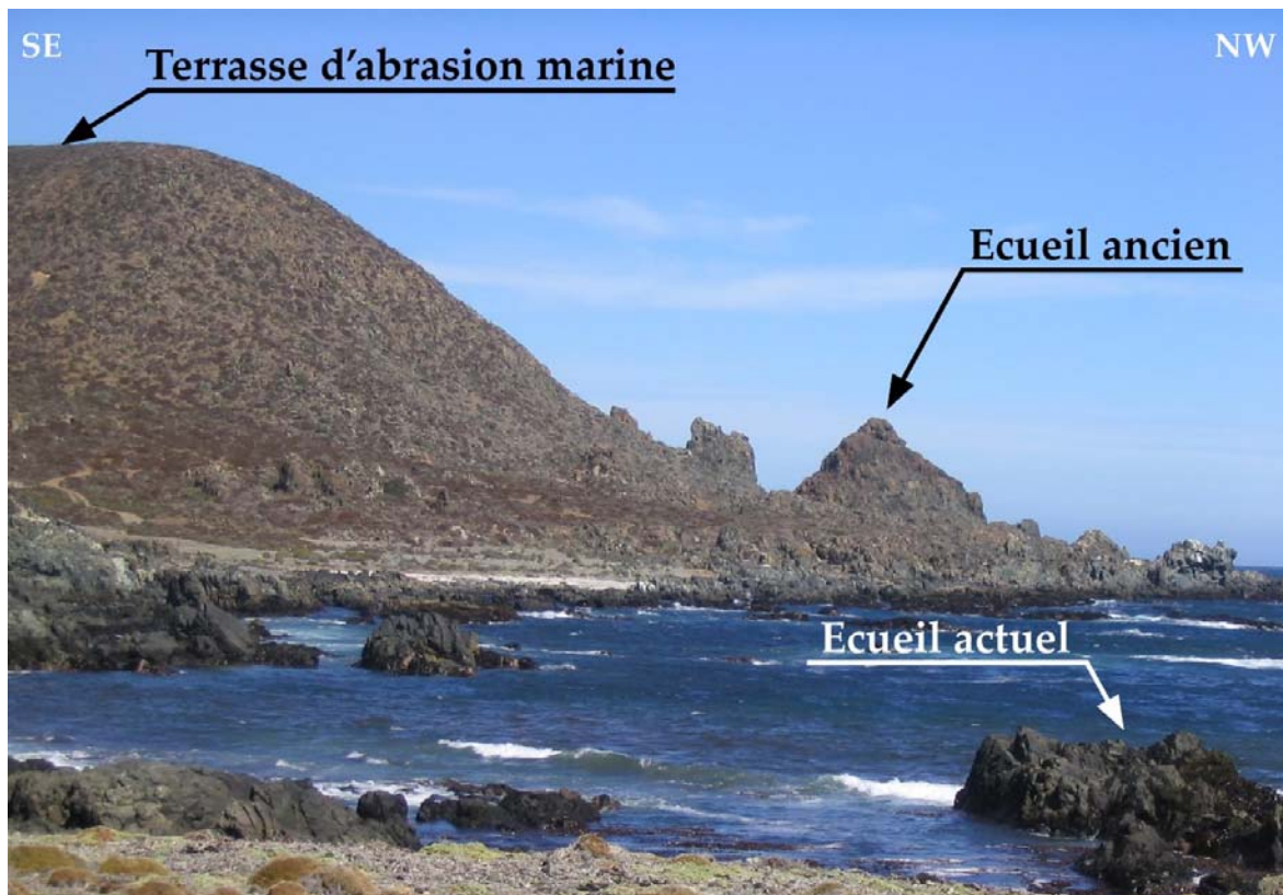
Figure 24 : Photographie d'écueils rocheux. L'écueil rocheux est dit actuel quand sa base est encore immergée et soumise à l'érosion marine. L'écueil rocheux ancien a été soulevé avec la terrasse marine qui le porte et préservé. Enfin, on peut observer dans le quart en haut à gauche de la photographie, un niveau de terrasse d'abrasion marine avec son escarpement et sa surface plane.
