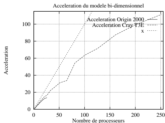
FIG. 10.8 – Accélération comparées selon la machine cible pour le modèle bi-dimensionnel
