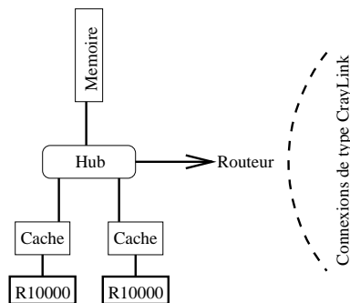
FIG. 7.3 – Architecture simplifiée d'un noeud de l'ORIGIN 2000 à 32 processeurs
