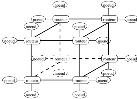
FIG. 7.2 – Architecture simplifiée de l'ORIGIN 2000 à 16 noeuds et 32 processeurs
