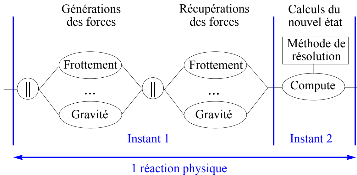
FIG. 7.5 – Les deux phases d'une r action physique  l mentaire
