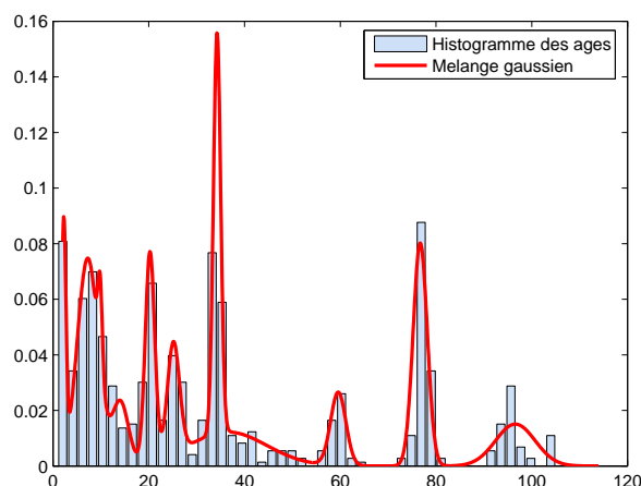
FIG. 3.16 – Estimation de l'histogramme des âges par mélange gaussien
