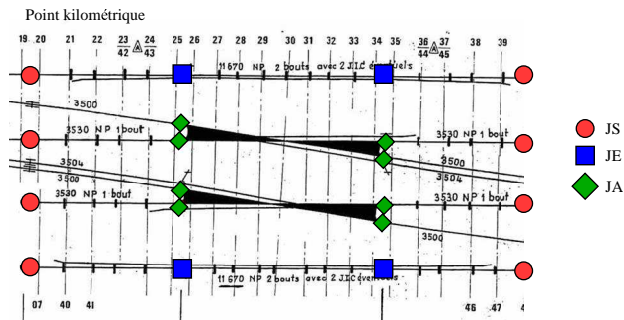
FIG. 2.3 – Exemple d'appareil de voies
