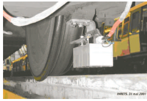
FIG. 1.5 – Le capteur à courants de Foucault monté sur une voiture d'inspection [Aknin et al., 1992]
