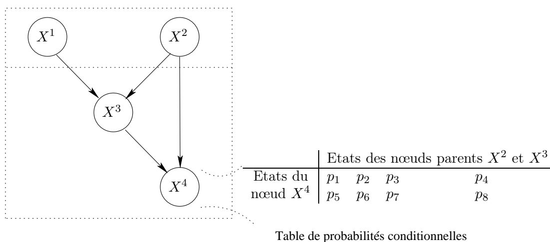
FIG. 2.11 – Exemple d'un Réseau Bayésien
