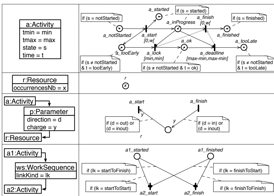
FIGURE 6.5: Schéma de traduction de xSPeM vers PETRINET
