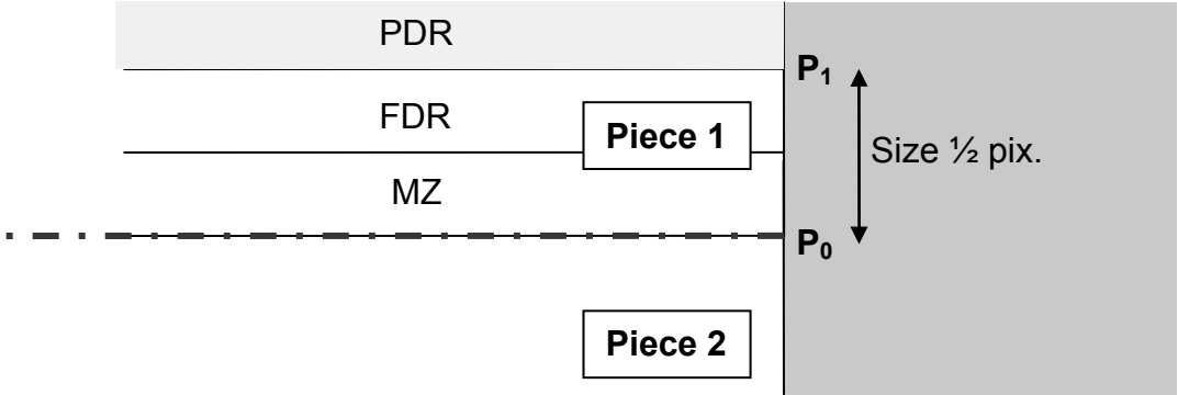
Figure 88: Détail du bas du maillage: épaisseur des différentes zones et position des points P_1 et P_0 .
