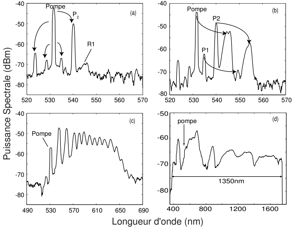
Fig. A.4 Spectres de sortie de la fibre PCF 4 pour une puissance de pompe croissante. (a) processus paramétriques, (b) double diffusion Raman stimulée, (c) cascade Raman ( P = 1 \text{ mW} ), (d) SC de 1350 nm pour une puissance moyenne injectée de 20 mW.
