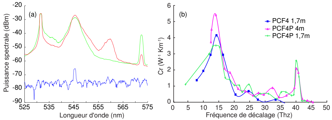
Fig. B.7 (a), dans la fibre PCF 4 P de 4m, en plaçant un signal (bleu) sur le premier ordre Raman de la pompe (vert), on fait apparaître le deuxième ordre Raman sur le signal amplifié (rouge). (b), mesure du spectre de gain Raman dans trois PCF (PCF 4 de 1,7 m, PCF 4 P de 1,7 m et 4 m) avec un signal issu d'un continuum généré dans une fibre DSF.
