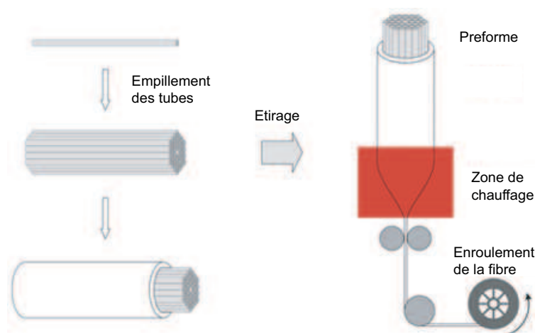
Fig. 2.3 Illustration de la méthode de fabrication d'une PCF par étirage.
