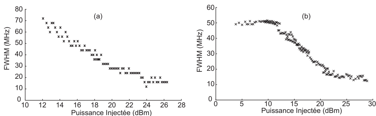
Fig. 4.15 Largeur à mi-hauteur du pic principal du spectre Brillouin dans la fibre (a) PCF 4 et (b) PCF 4 P en fonction de la puissance injectée.
