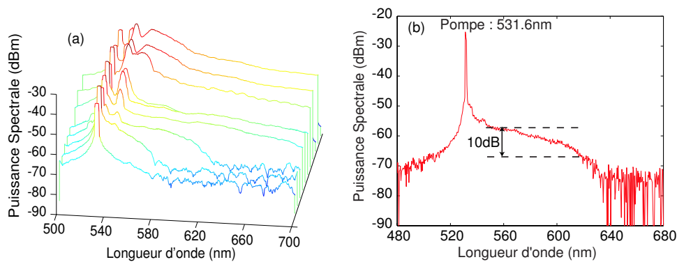
Fig. A.3 (a), spectres de sortie pour une puissance d'entrée variant de 0,5 à 4 mW. (b), élargissement de 80 nm du côté des grandes longueurs d'onde d'une amplitude de 10 dB.
