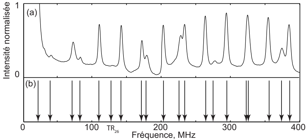
Fig. 3.7 (a), spectre GAWBS dépolarisé dans une HNFL. (b), les flèches marquent les fréquences des modes de résonance, solutions de l'équation 1.18 avec les paramètres suivant \alpha = 0.6248 et V_L = 6050\text{m/s} . La vitesse plus élevée que dans une fibre SMF-28 est due au dopage germanium .
