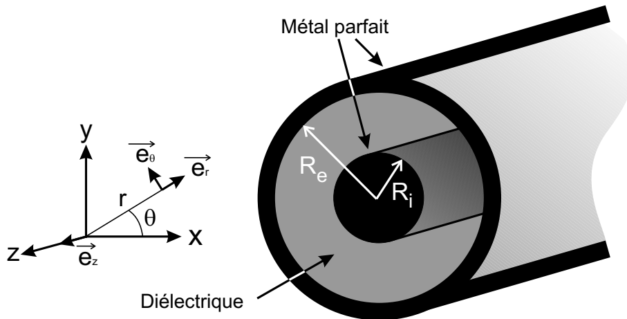
Figure 1.5 – Schéma de la cavité étudiée. Les parois en métal parfait sont séparées par une couche de diélectrique. Un repère en coordonnées cartésiennes et un repère en coordonnées cylindriques orientent l'espace.
