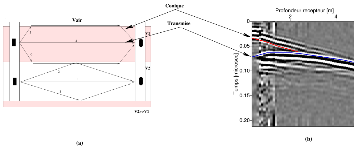
FIG. 3.4 – Trajectoires des ondes EM dans un milieu stratifié et à forts contrastes de vitesse (a) Trajectoires schématiques avec V2 vitesse élevée et V1 vitesse lente : les notations 1 et 4 correspondent à la directe, 2 et 3 à la réfléchie et 5 et 6 à la conique (b) Point de tir du panneau tomographique 5/10 où l'émetteur se situe à 0.3 m de profondeur, en période humide (courbe rouge : conique et courbe bleue : transmise)
