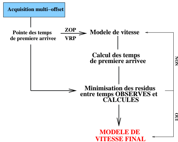
FIG. 4.1 – Méthodologie d'inversion
