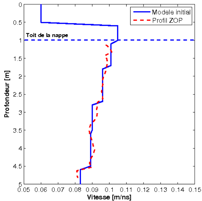
FIG. 5.1 – Détermination du modèle initial à partir des raies ZOP pour le panneau 5/10 en période humide
