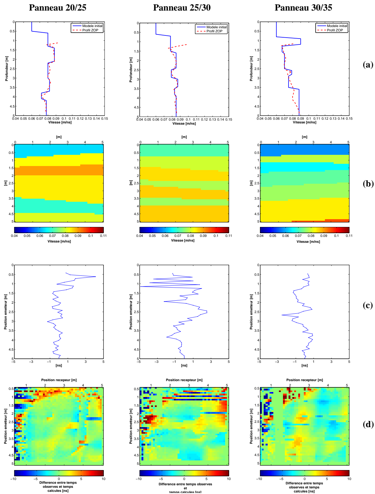
FIG. 5.11 – Résultats obtenus après inversion des panneaux tomographiques 20/25, 25/30 et 30/35 de façon individuelle en période humide
