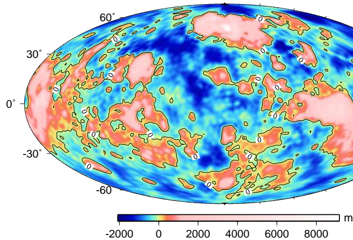
FIG. 2.25 – Topographie de Vénus.
