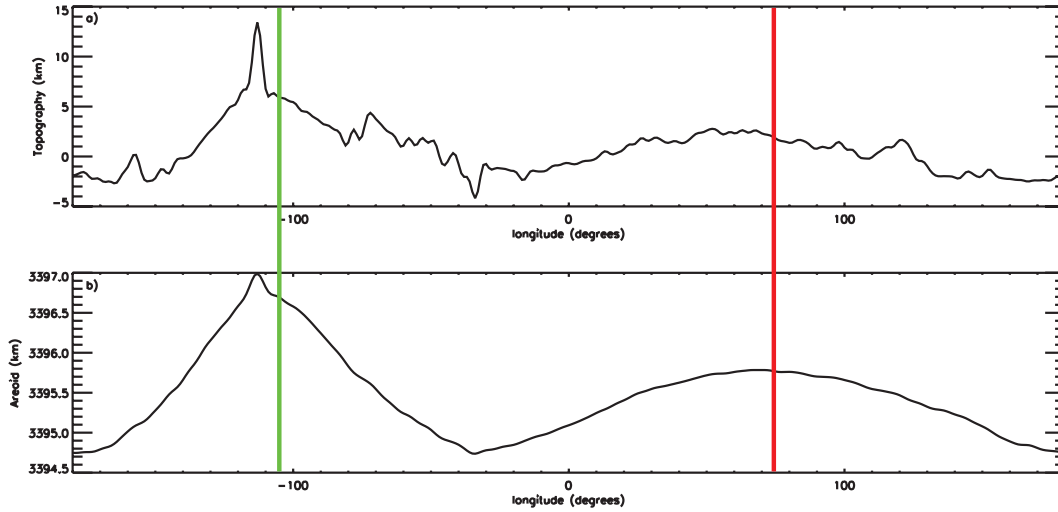
FIG. 2.12 – Profils équatoriaux de la topographie et du géoïde martiens. La ligne rouge indique la longitude du potentiel de pesanteur minimum le long de Deuteronilus ( 75^\circ ).
