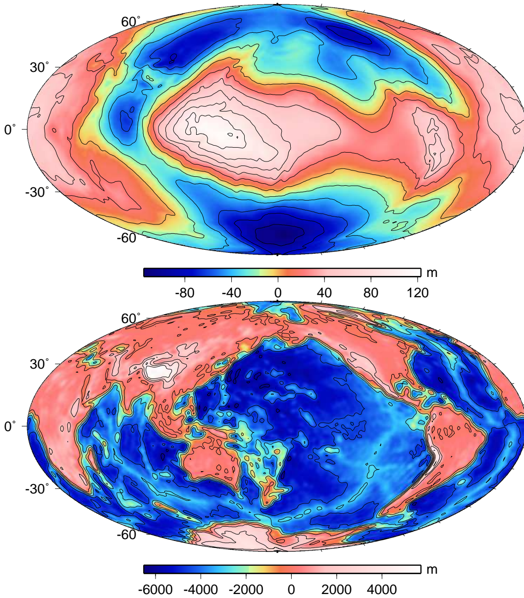
FIG. 1.1 – Géoïde et topographie de la Terre (d'après Wiczorek (2007)).
