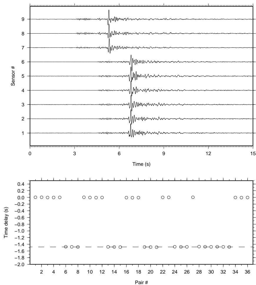
FIG. 4.2 – En haut : traces du séisme tectonique du 6 janvier 2004, de magnitude M_L = 1.22 , enregistré sur les 9 capteurs de l’antenne d’Argentière. En bas : différences de temps d’arrivée calculées pour tous les couples possibles. Ces derniers sont classés dans l’ordre suivant : 1-2, 1-3, ..., 1-9, 2-3, ..., 2-9, ..., 8-9. Seuls les couples faisant intervenir les stations ARG1 ou ARG2 et ARG3 présentent une différence de temps d’arrivée de -1,48 s.
