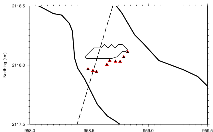
FIG. 4.14 – Représentation schématique de la zone dans laquelle la source de bruit nocturne est susceptible de se trouver.
