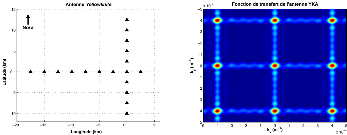
FIG. 2.2 – à gauche : géométrie de l’antenne Yellowknife ( YKA ), située au Canada. La distance entre les capteurs est de \Delta x = 2500m . à droite : fonction de transfert dans le plan des nombres d’ondes (k_x, k_y) . Le nombre d’onde maximal caractérisable avec YKA est de \frac{1}{2\Delta x} , qui correspond à la demi-distance entre le lobe principal (centré sur (0, 0) ) et les lobes secondaires.
