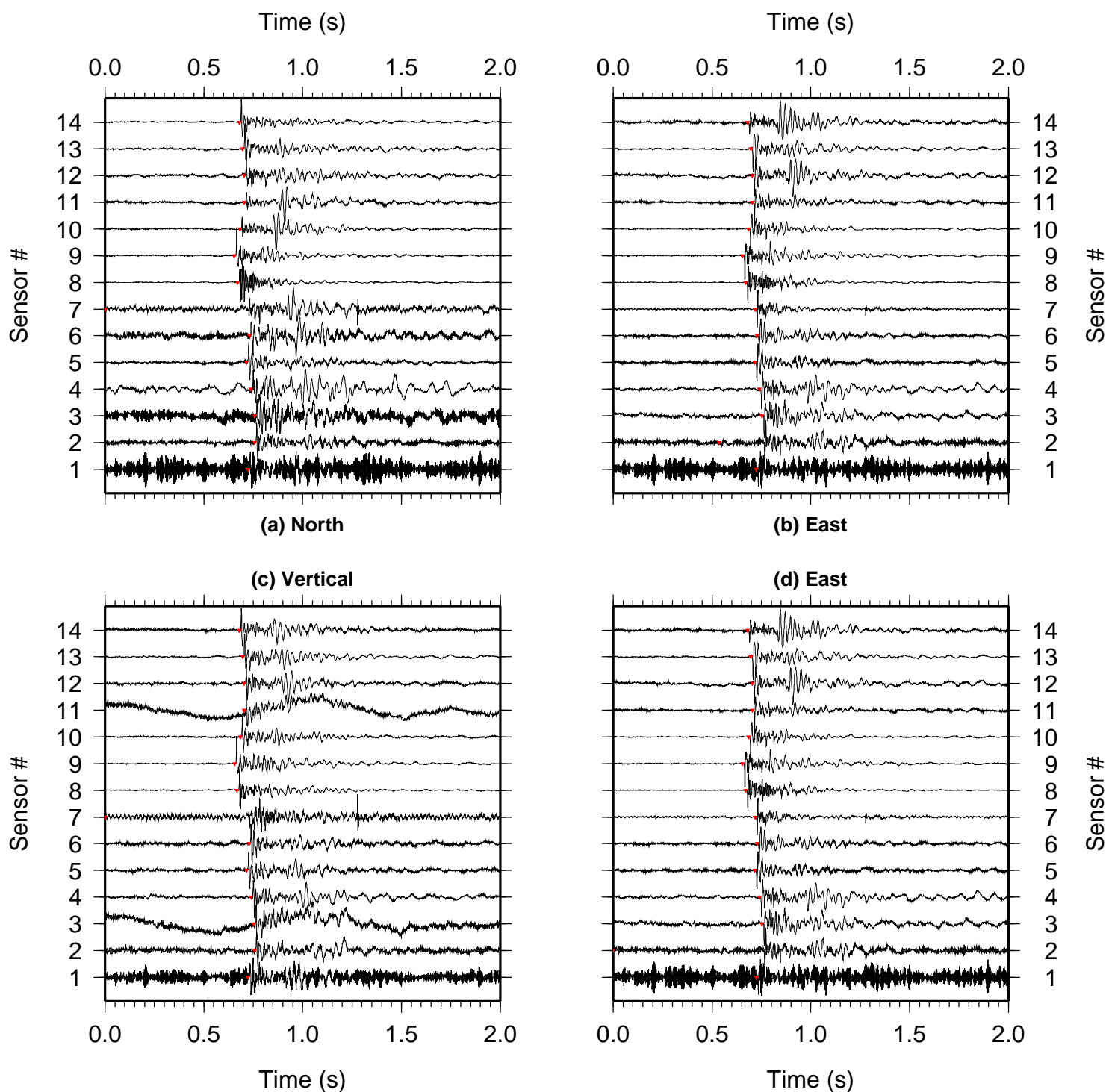
FIG. 5.6 – Exemple d'application du critère de pointé de phase utilisant l'algorithme de Earle and Shearer (1994) au séisme de la figure 5.5. Les paramètres de pointé sont les suivants : STA 0.01s , LTA 0.2s , seuil à 5 et seuil de corrélation à 85 %. (a), (b) et (c) : pointés réalisés sur les composantes Est, Nord et Verticale, respectivement, après la première étape du critère. La voie #7 des composantes Verticale et Nord sont à zéro, indiquant que le pointé n'a pas fonctionné avec les paramètres utilisés. On remarque de plus que le pointé de la voie # 2 de la composante Est ne correspond pas à la première arrivée. Le résultat final pour la composante Est est montré en (d). Le pointé de la voie # 2 a effectivement été mis à 0.
