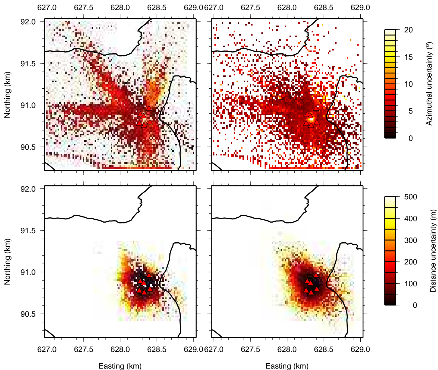
FIG. 6.11 – Répartition spatiale de l'incertitude (intervalles de confiance à 90%) en distance (en bas) et en azimuth (en haut), pour les deux périodes de temps considérées. Dans les deux cas, les échelles de couleur sont saturées (ne sont représentées que des incertitudes inférieures à 500 m et 20°, respectivement). On constate que, pour la seconde période (après le début de la vidange), le périmètre à l'intérieur duquel l'incertitude reste inférieure à 500 m augmente sensiblement. Aucun critère sur l'amplitude crête-à-crête n'est appliqué.
