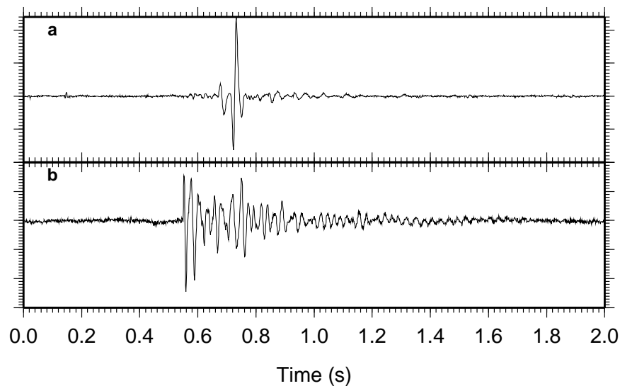
FIG. 5.3 – Comparaison entre un séisme glaciaire de surface ( a ) (17/06/04, 11h33) et un séisme glaciaire profond ( b ) (20/06/04, 1h10). Le rapport d’amplitude entre l’onde P et l’onde de Rayleigh est nettement supérieur dans le cas du séisme profond.
