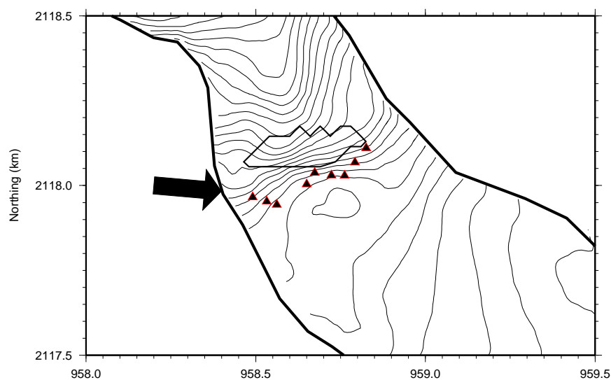
FIG. 4.11 – Représentation schématique de la direction de propagation (direction source – capteur) indiquée par l’asymétrie des fonctions de corrélation.
