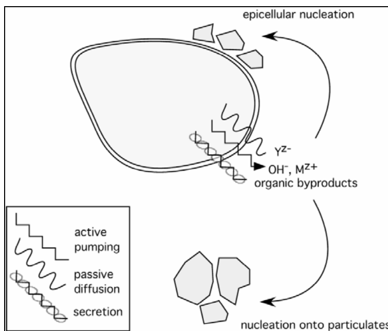
Figure 10: Illustration de la minéralisation biologiquement induite. Le minéral précipite de manière fortuite selon les activités métaboliques de l'organisme qui affectent le pH, pCO_2 et la production de sécrétions. La cellule est uniquement un germe responsable sans aucun contrôle sur le type ou la structure du minéral formé.
