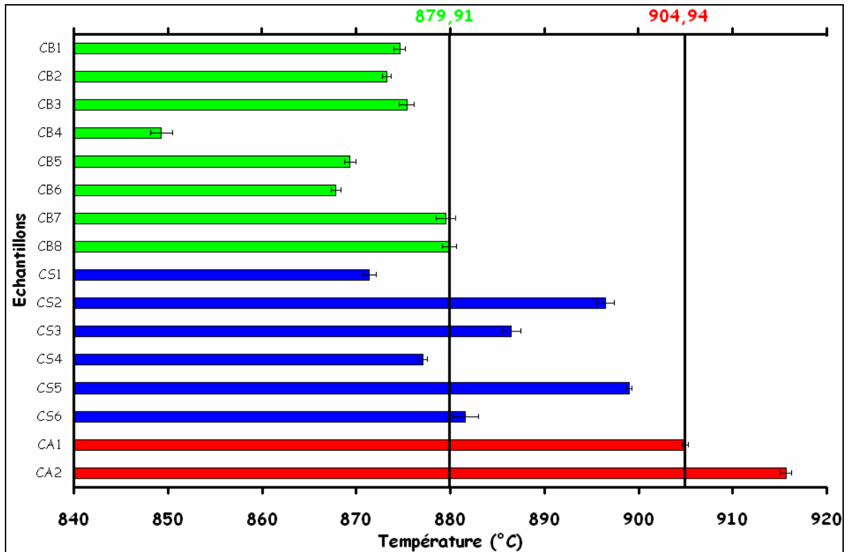
Figure 9 : Comparaison des températures de l'absorption maximale d'énergie T_D de chaque échantillon. L'ordonnée représente les échantillons. L'abscisse représente la température moyenne de l'absorption maximale d'énergie T_{Dm} atteinte par chaque échantillon. Une différence de température de 25,03 \pm 2,76 °C sépare les échantillons de calcite biogéniques et les échantillons de calcite abiotiques. Entre les deux se trouvent la plupart des échantillons de calcite sédimentaires dont la minéralogie a évolué suite à de la diagenèse. Les températures des points d'inflexion délimitant le domaine biologique à gauche et le domaine abiotique à droite sont respectivement celles des échantillons CB8 et CA1 dont les valeurs sont 879,91 \pm 0,72 °C et 904,94 \pm 0,34 °C
