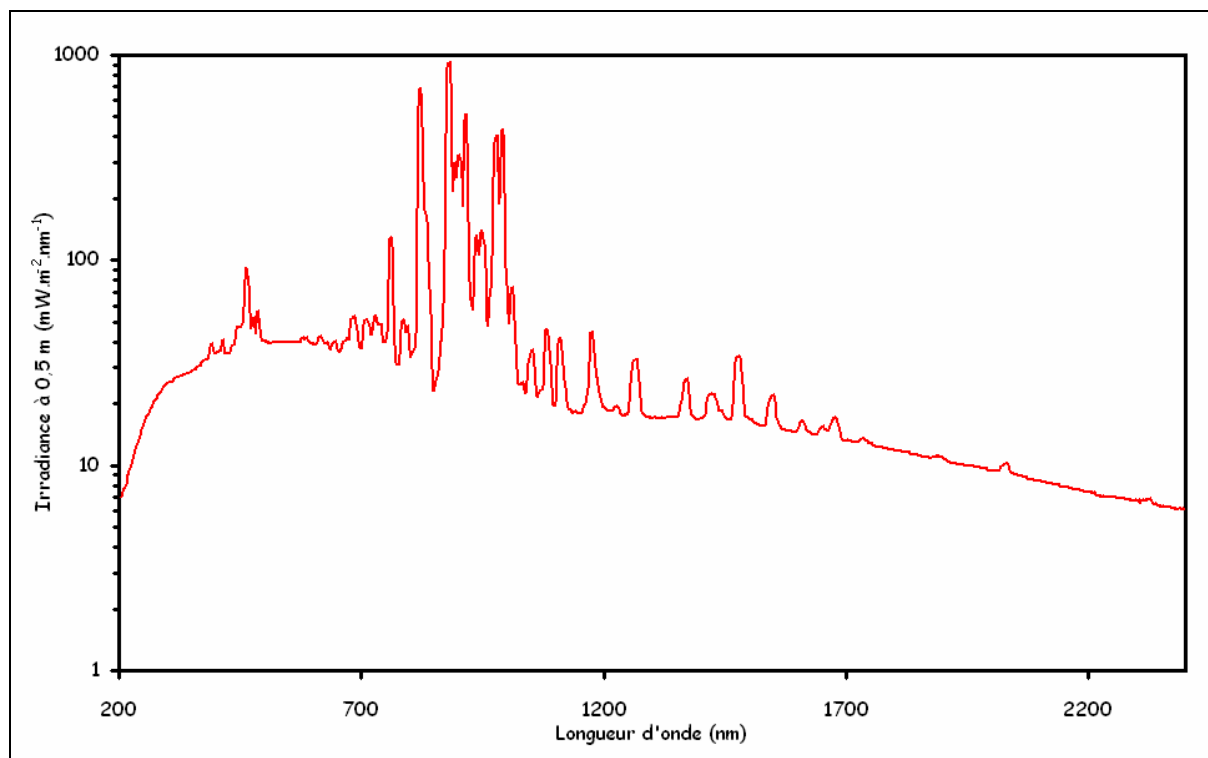
Figure 5 : Spectre d'irradiance exprimée en mW/m^2/nm , en fonction de la longueur d'onde (exprimée en nm ) de la source d'irradiation utilisée dans la chambre MOMIE. Source : données constructeurs LOT-ORIEL.
