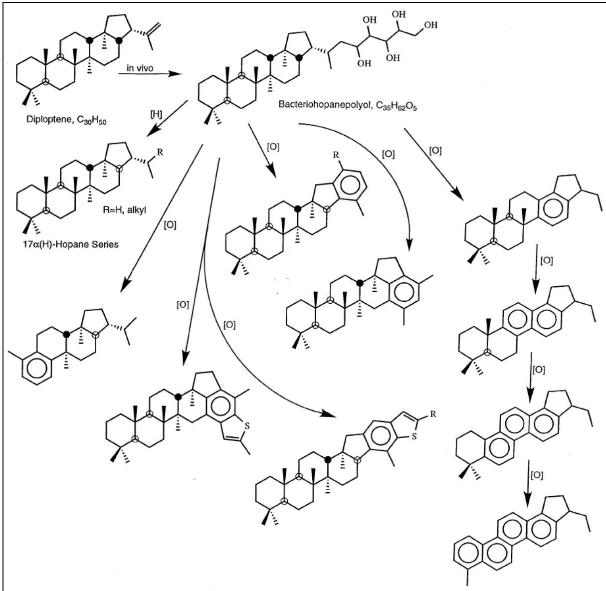
Figure 16 : Schéma d'altération des hopanoïdes : [H] par réduction (ou catagénèse) et [O] par oxydation des fonctions aromatiques ou par réaction avec du soufre pour produire des hétérocycles soufrés. Les composés de départ dans ce schéma sont le diploptène et le bacteriohopanepolyol. Plus le degré d'oxydation est élevé (selon la voie [O], à droite), plus la formation de noyau benzénique est grande, plus le composé est stable dans les conditions environnementales terrestres sur de longues périodes géologiques. La catagenèse par réduction [H] produit également des composés très résistants : les hopanes. Sources : (Simoneit et al., 1998; Simoneit, 2004)
