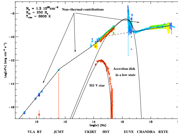
FIG. 2.5 – Distribution spectrale d'énergie du microquasar XTE J1118+480, qui peut être décrite par la somme des émissions du disque d'accrétion à corps noir multicolore, une contribution non-thermique du jet, et l'émission thermique de l'étoile compagnon M1 V (Chaty et al., 2003b).
