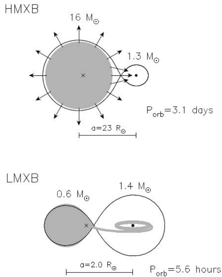
FIG. 1.2 – Systèmes binaires de grande masse et de faible masse : schémas typiques de HMXB (en haut) et LMXB (en bas). L'étoile à neutron dans une HMXB accrete un fort vent stellaire de grande vitesse et/ou l'atmosphère de l'étoile commençant à dépasser le lobe de Roche. L'étoile à neutron dans une LMXB est entourée d'un disque d'accrétion qui est alimenté par dépassement du lobe de Roche. Il existe aussi des évidences observationnelles que certaines HMXBs et LMXBs contiennent des trous noirs. Figure tirée de Tauris & van den Heuvel (2006).
