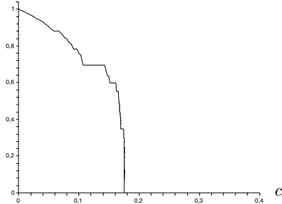
\dim_H F(c, 2)
