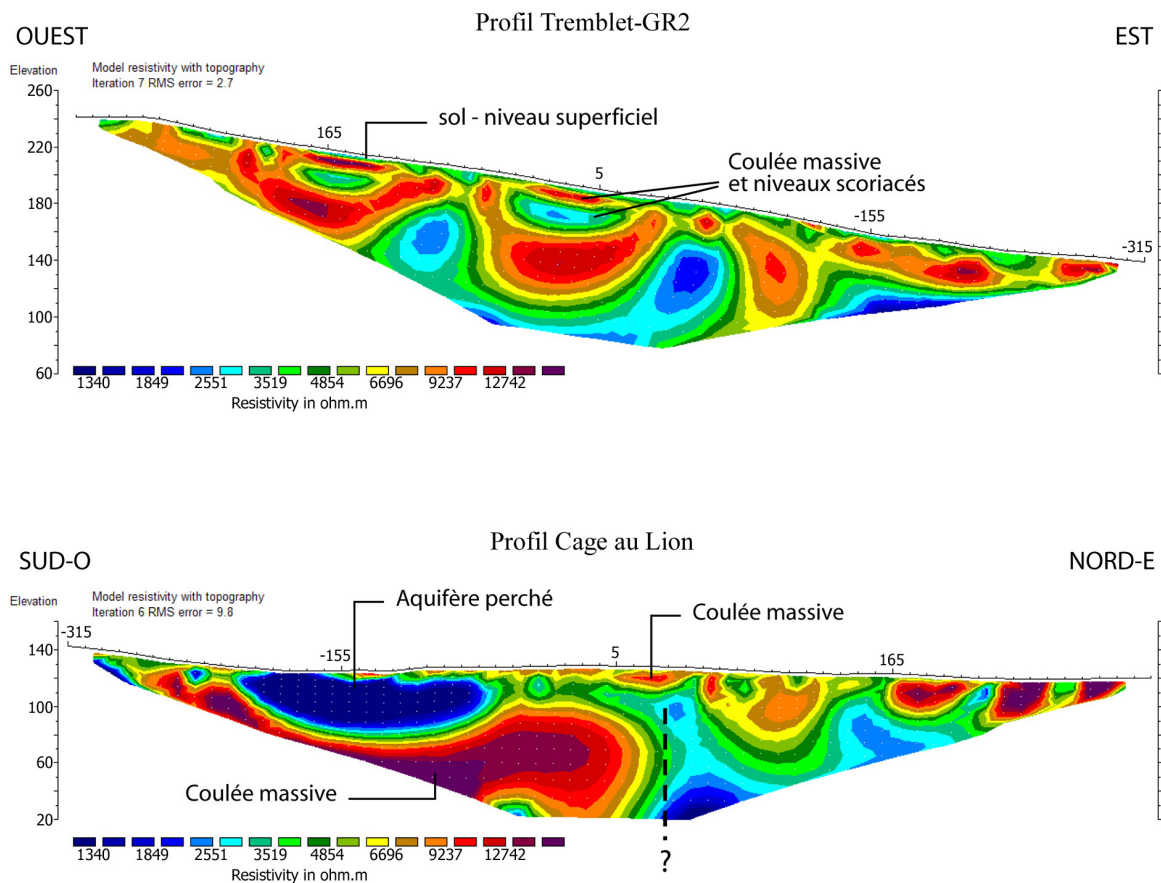
Figure III-48 : Modèles de résistivité pour les profils réalisés en dehors du Grand Brûlé, au sud du Rempart du Tremblet (Tremblet-GR2 ; erreur RMS de 2,7 après 7 itérations) et au nord du Rempart de Bois Blanc (Cage au lion ; erreur RMS de 9,8 après 6 itérations).
