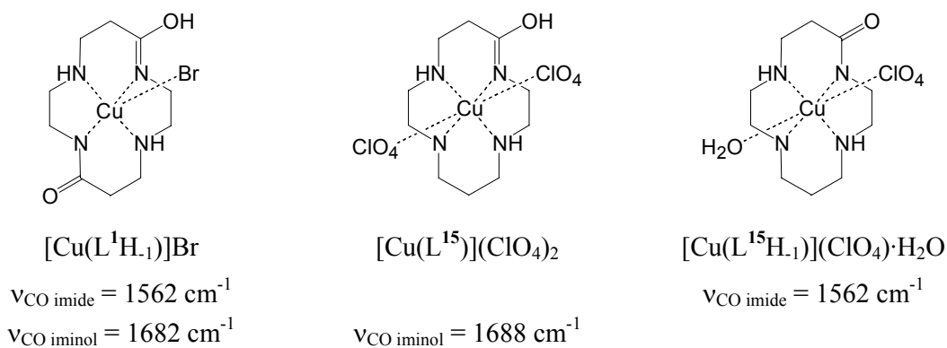
Figure II-27. Données infrarouge relatives aux complexes de cuivre des ligands L^1 et L^{15} [91].
