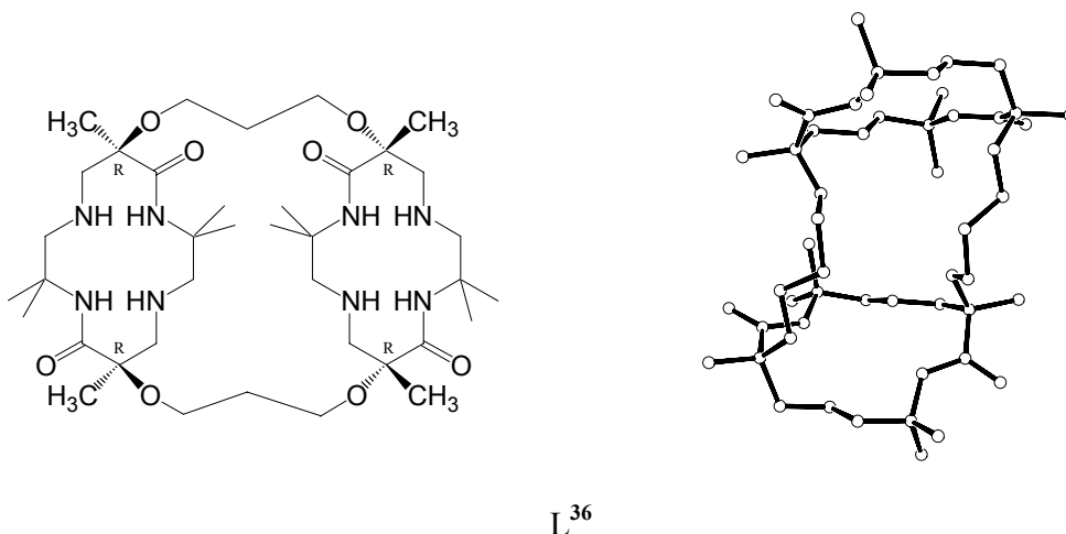
Figure I-15. Formule chimique et structure cristallographique du diastéréoisomère d,l-d,l (ou R,R-R,R ) du bisdioxocyclame L^{36} préparé selon la méthode d'Hegedus [165].
