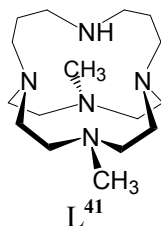
Figure I-21. Formules chimiques de polyaza- et polyoxamacrobicycles.
