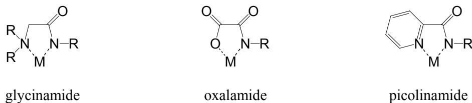
Figure I-1. Cycles chélates dans lesquels l'amide est coordonné au métal via l'atome d'azote.
