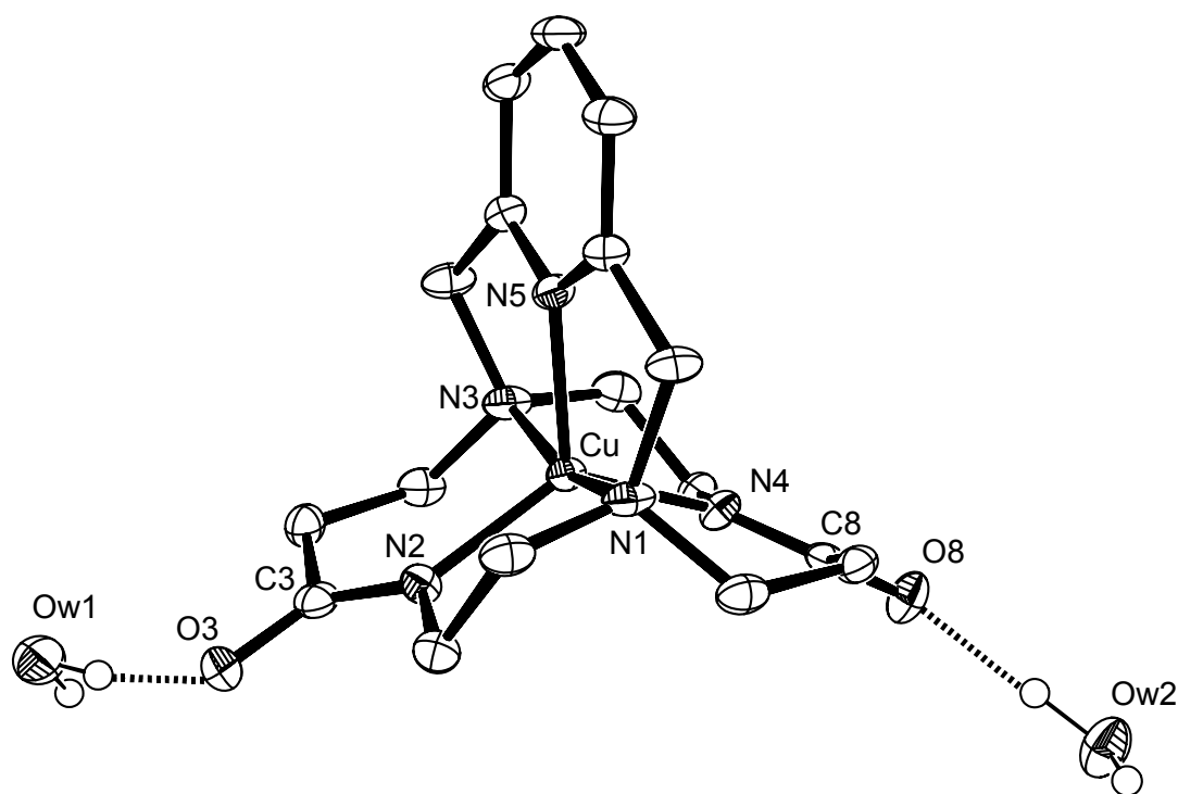
Figure III-28. Vue ORTEP du [\text{Cu}(\text{L}^6\text{H}_2)]^0 . Les ellipsoïdes sont représentés au seuil de probabilité de 50 %.
