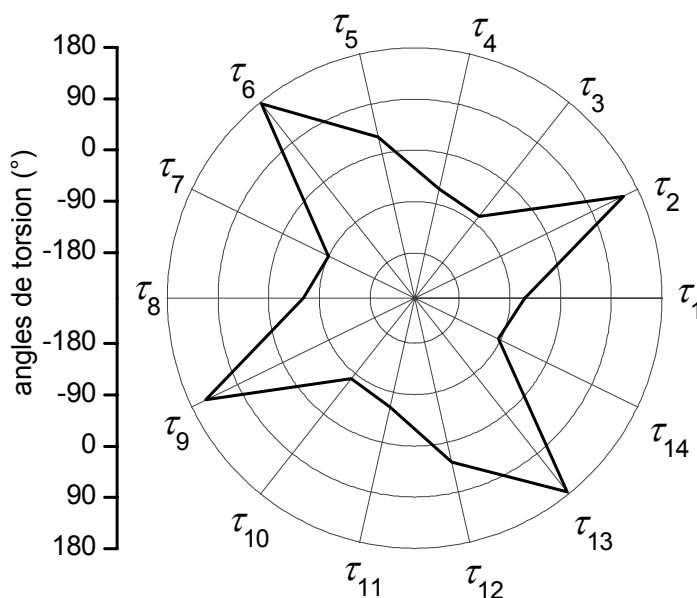
Figure II-10. Diagramme polaire présentant les angles de torsion des deux sous-unités macrocycliques du ligand L 3 . \tau_1 correspond à l'angle de torsion N3-C5-C4-N2, les angles suivants sont obtenus par permutation circulaire dans le sens des aiguilles d'une montre.
