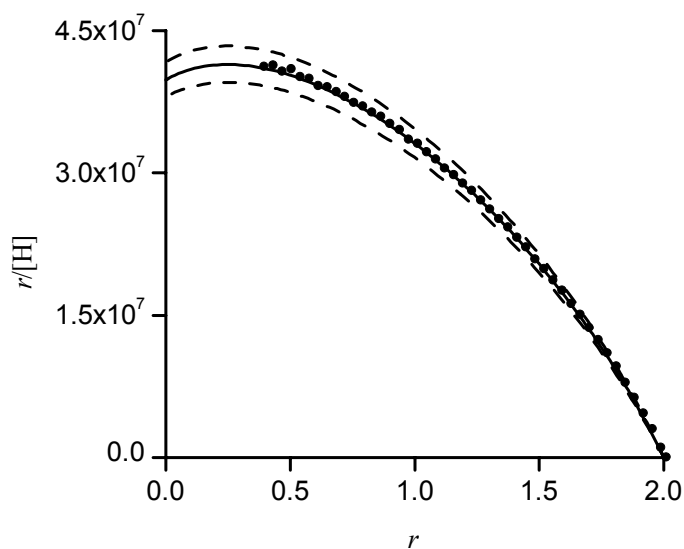
Figure II-14. Courbes de Scatchard correspondant à la protonation du ligand L^1 : données expérimentales ( \bullet ) et calculées pour \log K_{011} = 7,60 et \log K_{012} = 7,44 (—) ; \log K_{011} = 7,60 \pm 0,02 et \log K_{012} = 7,44 \pm 0,02 (---).
