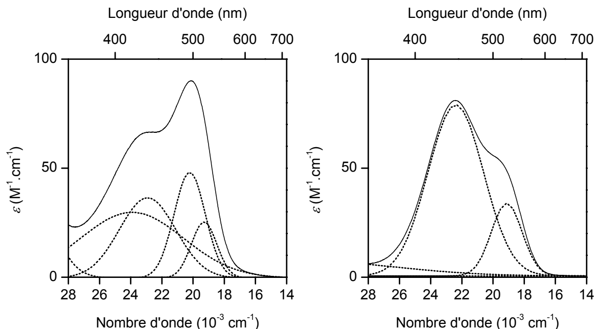
Figure II-19. Spectres électroniques des complexes [Ni(L^1H_2)]^0 \cdot H_2O (gauche) et [Ni(L^2H_2)]^0 \cdot 2H_2O (droite) en solution aqueuse.
