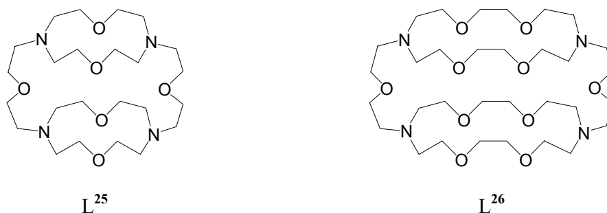
Figure I-11. Formules chimiques de ligands macrotricycliques cylindriques [142,144].
