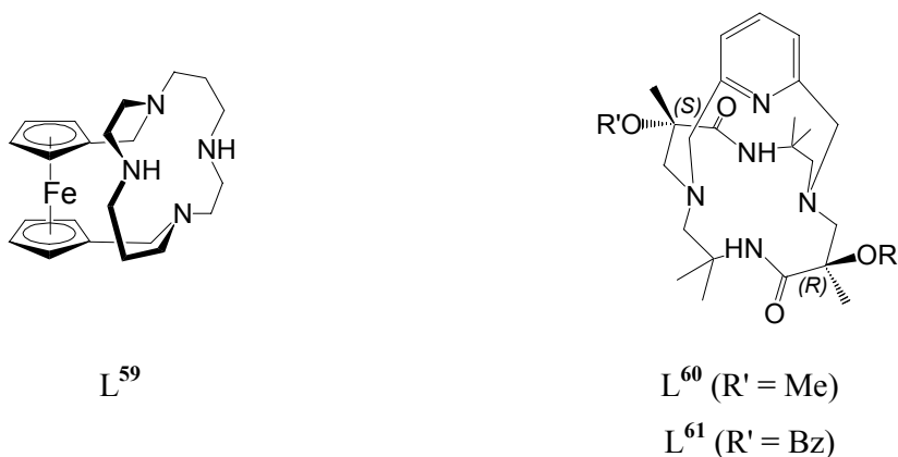
Figure I-27. Formules chimiques de macrobicycles.
