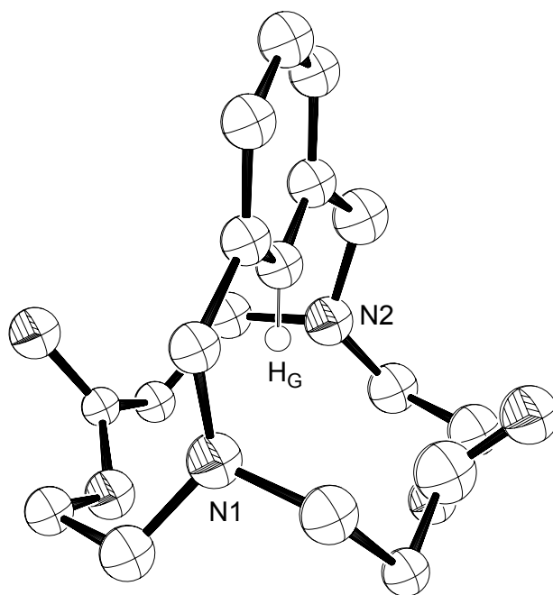
Figure III-14. Affinement isotrope de la structure cristallographique du ligand L 5 (conformère A). Le proton du groupe xyle a été introduit en position calculée.
