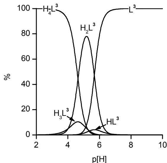
Figure II-13. Courbe de distribution des espèces libres et protonées du ligand L^3 dans le mélange eau-méthanol (50/50 v/v). [L^3]_{\text{tot}} = 2 \times 10^{-3} \text{ M} ; I = 0,1 \text{ M} (KCl) ; T = 25 \text{ }^\circ\text{C} .
