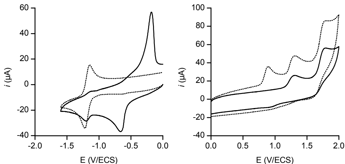
Figure III-34. Voltammétrie cyclique sur électrode de carbone vitreux des complexes [\text{Cu}(\text{L}^6\text{H}_1)]\text{ClO}_4 \cdot \text{H}_2\text{O} (—) et [\text{Cu}(\text{L}^6\text{H}_2)]^0 \cdot 4\text{H}_2\text{O} (- - -). Solvant : MeCN ; [\text{CuL}^6] = 1 \times 10^{-3} \text{ M} ; I = 0,1 \text{ M} (TBAP) ; \nu = 100 \text{ mV/s} .
