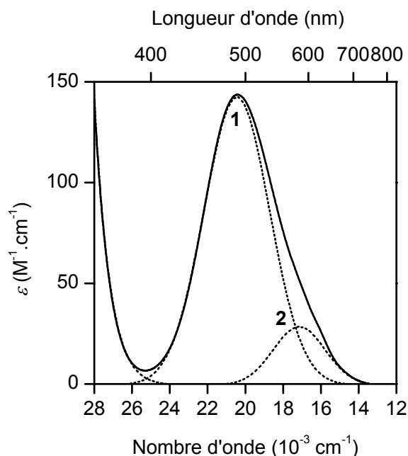
Figure II-43. Déconvolution du spectre électronique du complexe mononucléaire [\text{Cu}(\text{L}^3\text{H}_2)]^0 \cdot 3\text{H}_2\text{O} en solution aqueuse.
