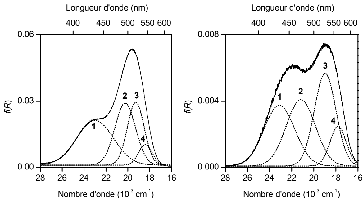
Figure II-18. Déconvolution des spectres électroniques des complexes [\text{Ni}(\text{L}^1\text{H}_2)]^0 \cdot \text{H}_2\text{O} (gauche) et [\text{Ni}(\text{L}^2\text{H}_2)]^0 \cdot 2\text{H}_2\text{O} (droite) à l'état solide.
