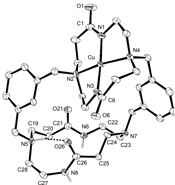
Figure II-40. Vue ORTEP d'un des deux stéréoisomères trouvé dans la structure cristallographique de [Cu(L 3 H 2 )H]ClO 4 ·8,5H 2 O. Les ellipsoïdes sont représentés au seuil de probabilité de 50 %.
