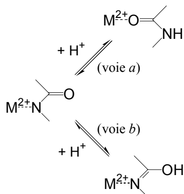
Figure I-4. Protonation d'une liaison métal-amide.
