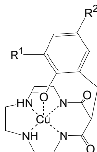
Figure I-9. Formule chimique du complexe [\text{Cu}(\text{L}^{24}\text{H}_3)]^+ avec \text{R}^1 = \text{R}^2 = \text{H} ou Br.
