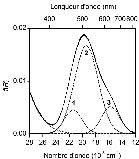
Figure II-42. Déconvolution du spectre électronique de [\text{Cu}(\text{L}^3\text{H}_2)]^0 \cdot 3\text{H}_2\text{O} à l'état solide.
