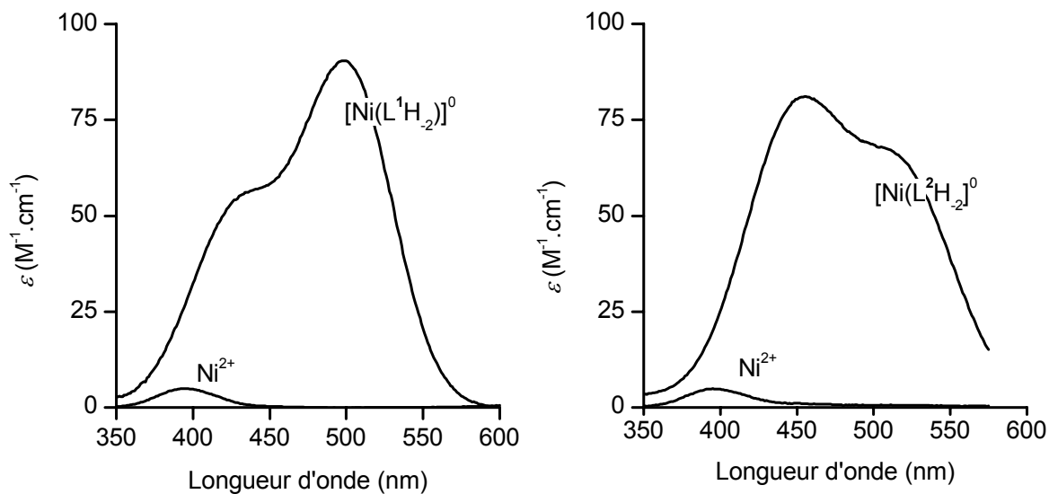
Figure II-22. Spectres électroniques calculés des complexes de nickel(II) formés avec les ligands \text{L}^1 et \text{L}^2 . I = 0,1 \text{ M} ( \text{KNO}_3 ) ; T = 25 \text{ }^\circ\text{C} .
