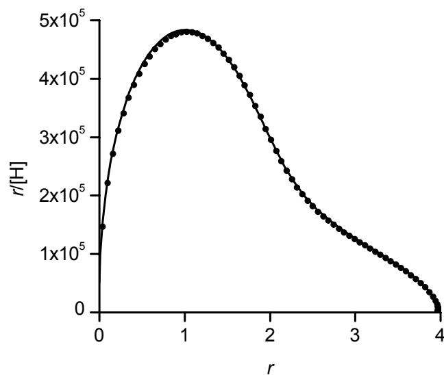
Figure II-15. Courbes de Scatchard correspondant à la protonation du ligand L^3 : données expérimentales (●) et calculées pour \log K_{011} = 4,71 ; \log K_{012} = 6,63 ; \log K_{013} = 4,03 et \log K_{014} = 5,24 (—).
