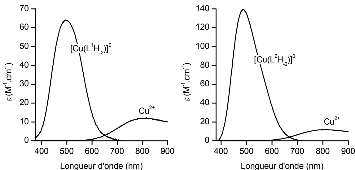
Figure II-39. Spectres électroniques calculés des complexes de cuivre(II) des ligands L^1 et L^2 . I = 0,1 \text{ M (KNO}_3) ; T = 25 \text{ }^\circ\text{C} .
