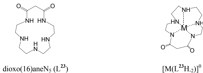
Figure I-8. Formules chimiques du cis -dioxopentaazamacrocycle L 23 et du complexe [M(L 23 H 2 )] 0 (M = Ni 2+ ou Cu 2+ ).
