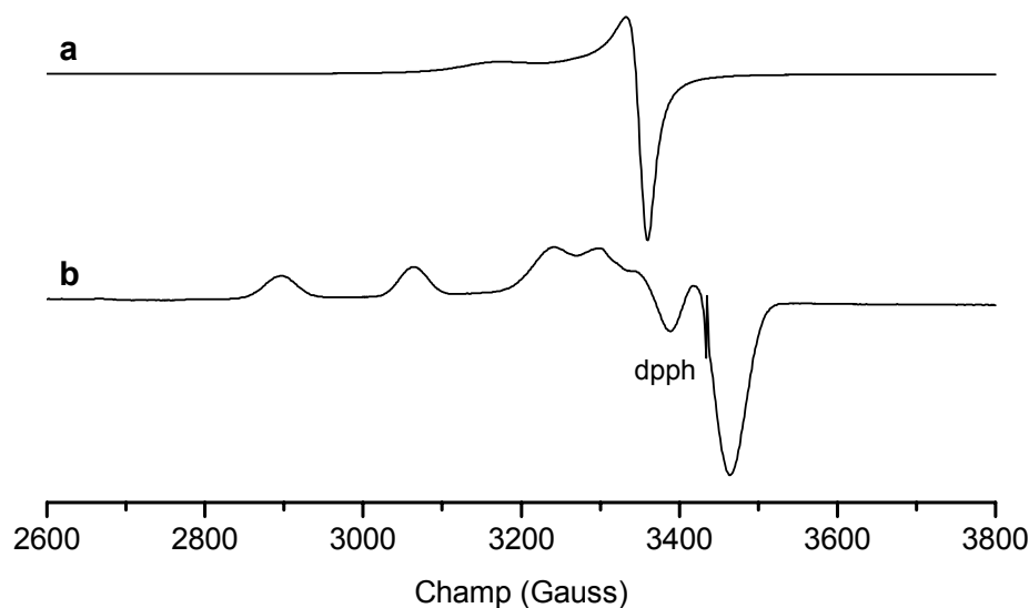
Figure IV-4. Spectre RPE bande X du complexe [\text{Cu}(\text{L}^7)](\text{ClO}_4)_2 \cdot \text{H}_2\text{O} à l'état solide (a) et en solution gelée (b). Solide : \text{MgSO}_4 ; T = 100 K. Solution : mélange eau-éthylène glycol (7/3 v/v) ; T = 100 K.
