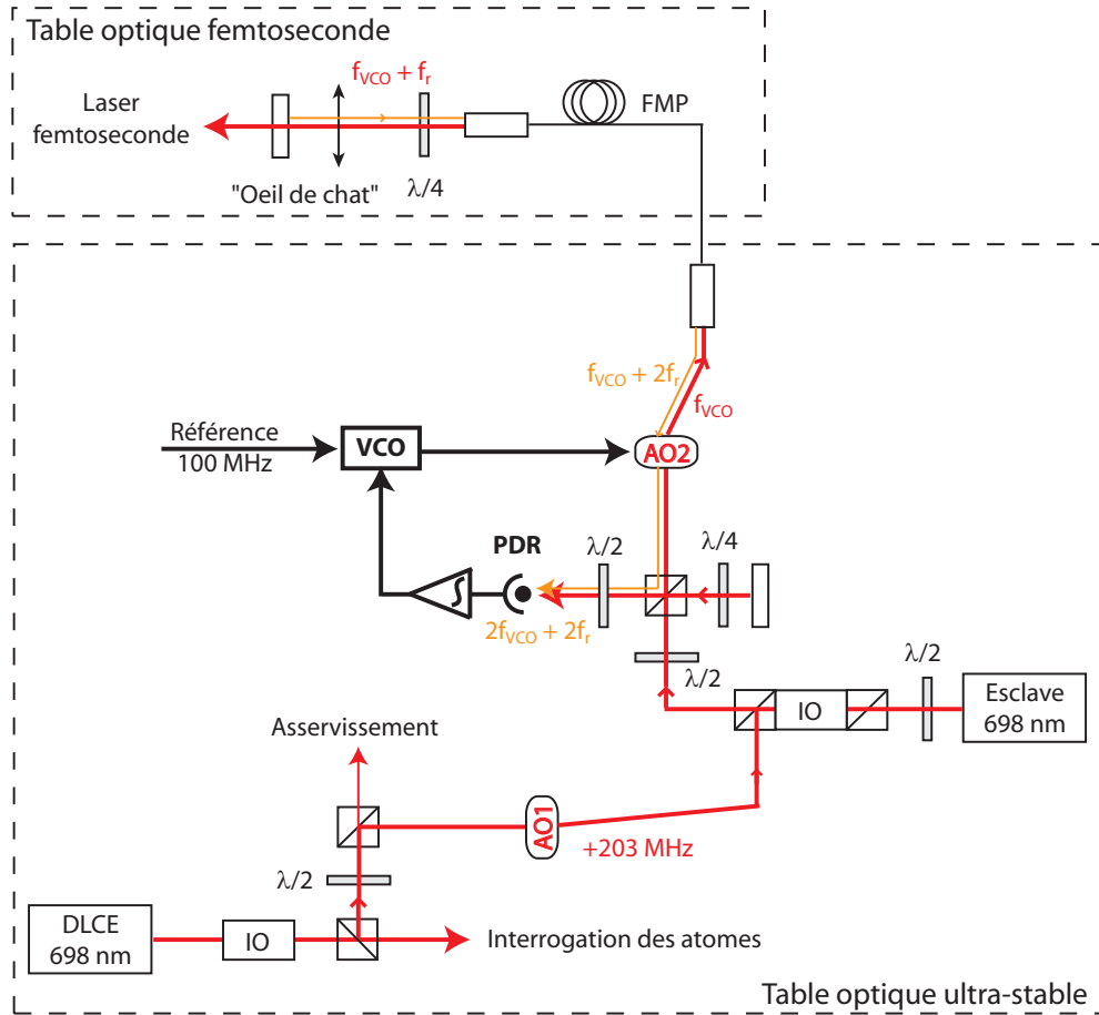
FIG. 3.9 – Dispositif d’annulation du bruit de phase. DLCE : diode laser à cavité étendue ; IO : isolateur optique ; PDR : photodiode rapide ; VCO : voltage controlled oscillator.
