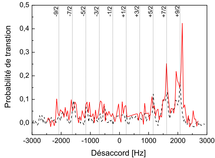
FIG. 5.10 – Spectre des différentes transitions \pi lorsque les atomes sont interrogés en présence d'un champ magnétique de 4.2 G et après une phase de pompage optique avec un laser polarisé \sigma^+ . Courbe noire (tirets) : avant optimisation du pompage optique. Courbe rouge (traits pleins) : après optimisation. On voit que les atomes se trouvent essentiellement dans les deux derniers niveaux. Les traits pointillés verticaux représentent les fréquences théoriques des différentes résonances pour un champ magnétique de 4.2 G.
