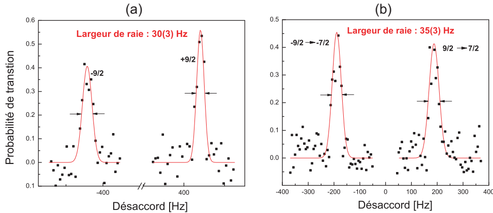
FIG. 5.13 – Résonances utilisées pour asservir le laser d’horloge sur la transition atomique. (a) Résonance m_F = 9/2 \rightarrow m_F = 9/2 et symétrique. (b) Résonance m_F = 9/2 \rightarrow m_F = 7/2 et symétrique. Dans les deux cas la largeur de raie est de l’ordre de 30 Hz. Les dissymétries proviennent d’une efficacité différente du pompage optique dans les deux sens.
