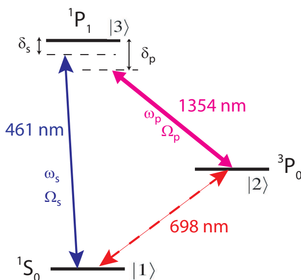
FIG. 6.1 – Schéma des niveaux intervenant dans l'excitation de la transition ^1S_0 \rightarrow ^3P_0 du ^{88}\text{Sr} en utilisant deux lasers et le niveau ^1P_1 comme intermédiaire.
