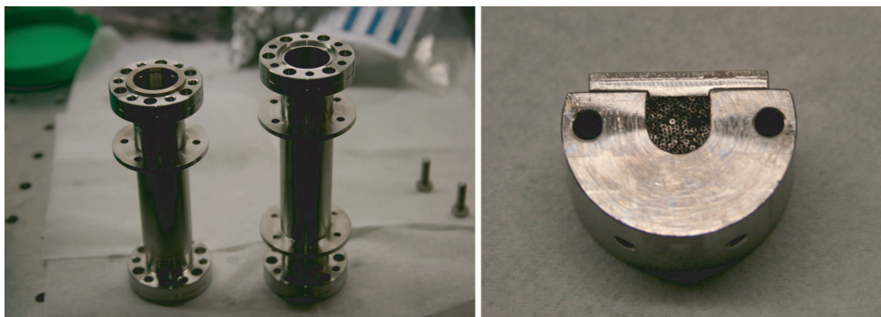
FIG. 4.2 – Détail des éléments du four. Gauche : tubes CF 16 pour la réserve et les éjecteurs. Droite : support en U et éjecteurs.
