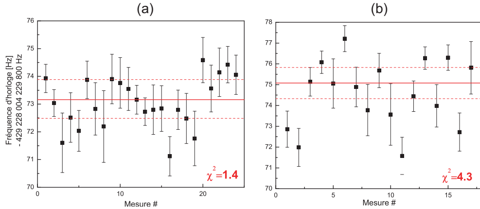
FIG. 5.19 – Séries de mesures répétées un grand nombre de fois dans la même configuration au cours de la campagne de mesure de novembre 2006. (a) B = 0.87 \text{ G} , f_{mod} = 10 \text{ Hz} . (b) B = 1.4 \text{ G} , f_{mod} = 7 \text{ Hz} . Le trait plein central représente la valeur moyenne, et les deux lignes pointillées la barre d'erreur statistique attribuée à chaque série. La valeur \chi^2 indiquée en bas à droite de chaque mesure représente une évaluation de la cohérence statistique de chaque mesure.
