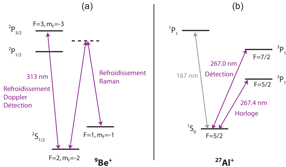
FIG. 1.4 – Niveaux d'énergie utilisés dans la réalisation de l'horloge à ion piégé \text{Al}^+ . (a) Transitions utilisées dans la manipulation de l'ion logique {}^9\text{Be}^+ . (b) Transitions utilisées dans la manipulation de l'ion de spectroscopie {}^{27}\text{Al}^+ .
