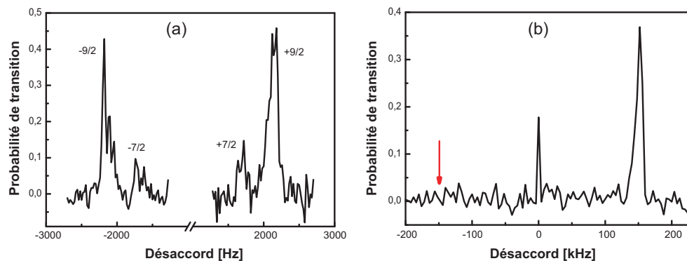
FIG. 5.11 – (a) Spectre de la transition ^1S_0 \rightarrow ^3P_0 en présence d'un champ magnétique B = 4.2 G. Les deux moitiés ont été mesurées séparément en optimisant successivement le pompage optique dans un sens et dans l'autre. (b) Spectre de bandes latérales obtenu avec les mêmes réglages. La flèche rouge indique l'emplacement de la bande latérale rouge.
