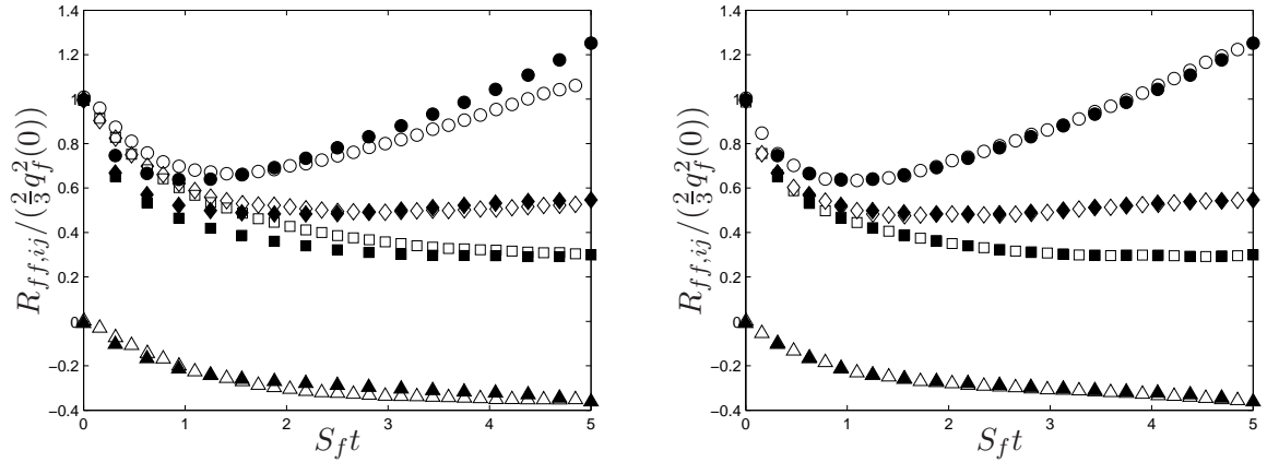
FIG. 5.4 – Développements des contraintes cinétiques du fluide vu par les particules (cas A). gauche : modèle NCSLM avec correction (5.8), droite : modèle NCSLM avec correction (5.9). ○ : lagrangien stochastique (○ : R_{ff,uu} , □ : R_{ff,vv} , ◇ : R_{ff,ww} , △ : R_{ff,uw} ) ; ● : LES/DPS (Laviéville [1997]).
