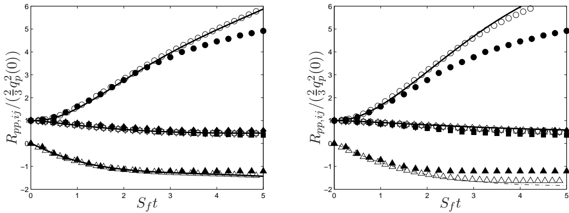
FIG. 5.8 – Développements des contraintes particulaires (cas A) prédits par le modèle SLM (gauche) et le modèle LIPM (droite). \circ : lagrangien stochastique ( \circ : R_{pp,uu} , \square : R_{pp,vv} , \diamond : R_{pp,ww} , \triangle : R_{pp,uv} ); — : eulérien ; \bullet : LES/DPS (Laviéville [1997]).
