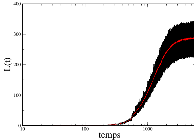
FIG. 2.12 – Fonction de localisation en fonction du temps pour le modèle de l'agrégat (noir). Un lissage est effectué sur \Delta t = 100 unités de temps (rouge).
