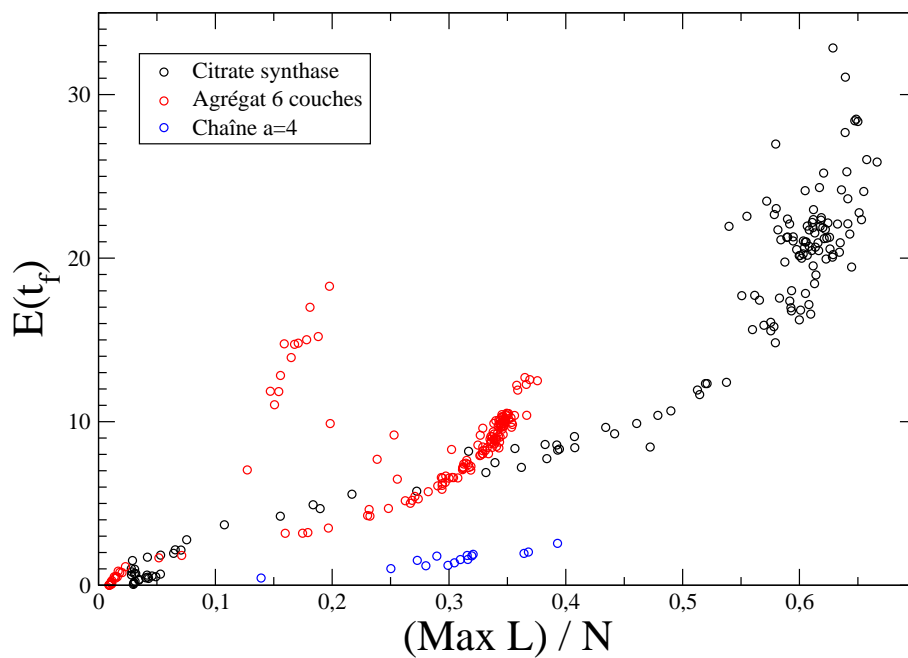
FIG. 3.20 – Energie des différents systèmes à la fin de la simulation ( t = t_f ) en fonction de la valeur maximale de la fonction de localisation MaxL . Le temps de simulation est de t_f = 6000 pour l'agrégat (6 couches) et la citrate synthase, et de t_f = 2 * 10^6 pour la chaîne de N atomes dont le pas a est de 4.
