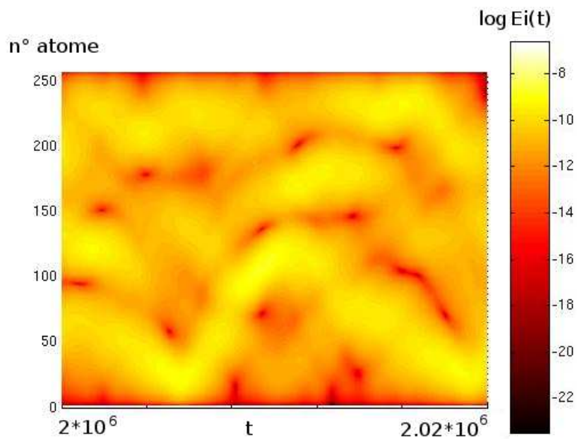
FIG. 1.9 – Energie sur chaque atome dans la chaîne (dynamique A).
