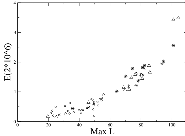
FIG. 1.31 – Energie à t = t_f de la chaîne en fonction de MaxL . La relation entre l'énergie de la chaîne et la localisation est la même pour tous les breathers obtenus. Les distances d'équilibre entre atomes liés sont a=1 ( \circ ), a=2 ( \triangle ) et a=4 ( \star ).
