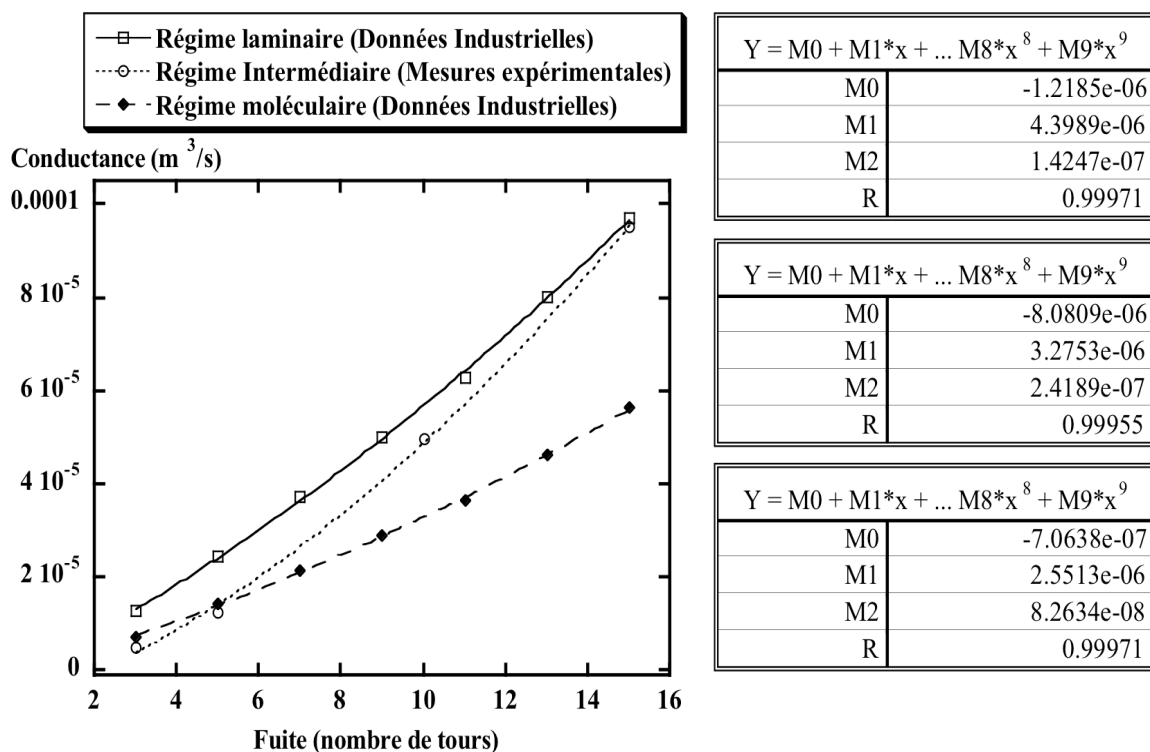
Figure 3.6: Comparaison des conductances, calculées à partir de mesures de débits, et des données industrielles de la vanne de fuite pour N_2 à 300 K. Les courbes ont été ajustées par polynômes respectivement par rapport aux régimes étudiés.
