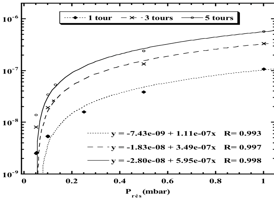
Figure 3.7: Qualification du système d'injection de PIRENEA. Cas de N 2 à 300 K sur une voie VG.
