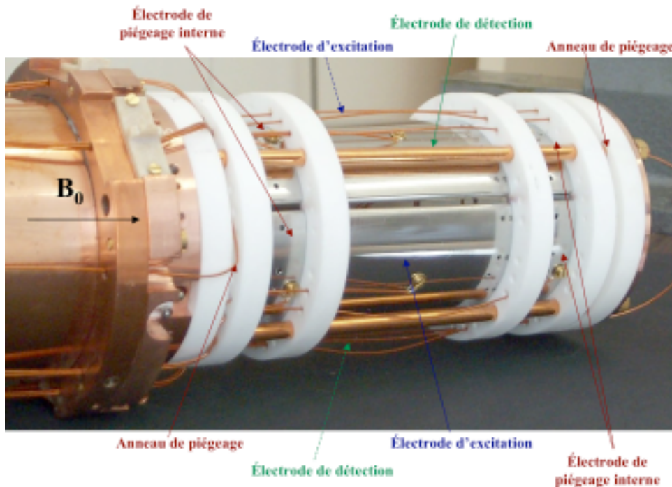
Figure 2.6: Photographie de la cellule ICR de PIRENEA.
