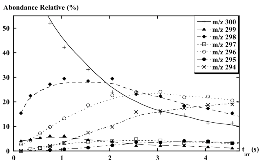
Figure 5.2: Exemple d'une cinétique de photodissociation des espèces 12 C 24 H n + effectuée sous irradiation continue de la lampe à arc Xe dans PIRENEA.
