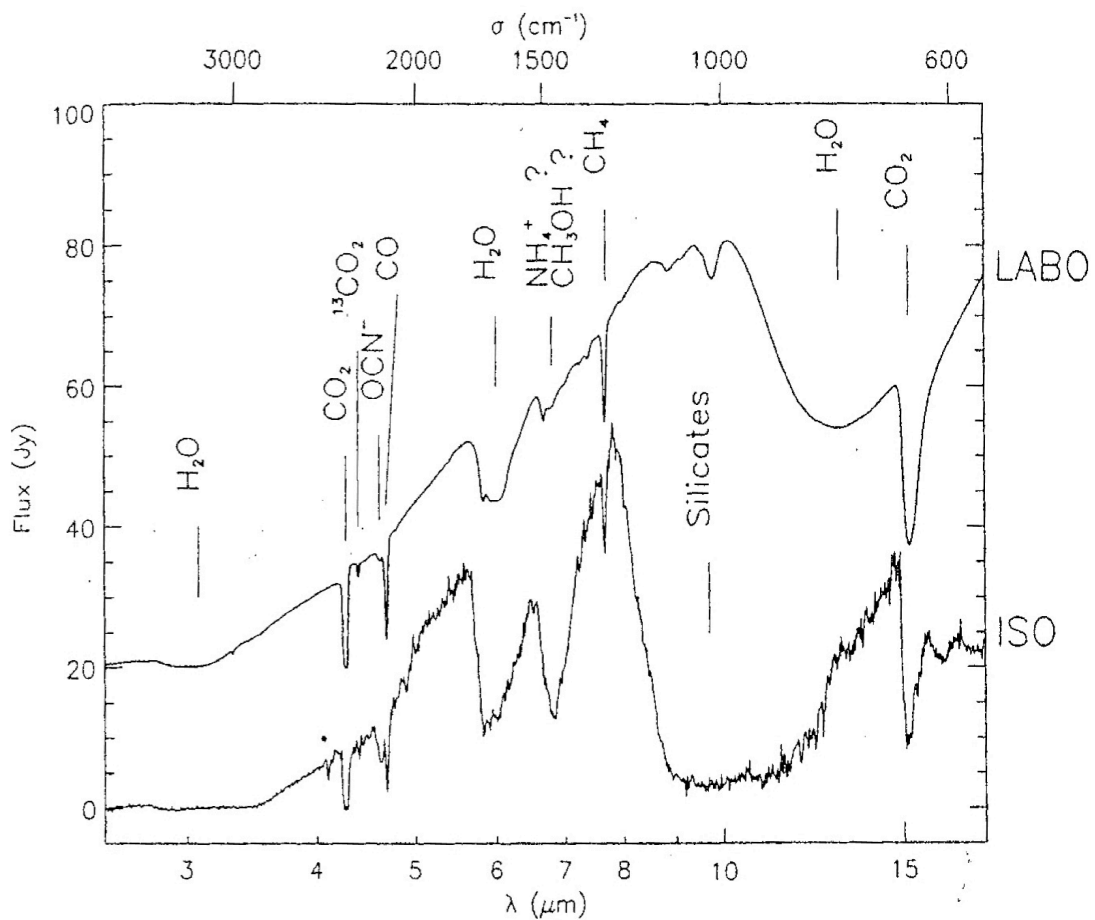
Figure 1.5: Spectre SWS (2.5 - 18 \mu\text{m} ) de la protoétoile RAFGL7009S. Les bandes des glaces moléculaires sont identifiées par des mesures en laboratoire consistant en un dépôt \text{H}_2\text{O}:\text{CO}:\text{CH}_4:\text{NH}_3:\text{O}_2 dans des proportions \sim 10:2:1:1:1 irradié par des photons UV (d'après Dartois 1998).
