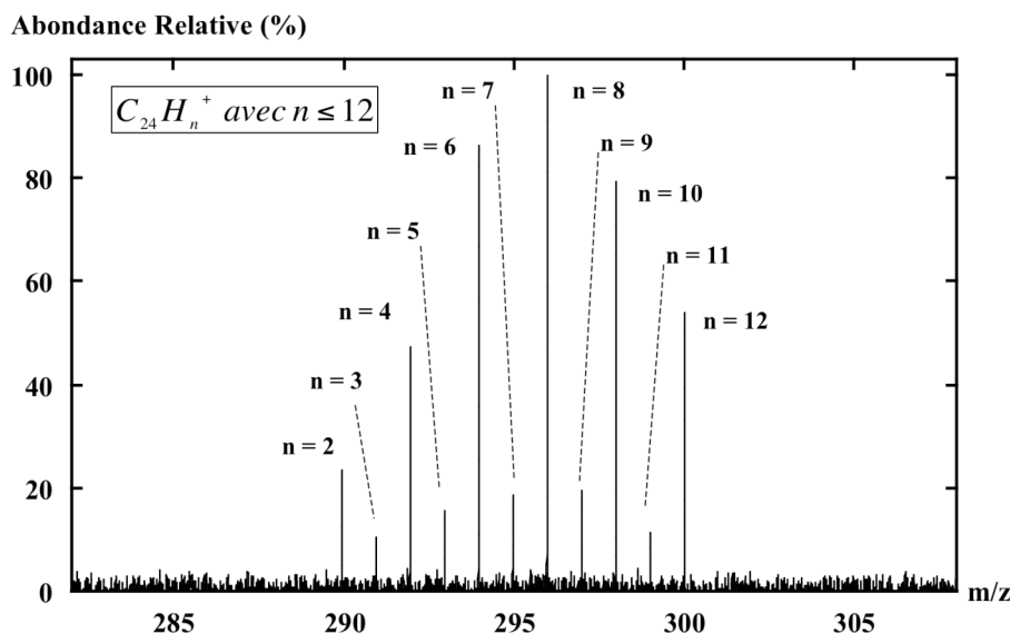
Figure 5.1: Spectre typique de photodissociation de 12 C 24 H 12 + (m/z = 300.094) sous irradiation continue de la lampe à arc Xe ( t_{irr} = 4 s).
