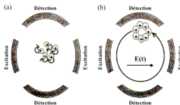
Figure 2.9: Schéma (a) du mouvement cyclotronique incohérent des ions et (b) du mouvement cohérent obtenu par un signal radiofréquence résonnant avec la fréquence cyclotronique effective des ions ( V' ).
