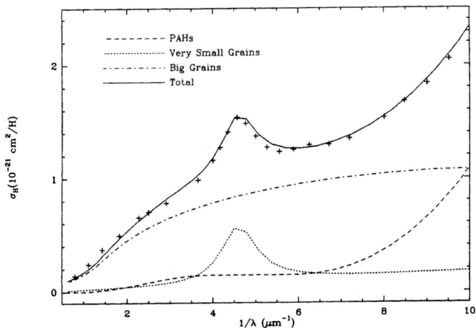
Figure 1.2: Courbe d'extinction du milieu diffus du visible à l'UV avec la contribution des différentes populations de grains: PAH, VSG et BG d'après Désert et al. (1990). Les mesures observationnelles de Savage et Mathis (1979) sont représentées par des croix. L'absorption importante autour de 4,5 \mu\text{m}^{-1} ( 220 \text{ nm} ) est généralement appelée "bump".
