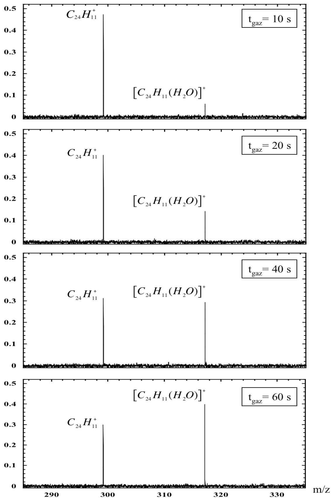
Figure 5.4: Spectres typiques de réactivité de C 24 H 11 + avec H 2 O ( Q = 10^{-6} \text{ mbar m}^3 \text{ s}^{-1} ) à 35 K en fonction du temps de réaction.
