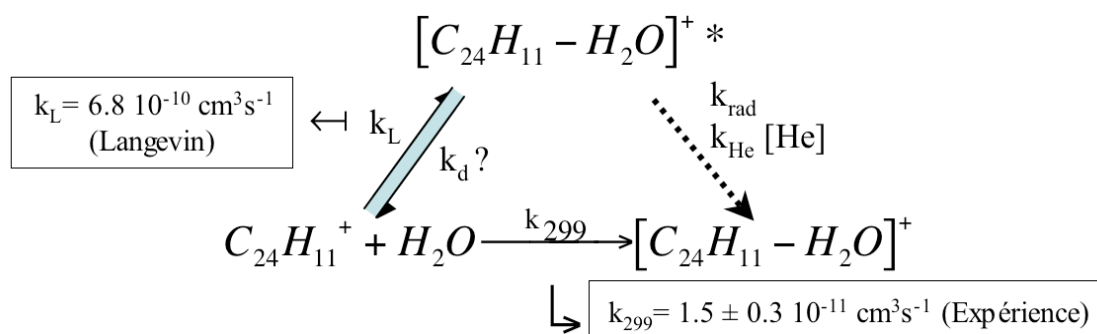
Figure 5.9: Théorie du complexe activé.
