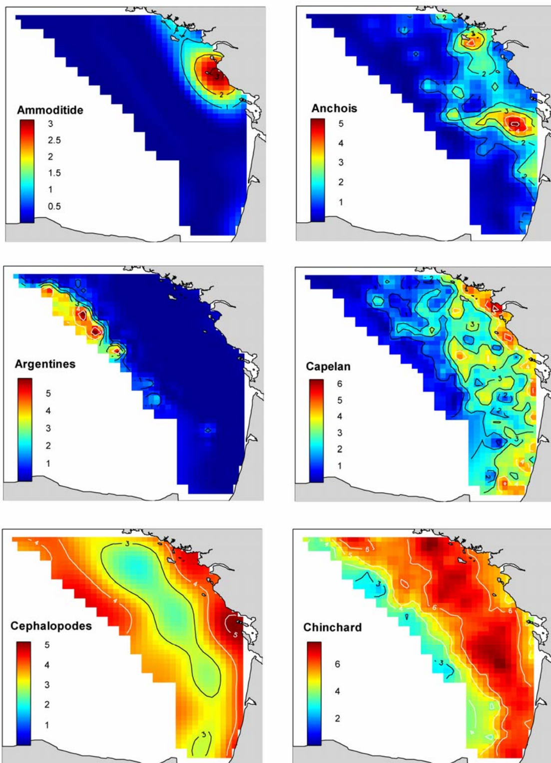
Fig 29. Cartographie des distributions spatiales (log abondances) des principales espèces de poissons pélagiques présentes en hiver dans le golfe de Gascogne
