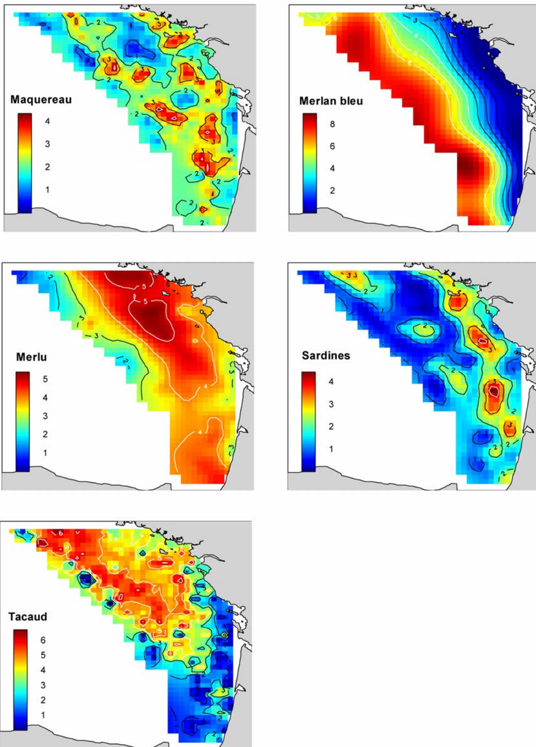
Fig 29-suite. Cartographie des distributions spatiales (log abondances) des principales espèces de poissons pélagiques présentes en hiver dans le golfe de Gascogne
