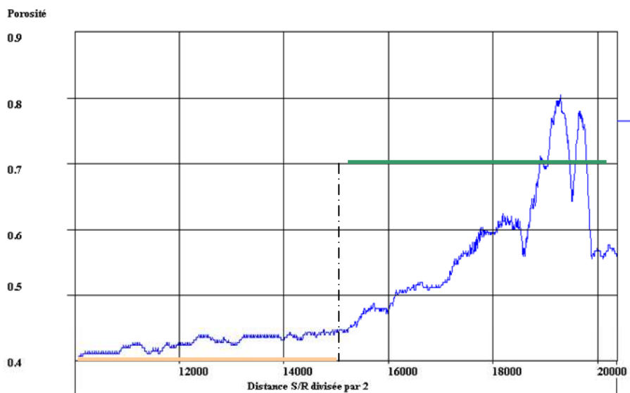
Figure 69 : Evolution de la valeur inversée de la porosité au cours de la radiale, les valeurs attendues sont 0.4 (Sable) jusqu'à 15 km puis 0.7 (Vase).
