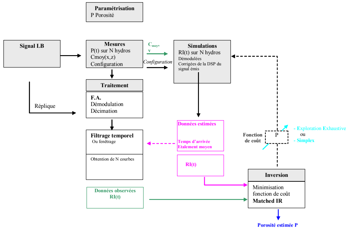
Figure 43 : Principe de la méthode globale d'inversion. Le module d'inversion ajuste le paramètre de porosité P , de telle sorte que la réponse impulsionnelle simulée ressemble le mieux à la réponse impulsionnelle observée.
