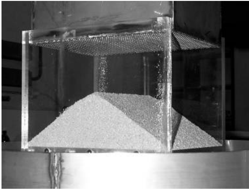
FIG. 3.19: Forme du prisme triangulaire construit par dépôt en couches horizontales.
