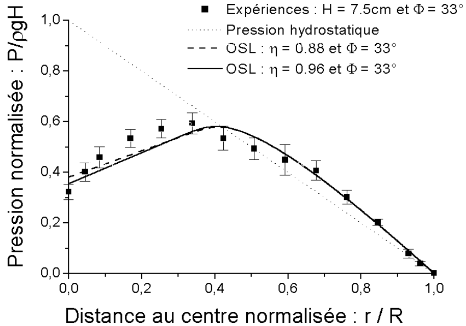
FIG. 3.29: Ajustement du modèle OSL à trois dimensions au profil de pression du tas conique construit à partir d'un point source.
