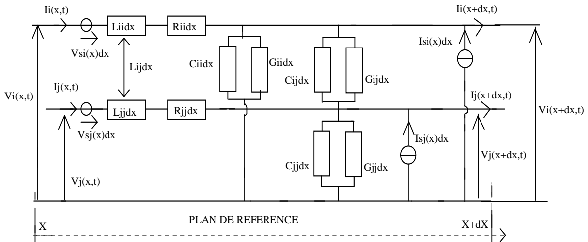
Figure II.1 - Elément infinitésimal d'une ligne composée de deux conducteurs et un plan de référence
