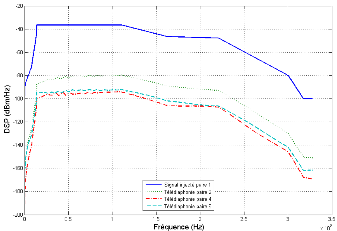
Figure II.14 - Télédiaphonie intra- et extra quarte d'un câble S98 14 paires de la boucle locale
