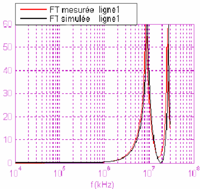
Figure V.12 - Rapport \frac{A}{R} (valeur absolue) - ligne 1
