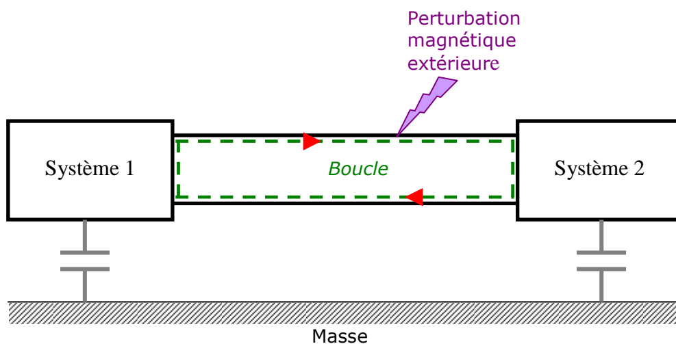
Figure I.9 - Couplage d'un champ magnétique avec la boucle formée par deux conducteurs proches
