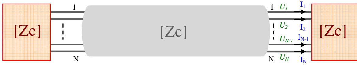
Figure III.1 - Adaptation d'une LMC
