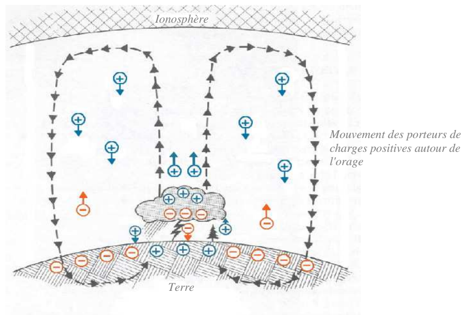
Figure I.4 - Circuit électrique atmosphérique global
