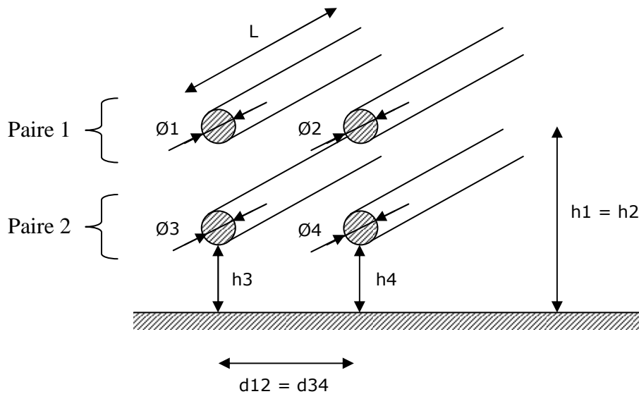
Figure II.9 - Configuration carrée d'un câble non écranté de quatre conducteurs
