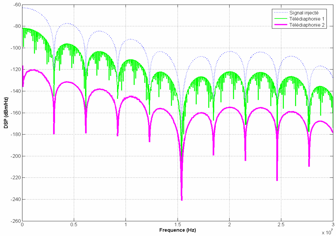
Figure IV.10 - Résultats fréquentiels
