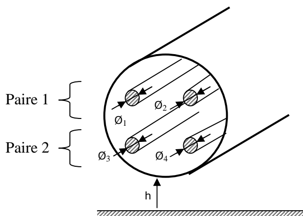
Figure III.5 - Ligne à quatre conducteurs dans blindage
