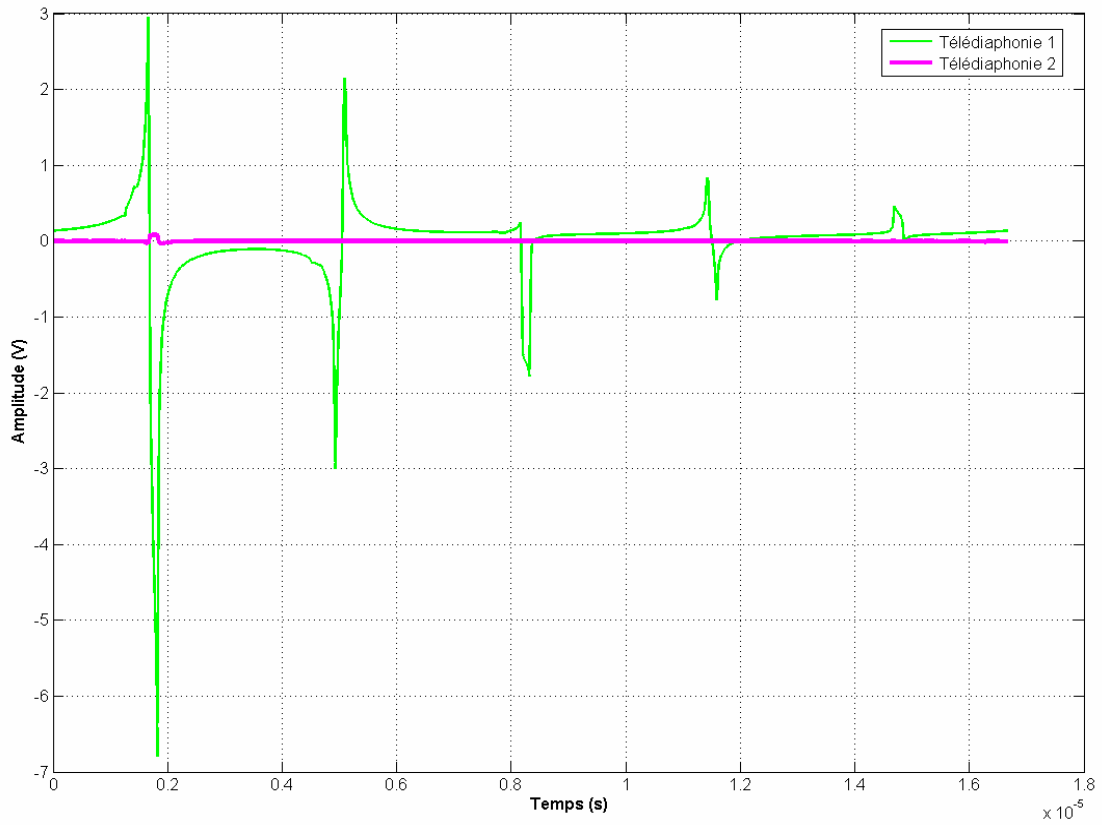
Figure IV.9 - Résultats temporels
