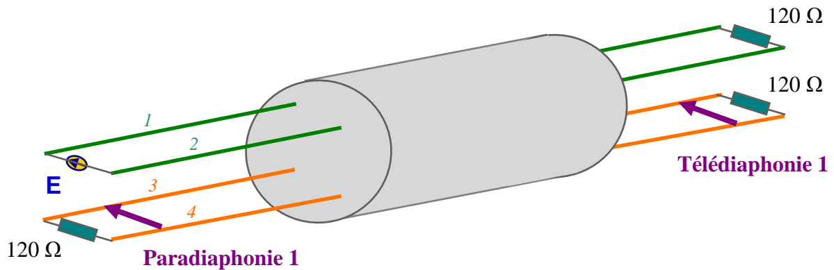
Figure III.6 - Première configuration
