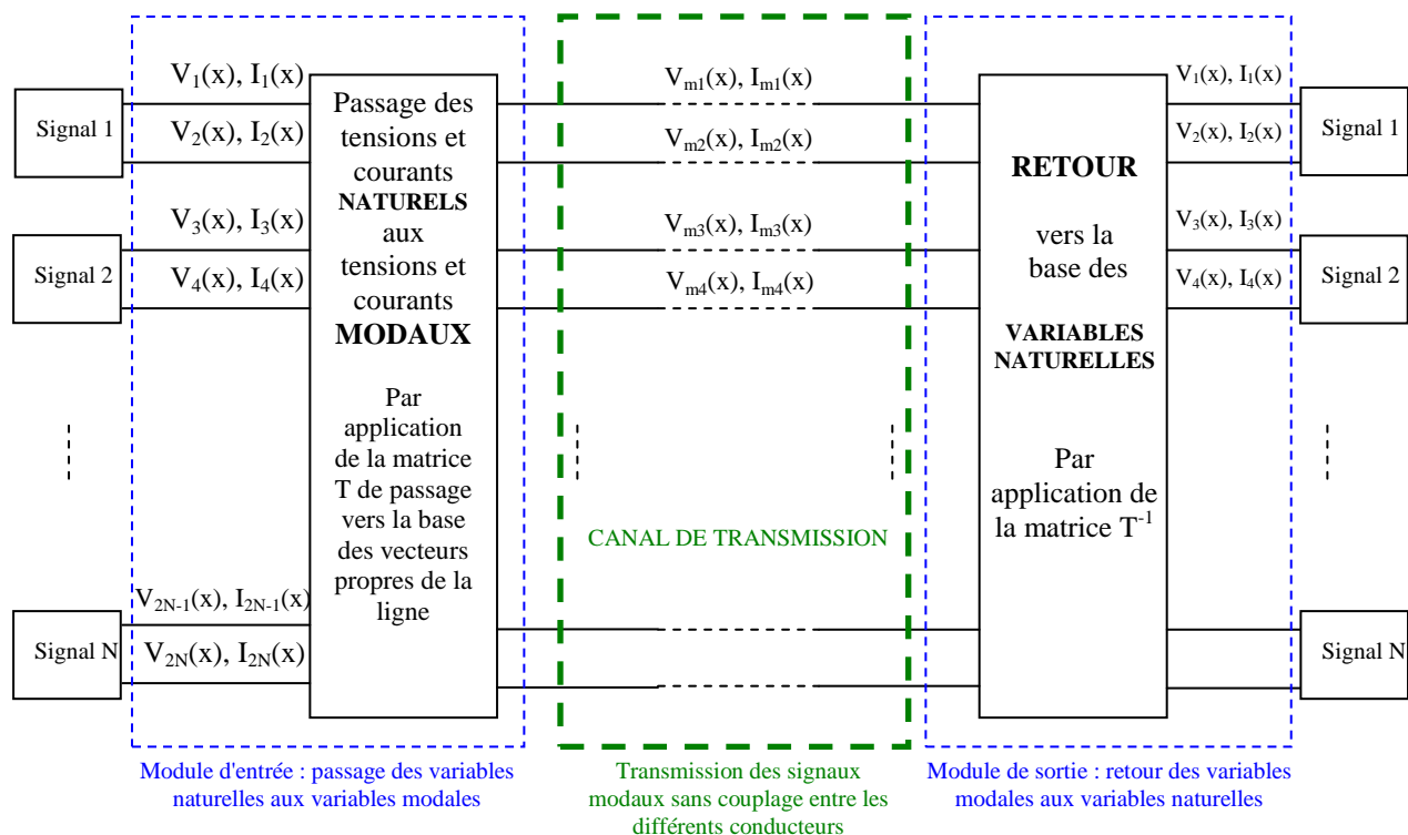
Figure IV.1 - Principe de la transmission suivant les modes propres de propagation
