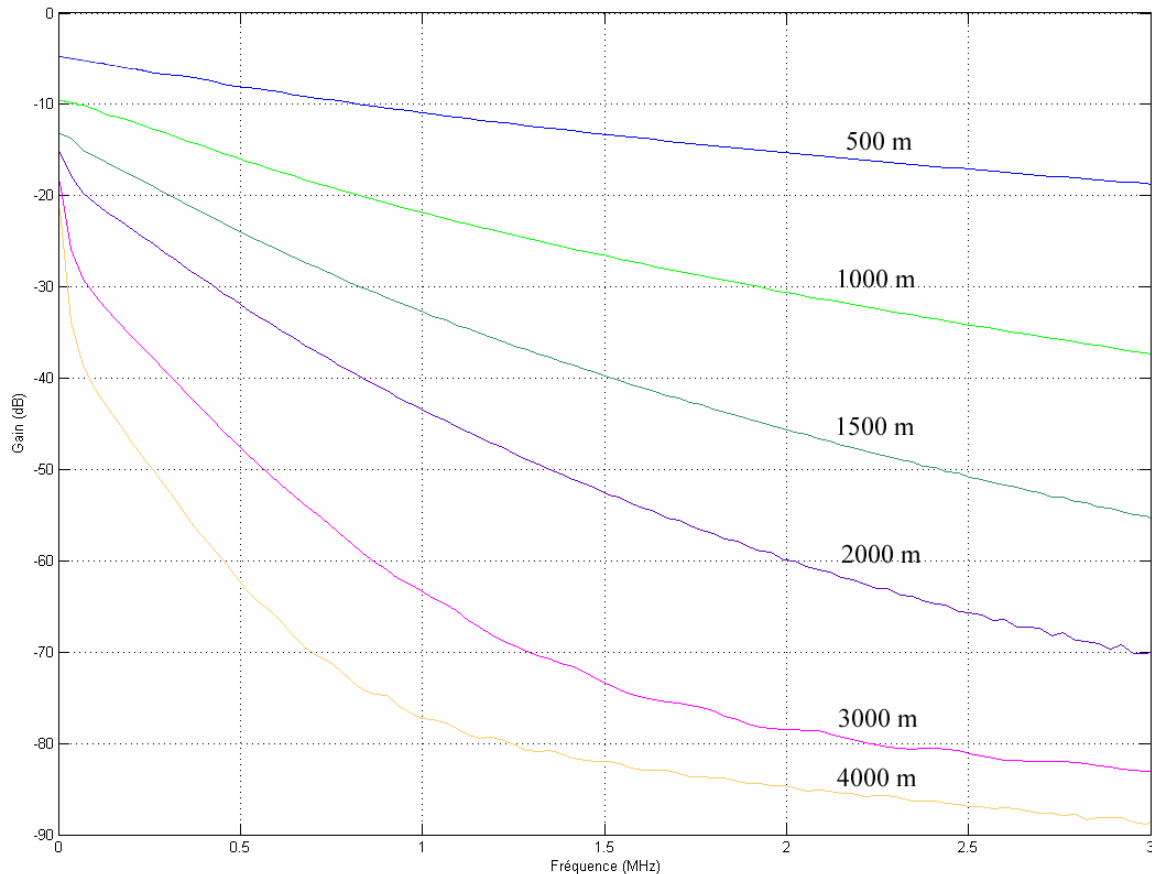
Figure I.20 - Atténuation de ligne d'une paire torsadée en fonction de la fréquence
