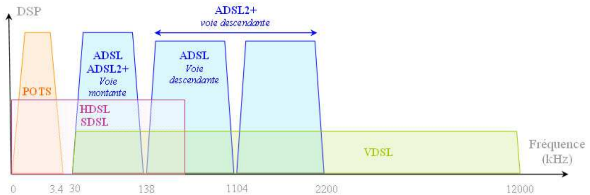
Figure I.15 - Organisation spectrale des systèmes xDSL
