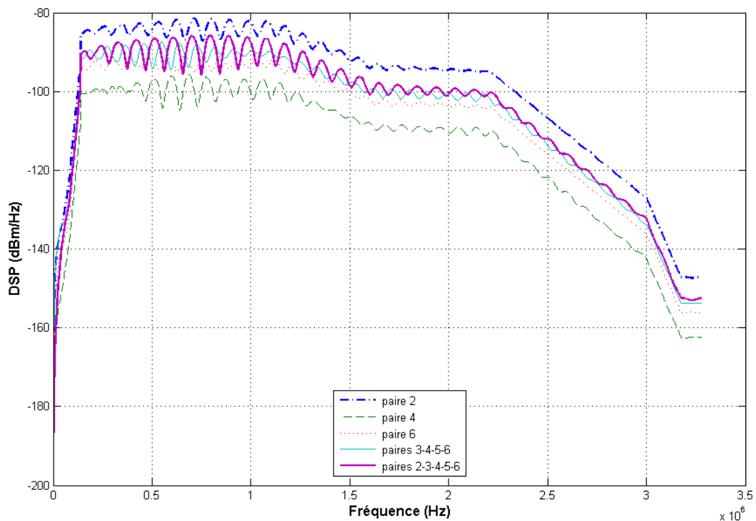
Figure II.15 - Paradiaphonie générée sur paire 1 suivant la/les paire(s) excitées
