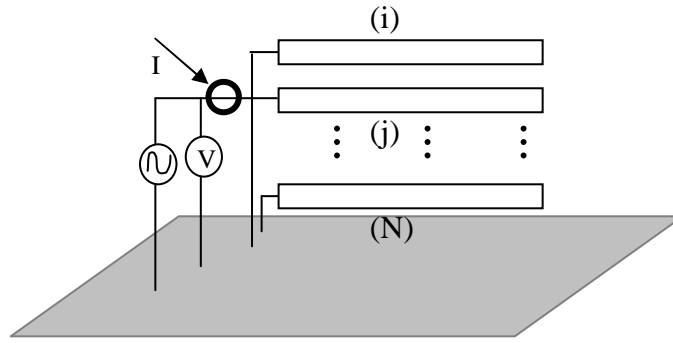
Figure A2 - Configuration d'excitation pour la mesure de l'admittance propre
