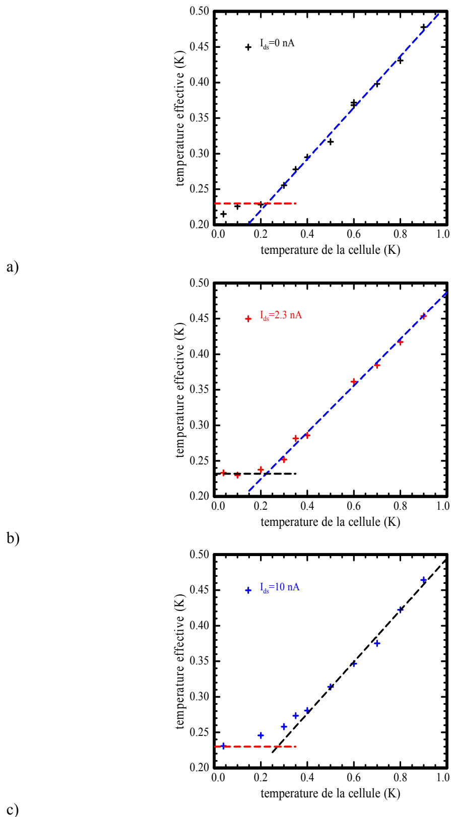
Figure 105 : évolution de la température effective de l'électron pour trois valeur du courant. a) pas de chauffage par le SET, le couant I_{ds} est nul. b) I_{ds}=2,3 nA. c) I_{ds}=10 nA . le courant modifie très légèrement les courbes. Avec un courant de 10 nA, on peut observer une augmentation de la température de l'électron lorsque la température de la cellule est comprise entre 200 mK et 400 mK. Au-delà de 400 mK, l'échappement est à nouveau dominé par les fluctuations thermiques.
