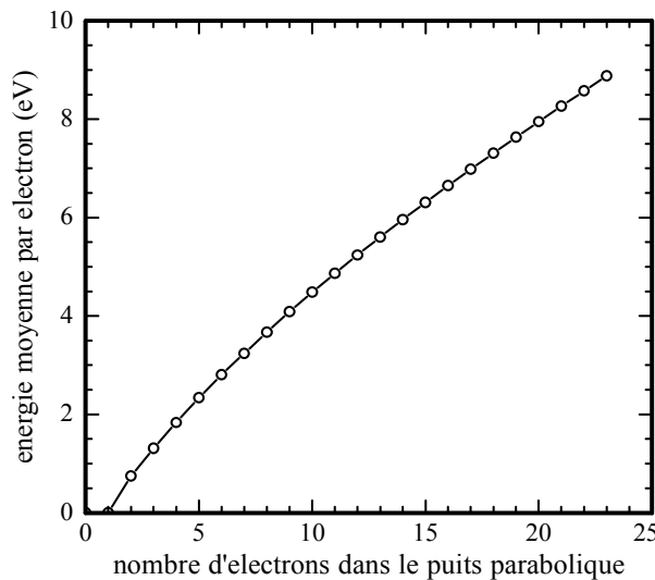
figure 73 : évolution de l'énergie moyenne par électron en fonction du nombre d'électrons (pour un confinement parabolique). L'énergie est en eV et normalisée par E_0 = (e^2/4\pi\epsilon_0)^{2/3} (m\omega_0/2)^{1/3} où \omega_0 est la fréquence du puits.
