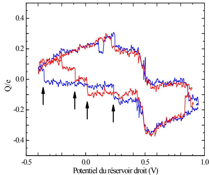
Figure 61: deux balayages (courbe rouge et courbe bleue) du réservoir droit en absence d'électrons. La phase des oscillations présente une boucle d'hystérésis traduisant le mouvement de charges dans le substrat de silicium. Les flèches marquent des sauts brusques de forte amplitude \sim 0.1e . il faut noter que ces sauts ne sont pas reproductibles.
