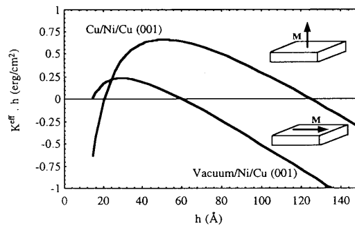
Figure III-2 : Variation de K_{eff}.h en fonction de l'épaisseur h de la couche de Ni, dans le système sandwich Cu(001)/Ni/Cu et Cu(001)/Ni/vidé en accord avec l'équation. D'après Bochi et al. [67].
