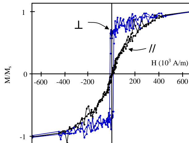
Figure III-3 : Cycles d'aimantation enregistrés par SQUID à température ambiante sur un échantillon Si(001)/Cu/Ni(4,5 nm)/Cu. Champ H appliqué // et \perp au plan du film.
