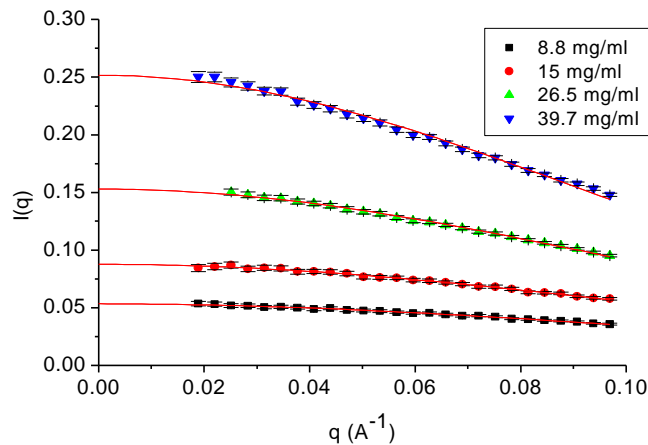
Figure III.12 : Intensité en fonction du vecteur d'onde pour une solution de BPTI à 22 °C.
