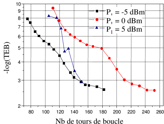
Figure 116 : Caractérisation de la boucle à vide en fonction de la puissance optique en entrée
