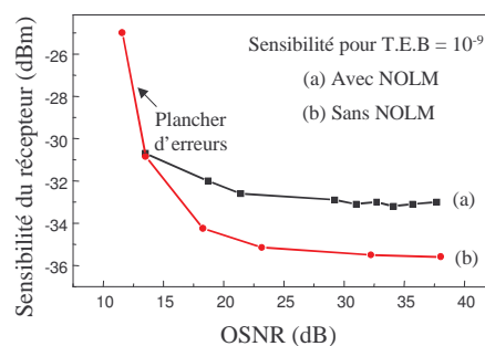
Figure 5: Caractérisation du récepteur en présence du régénérateur
