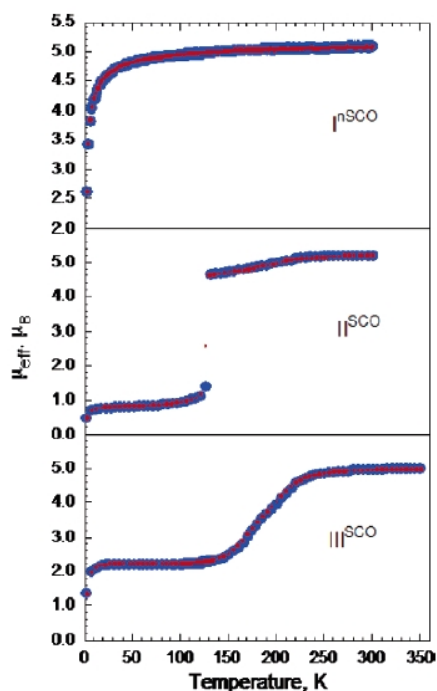
Figure III.5 : Moment magnétique effectif versus la température pour les polymorphes I, II et III de [Fe((p-IC_6H_4)B(Mepz)_3)_2] .
