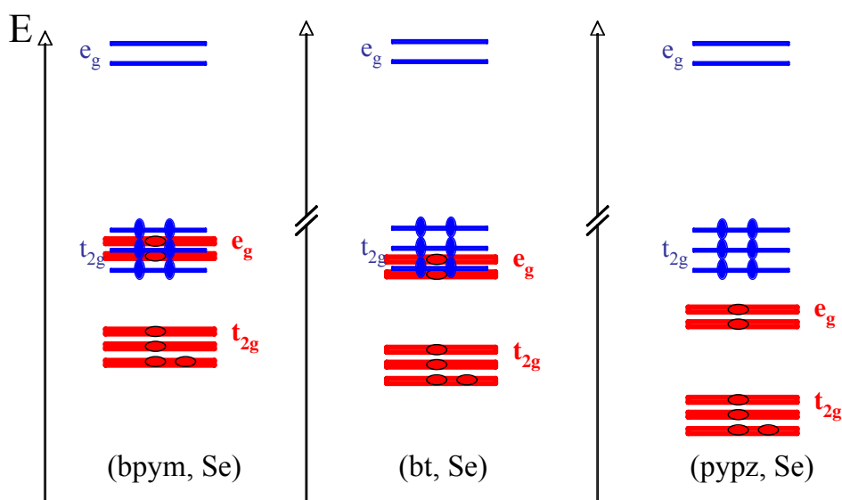
Figure IV.15 : Mélange des orbitales LS (lignes minces et courtes, les électrons désignés par des ellipses verticales) et HS à l'état [LS-HS]^{46} .
