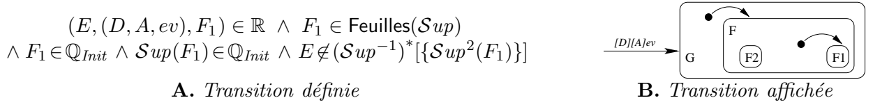
FIG. 5.4 – Exemple de transition en relation avec un sous-sous-état initial
