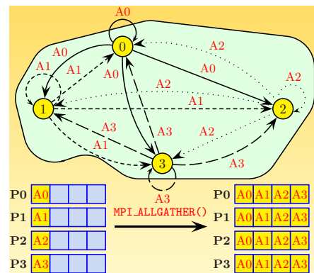
(d) MPI_Allgather
