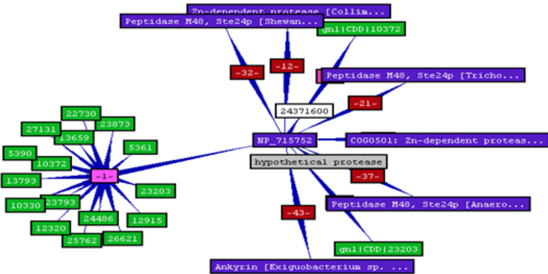
Figure 2.15 – BioMediator utilise TouchGraph pour visualiser le graphe résultat (visualisation basée sur un modèle physique).
