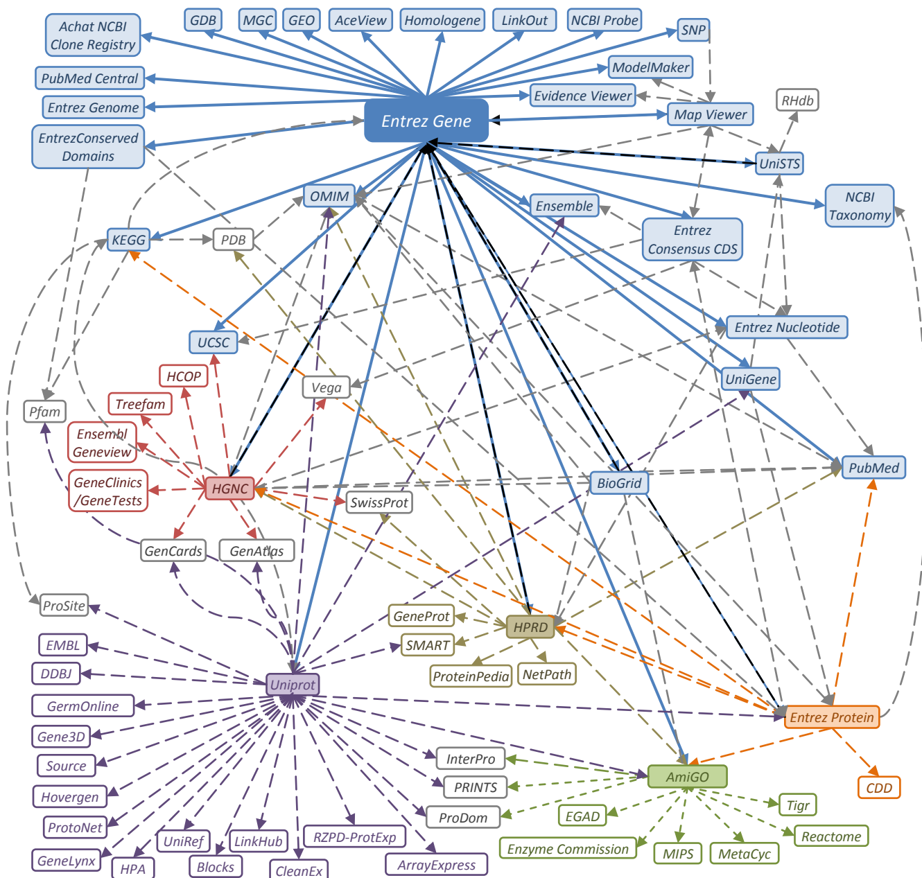
Figure 3.4 – Liste des sources accessibles en deux clics à partir d'Entrez Gene. Les boîtes pleines sont reliées par une flèche continue à Entrez Gene ; il s'agit des éléments accessibles à une distance de 1 clic. Les boîtes sur fond blanc et les flèches discontinues correspondent aux autres références croisées. Nous n'avons pas représenté les références croisées entre ces sources qui correspondraient à un troisième clic. Les couleurs ont été utilisées pour mieux suivre les origines et groupes de dépendances.
