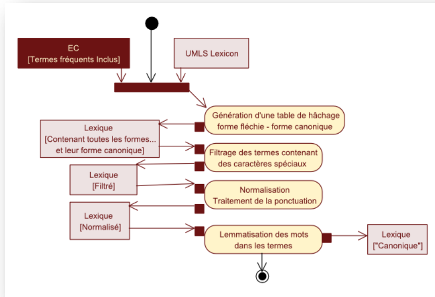
Figure 5.10 – Analyse lexicale – Normalisation du lexique
