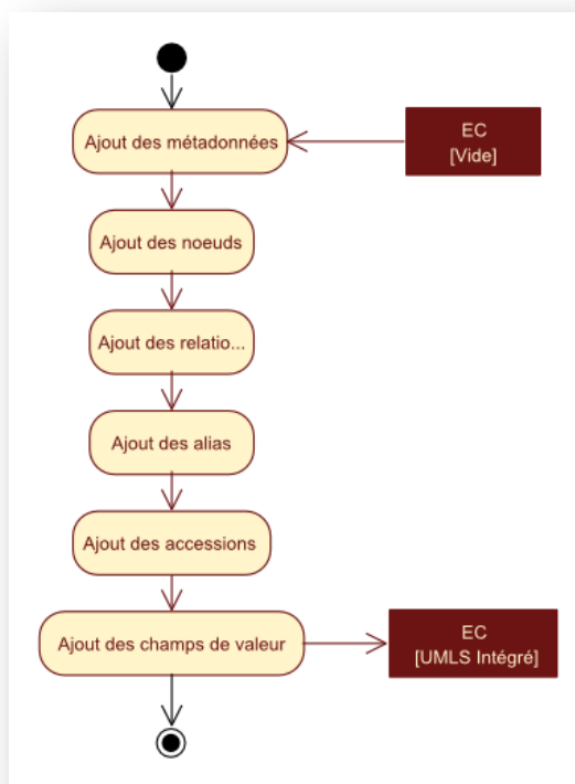
Figure 5.2 – Intégration d'UMLS
