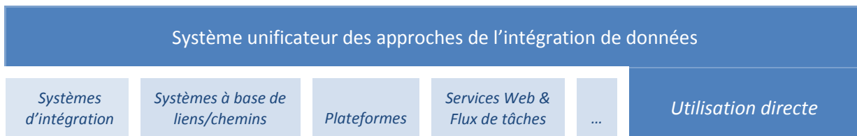
Figure 3.8 – Notre approche (blanc sur bleu foncé) se positionne comme une couche unificatrice favorisant l'interopérabilité des approches existantes. Elle propose un ensemble de services et d'outils fonctionnels permettant le développement rapide d'applications métiers accédant aux données intégrées et les visualisant.
