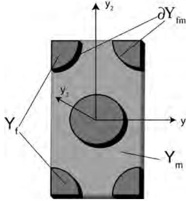
FIG. 3.4 – Représentation schématique du VER.
