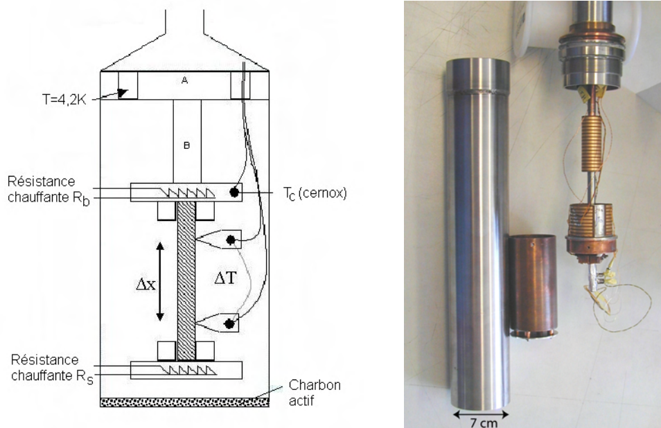
FIG. 4.10 – Schéma et photo du dispositif expérimental.
