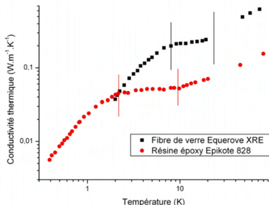
FIG. 2.2 – Evolution de la conductivité thermique de la résine époxyde (Epikote 828) [38] et de la fibre de verre E (Equerove XRE) [54] en fonction de la température.
