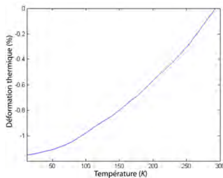
FIG. 6.2 – Evolution de la déformation thermique de la résine époxyde en fonction de la température [60].
