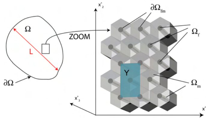
FIG. 3.1 – Représentation schématique d'un composite unidirectionnel.
