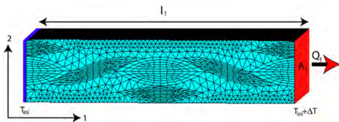
FIG. 4.8 – Exemple de détermination de \Lambda_{11} .
