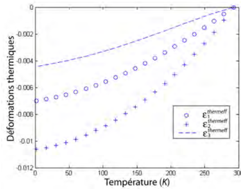
FIG. 8.5 – Déformations thermiques du composite tressé homogénéisé.
