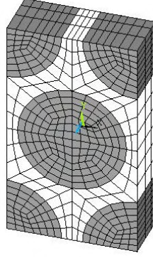
FIG. 3.5 – Maillage du VER microscopique.
