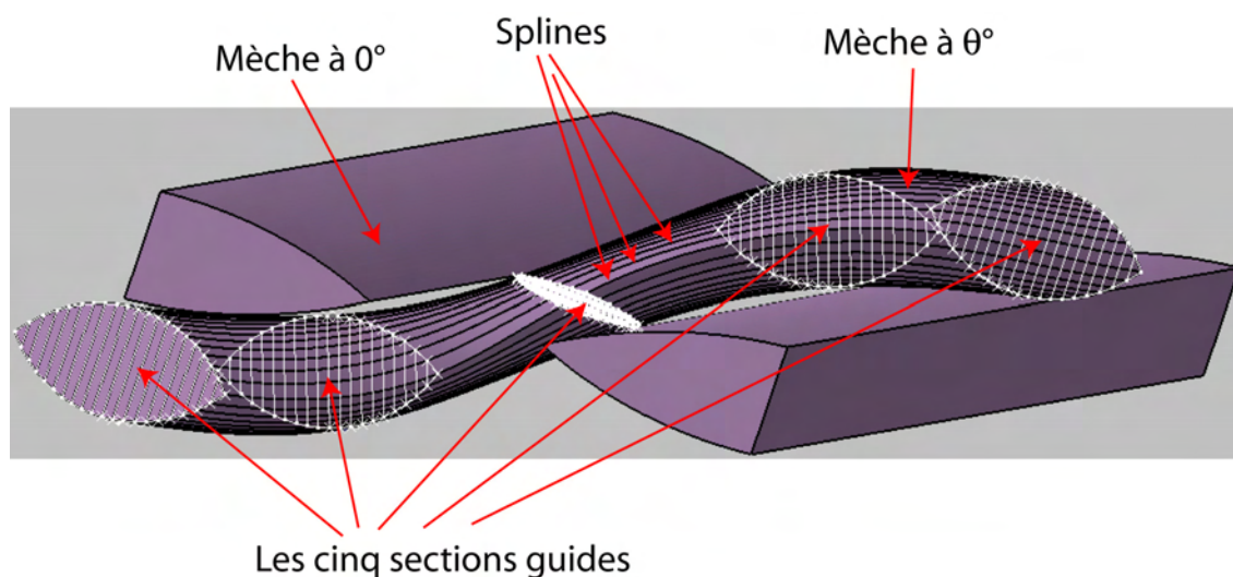
FIG. A.1 – Géométrie des mèches.
