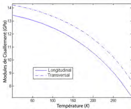
FIG. 7.5 – Evolution des modules de cisaillement.
