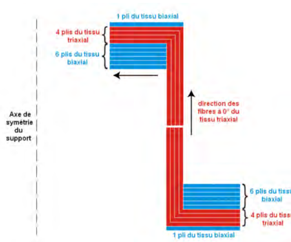
FIG. 1.6 – Séquence d'empilement des plis dans le support.
