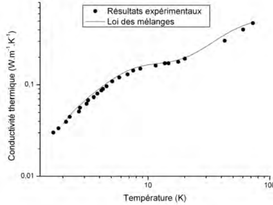
FIG. 2.3 – Conductivités thermiques longitudinales calculée et expérimentale [54] pour un composite unidirectionnel en verre/époxyde ( v_f=0,70 ).
