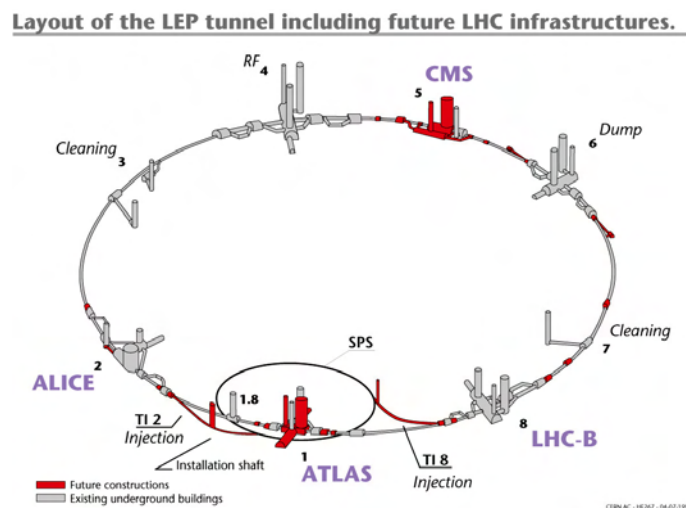
FIG. 1.2 – Disposition des détecteurs [1].
