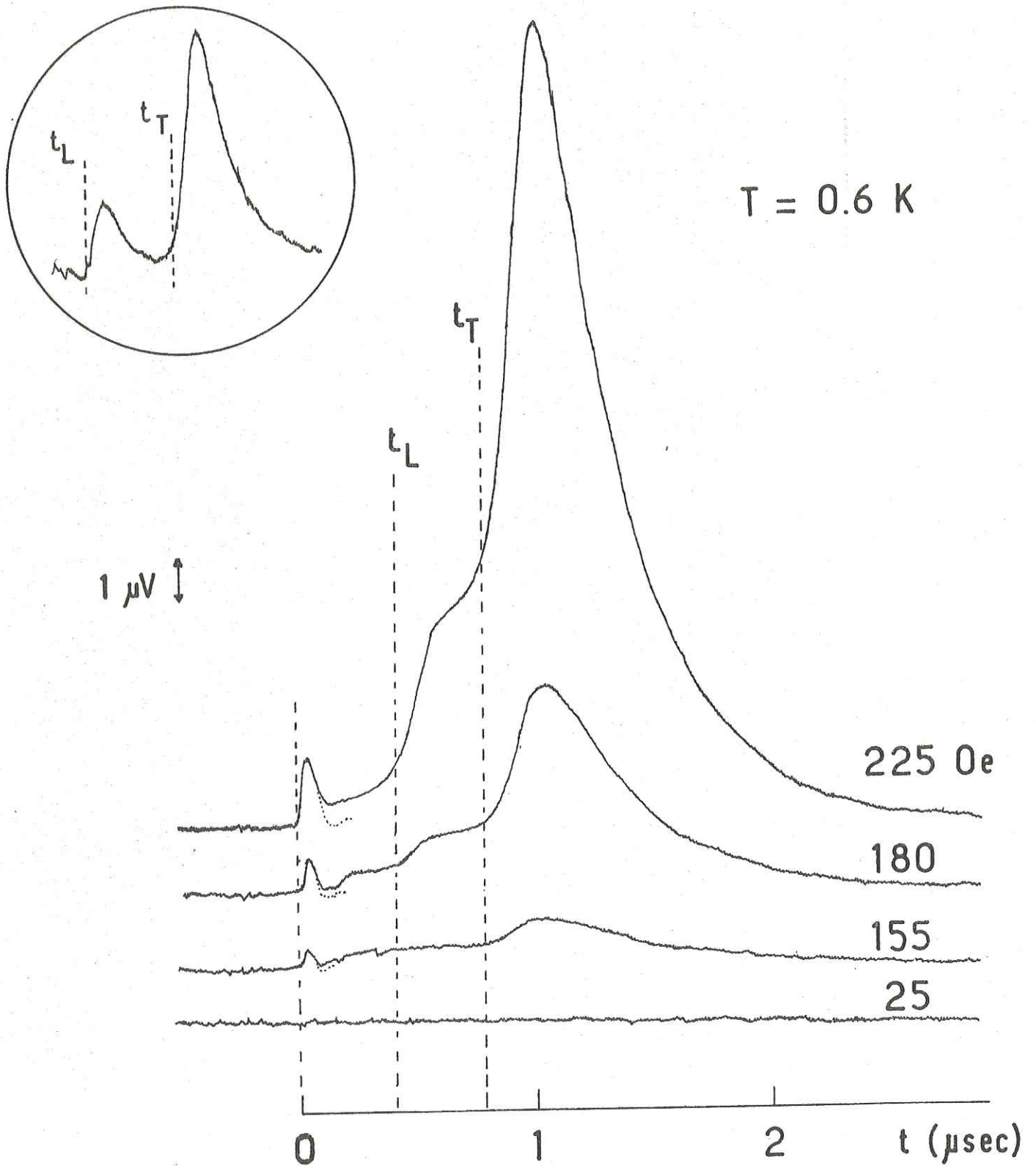
Fig. 4 : Signaux détectés à 0.6 K pour différents champs magnétiques. De bas en haut \nu_{det}(H) vaut respectivement 280, 230, 215 et 200 GHz. Pour comparaison, 2\Delta_{SN}/h=240 GHz. Photoexcitation. t_L et t_T sont les temps d'arrivée théoriques des phonons balistiques. En médaillon, pics de phonons produits par un émetteur de chaleur (extraits de Fig. III 13). Noter l'absence du mode mixte et l'apparition, en champ H \neq 0 du pic additionnel à t=0 qui subsiste même si la jonction est polarisée à courant nul (pointillés).
