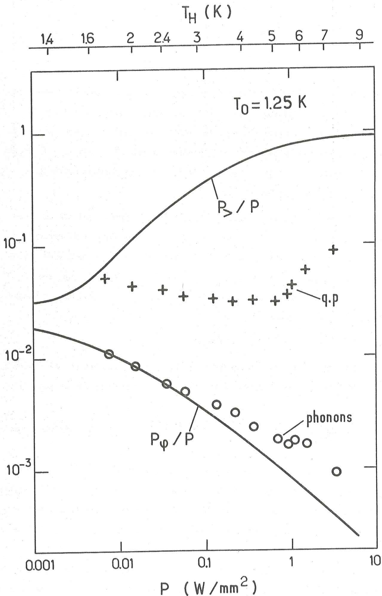
Fig. 2 : Fraction de la puissance transférée au mode mixte ( P_m/P ) et aux phonons de basse fréquence ( P_\phi/P ) en fonction de la puissance d'émission. Modèle du corps noir : ——. Amplitude du mode mixte (+) et des phonons balistiques (o) divisées par P . En haut : échelle des températures d'émetteur calculées d'après le modèle du corps noir.
