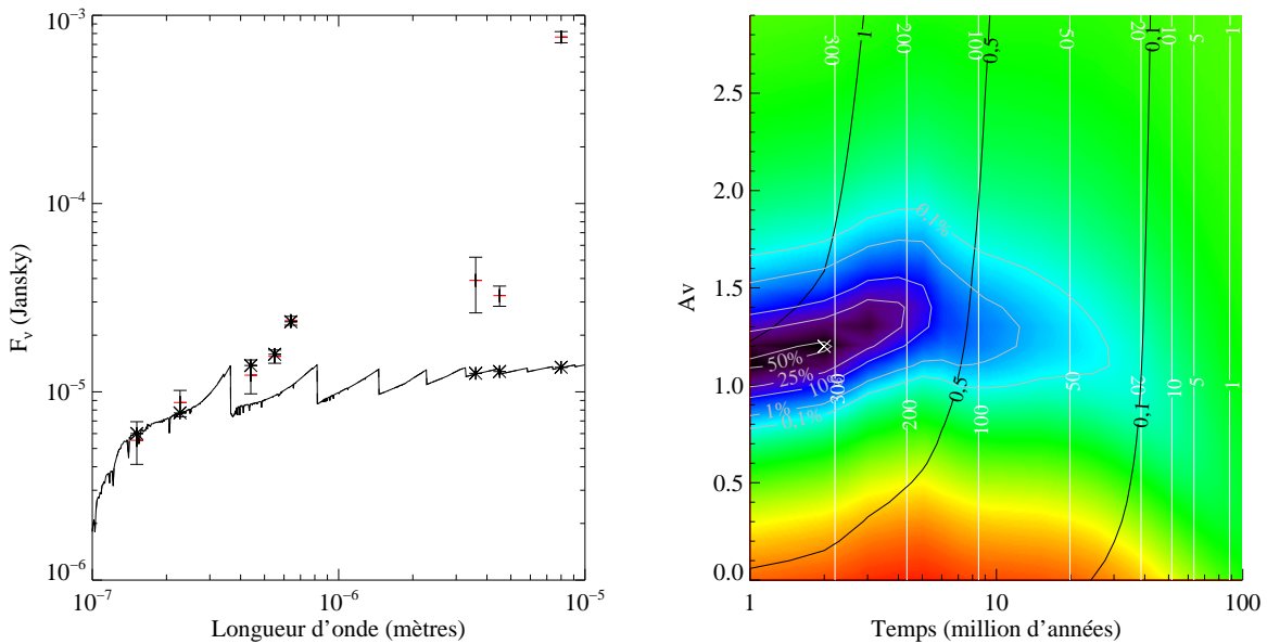
FIGURE 6.8 – Modélisation de la région 5 du Quintette de Stephan avec un rapport de masses valant r = 10^2 et une constante de temps \tau = 13 \cdot 10^6 ans. L'ajustement est effectué en prenant en compte les flux dans les bandes FUV, NUV, B, V et R. Voir la figure 6.6.
