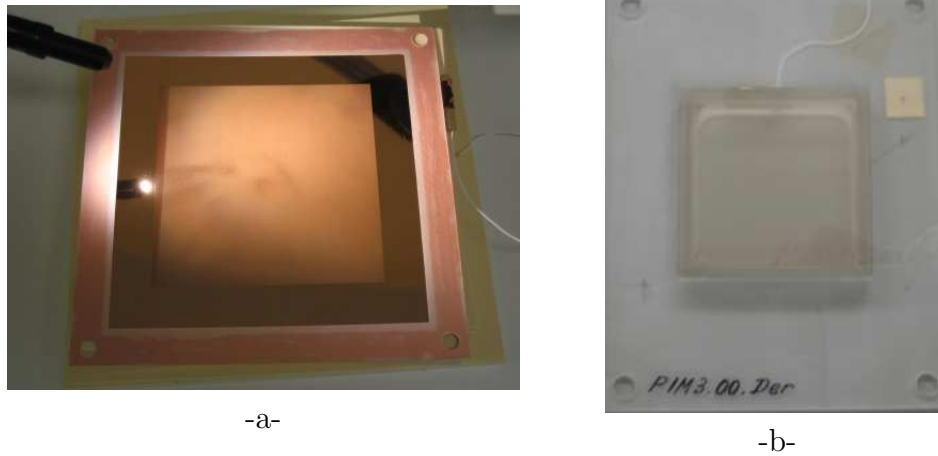
FIG. 2.4 – Photographies d’une micro-grille (CERN_μgrille_50c) tendue et collée sur un cadre fin FR4 (a) et d’une grille 500 LPI collée sur un cadre plexiglas (b).
