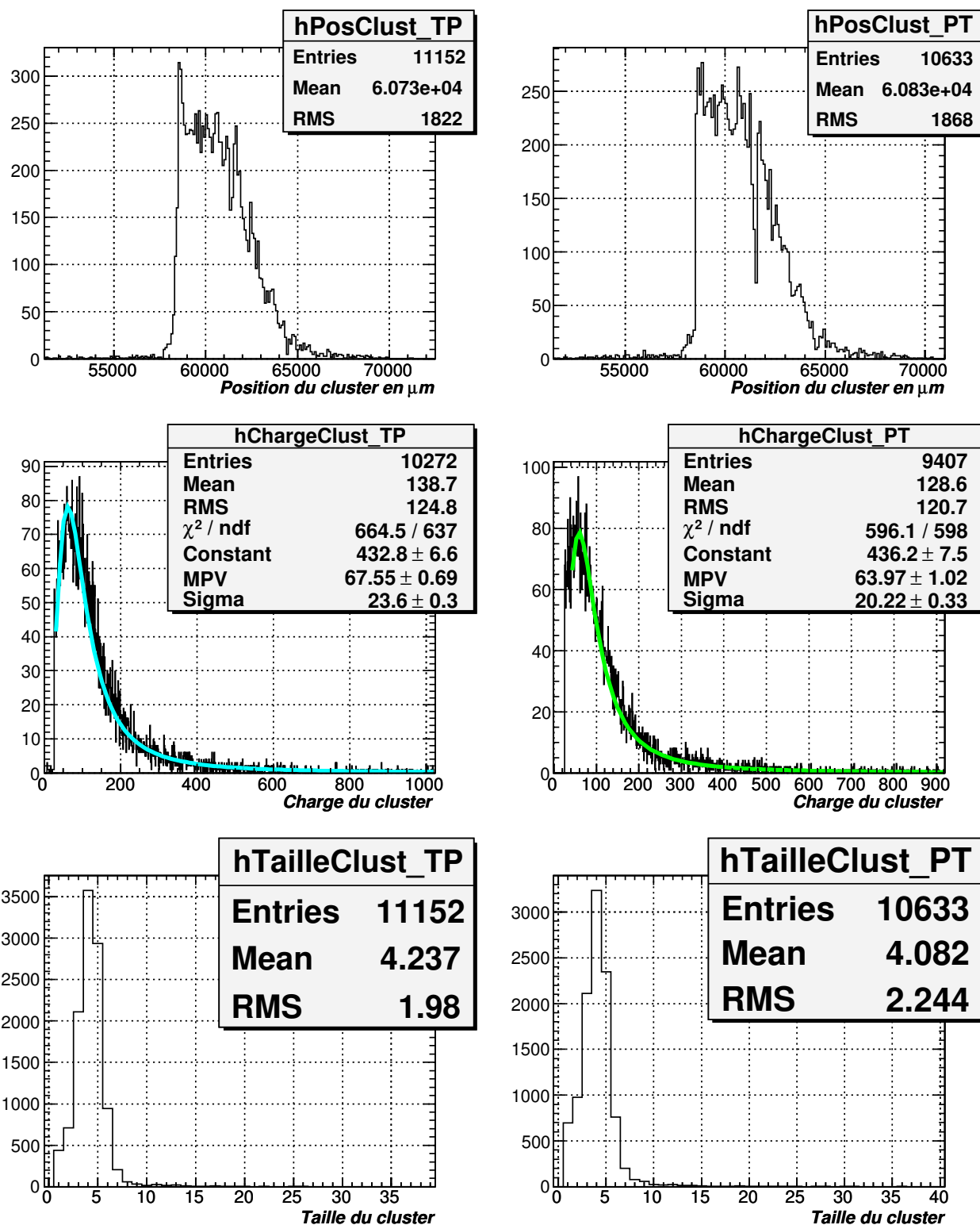
FIG. 3.16 – Distributions de la position, de la charge et de la taille du cluster pour chaque détecteur du doublet. Le champ électrique appliqué dans l'étage de pré-amplification ( E_{A2} ) était de 28 kV/cm.
