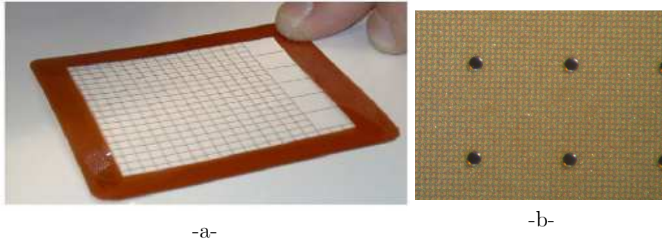
FIG. 2.3 – Photographies d'un espaceur en Kapton découpé au laser (a) et des plots en Kapton d'une grille (CERN- \mu grille-50c) (b).
