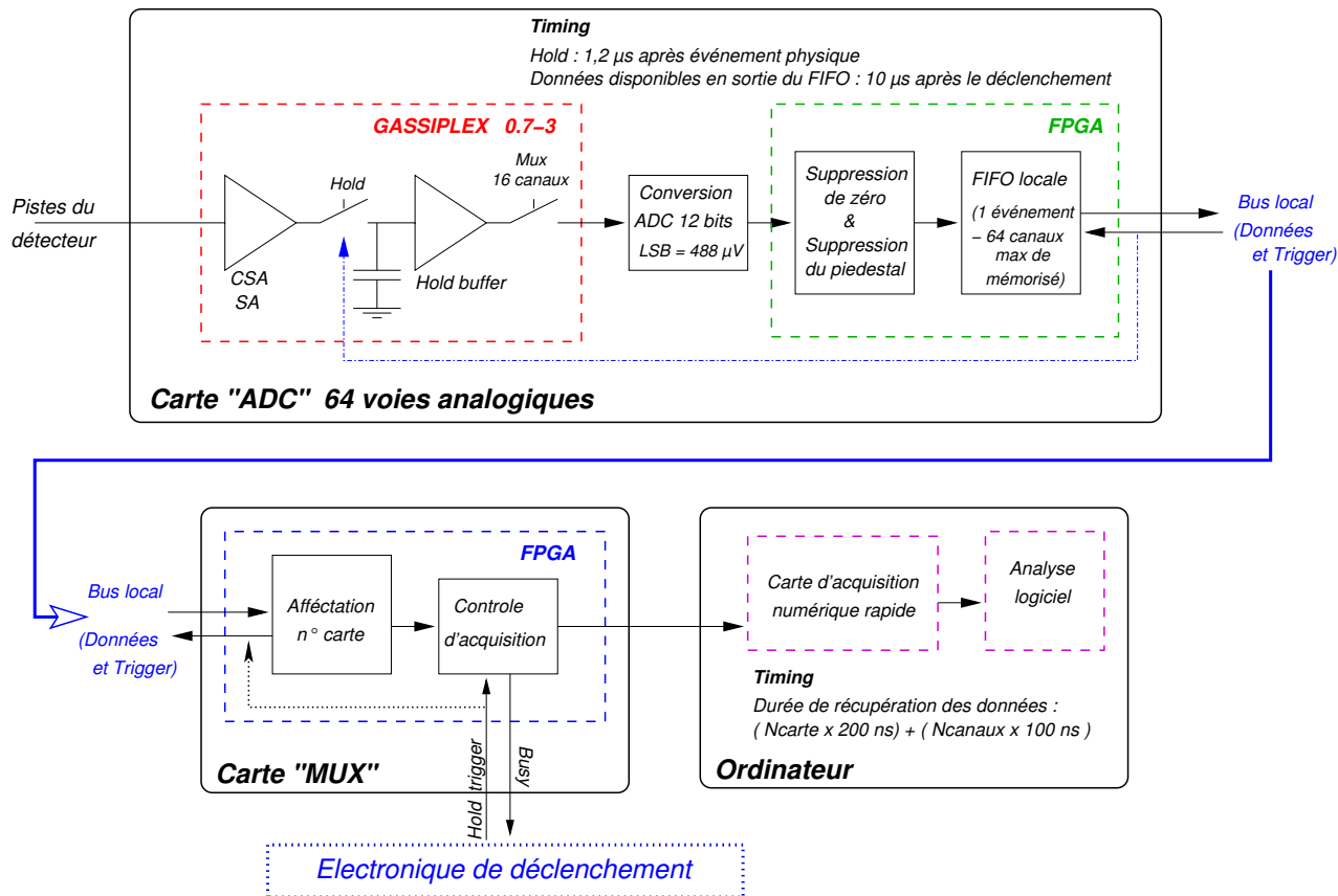
FIG. 3.3 – Structure de la chaîne électronique d'acquisition.
