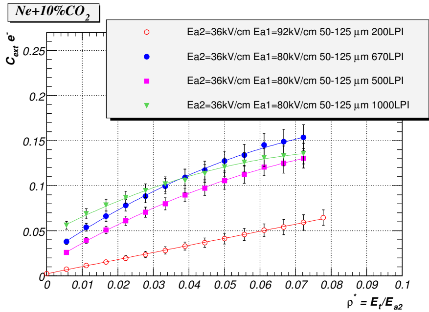
FIG. 2.13 – Coefficient d'extraction mesuré avec le prototype PIM 3 en configuration 50-125 \mu\text{m} pour diverses grilles en fonction de rapport de champ ( \frac{E_t}{E_{A2}} ).
