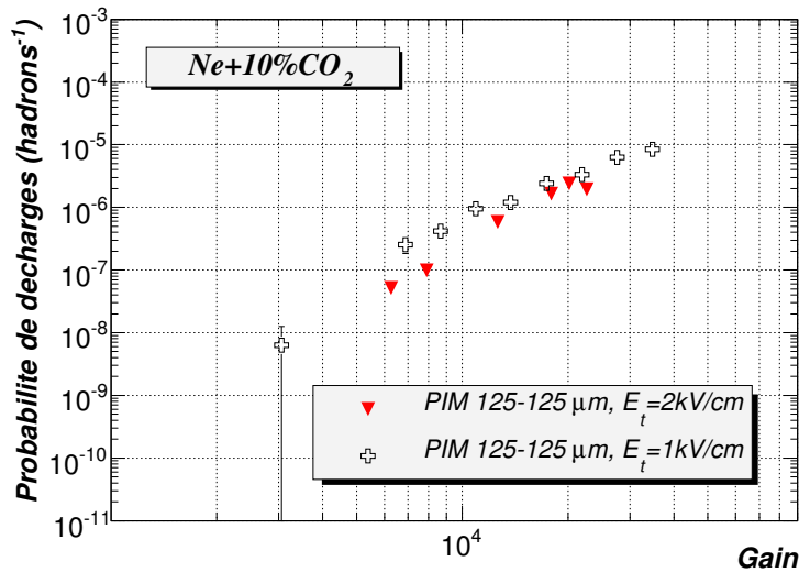
FIG. 4.13 – Comparaison de la probabilité de décharge mesurées avec la configuration 125-125 \mu m pour deux valeurs du champ électrique de l'espace de transfert ( E_t ). Le champ électrique de l'espace de pré-amplification ( E_{A2} ) pour ces deux séries de données est de 30 kV/cm.
