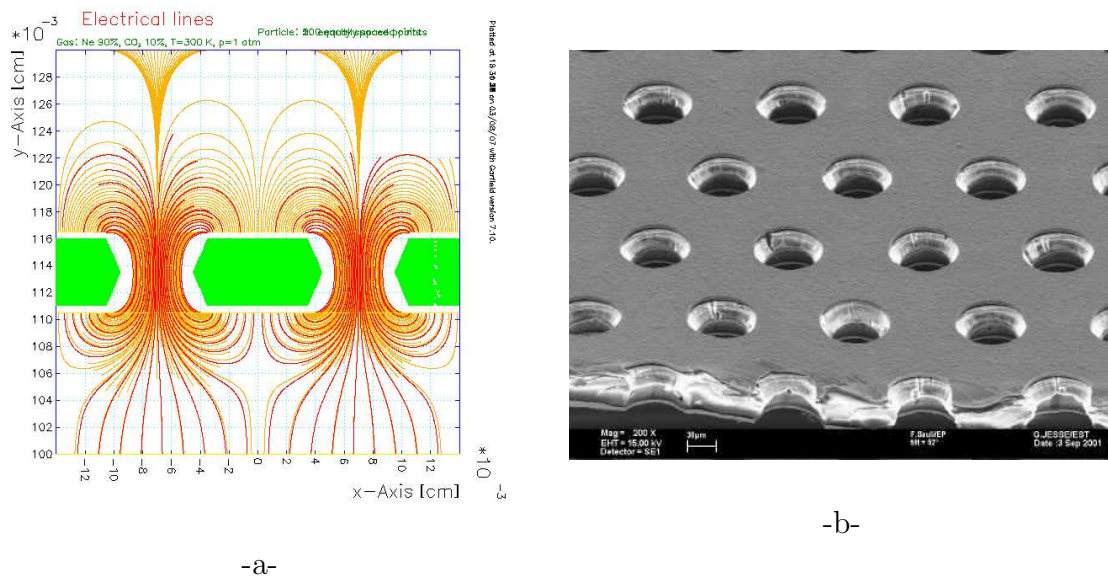
FIG. 3 – Schéma des lignes de champs (figure de gauche) et photographie d'une grille GEM (figure de droite).
