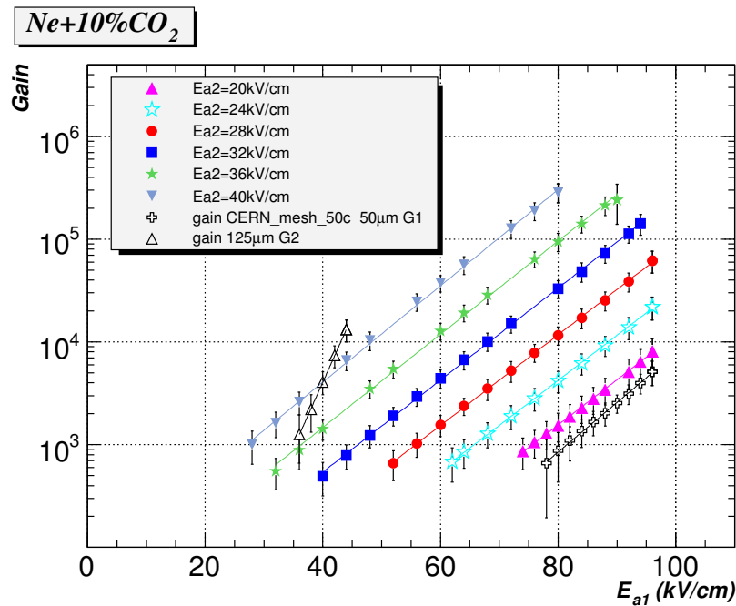
FIG. 2.24 – Gain mesuré pour une configuration 50-125 \mu m avec une grille 670 LPI.
