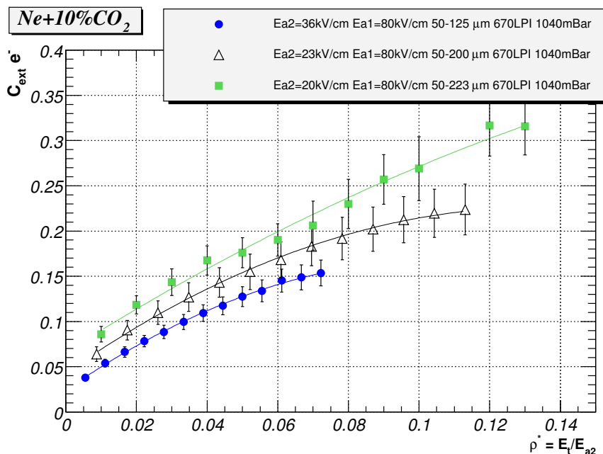
FIG. 2.16 – Coefficient d'extraction mesuré pour une grille 670 LPI pour trois gaps d'amplification (125, 200 et 220 \mu\text{m} ).
