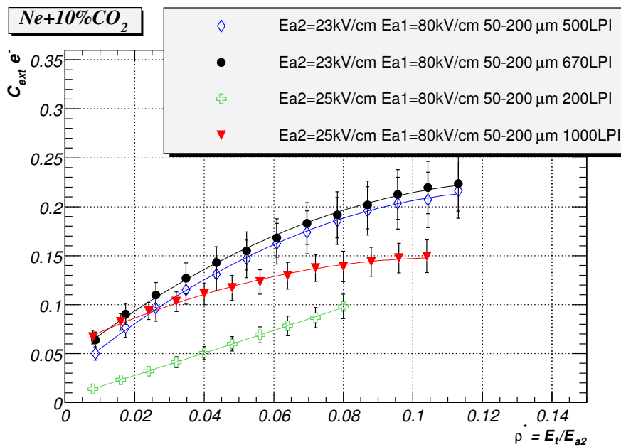
FIG. 2.14 – Les mêmes mesures réalisées avec cette fois-ci une configuration géométrique du détecteur PIM 3 : 50-200 \mu\text{m} .
