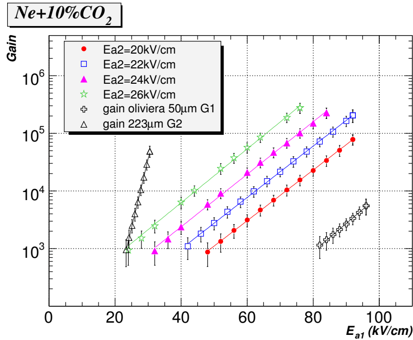
FIG. 2.23 – Série de mesures de gain obtenue avec une configuration 50-220 \mu m pour différentes polarisations des grilles constituant les espaces d'amplification. La pression du gaz était maintenue constante à une valeur de 1040 mbar.
