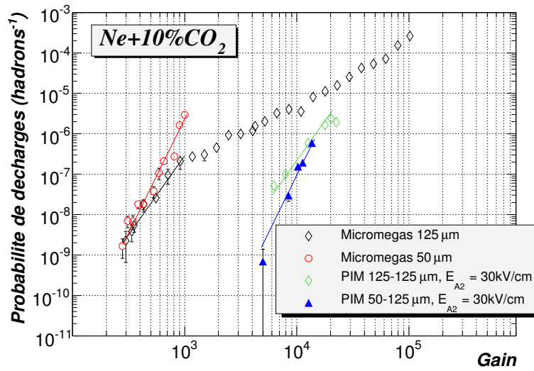
FIG. 4.11 – Comparaison des probabilités de décharge pour les configurations possédant un étage de pré-amplification de 125 \mu\text{m} .
