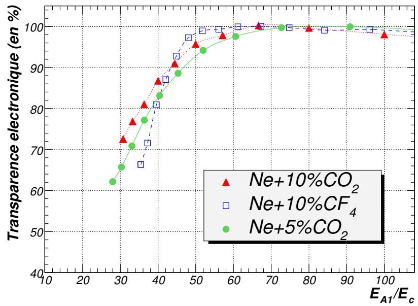
FIG. 2.12 – Transparence électronique en fonction du rapport de champ ( \frac{E_{amp}}{E_c} ) mesurée pour une grille CERN_μgrille_50c à l'aide d'une source ^{55}Fe . Ces tests ont été réalisés avec différents mélanges gazeux.
