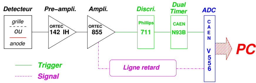
FIG. 1.17 – Schéma de la chaîne électronique utilisée pour les mesures de gain.
