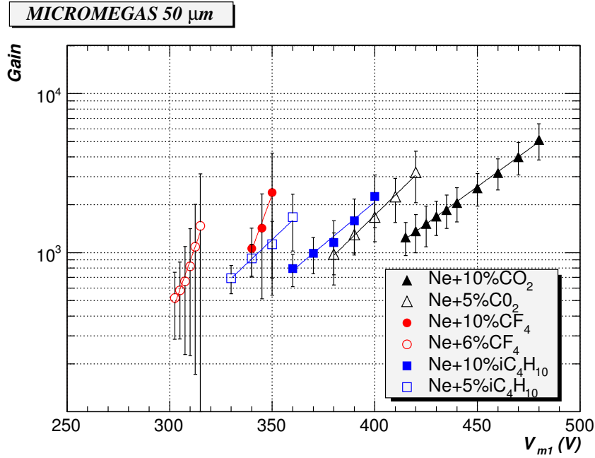
FIG. 1.22 – Gain du détecteur MICROMEGAS (50 μm) en fonction de la tension de polarisation de la micro-grille ( V_{m1} ) mesuré pour différents mélanges gazeux.
