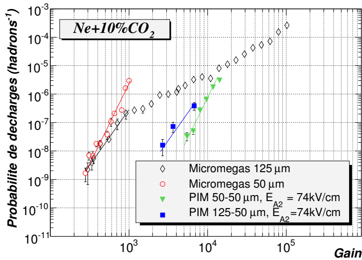
FIG. 4.10 – Comparaison des probabilités de décharge pour les configurations possédant un étage de pré-amplification de 50 μm.
