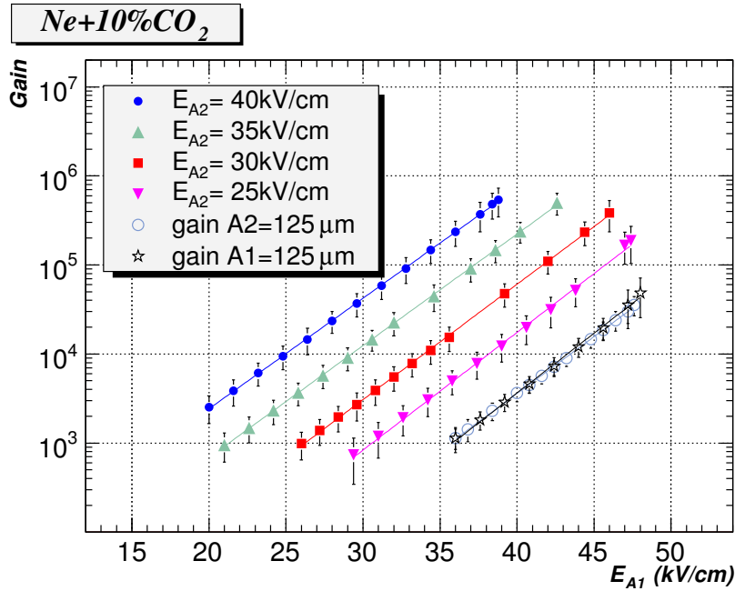
FIG. 2.18 – Gain du détecteur PIM3 en fonction du champ d’amplification E_{A1} pour le mélange \text{Ne}+10\%\text{CO}_2 . Le gain dans l’étage d’amplification A1 correspond à un champ dans l’étage de pré-amplification ( E_{A2} ) nul, tandis que le gain A2 (étage de pré-amplification) a été obtenu en fonction du champ E_{A2} pour un champ E_{A1} égal à zéro.
