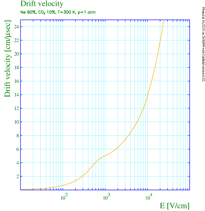
FIG. 1.6 – Vitesse de dérive des électrons dans du \text{Ne}+10\%\text{CO}_2 ( P=1 \text{ atm} et T=300\text{K} ) calculé par MAGBOLTZ (implémenté dans GARFIELD [Vee98]) en fonction du champ électrique E .
