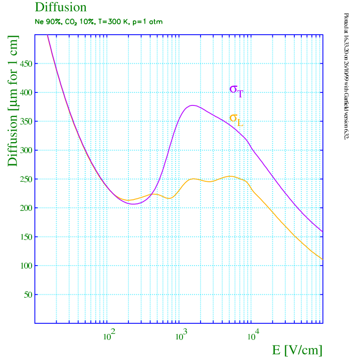
FIG. 1.8 – Diffusion transverse et longitudinale en fonction du champ électrique E calculé avec MAGBOLTZ pour un mélange Ne+10\%CO_2 ( P=1\text{ atm} et T=300K ).
