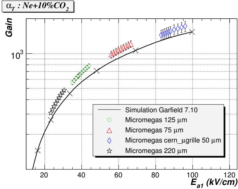
FIG. 1.20 – Facteur de multiplication effectif calculé à partir des mesures de gain de MICROMEGAS comparé au coefficient de Townsend simulé pour le mélange gazeux \text{Ne}+10\%CO_2 avec MAGBOLTZ.
