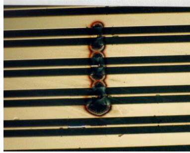
FIG. 2 – Exemple de détériorations provoquées par des décharges sur les pistes d'une MSGC.
