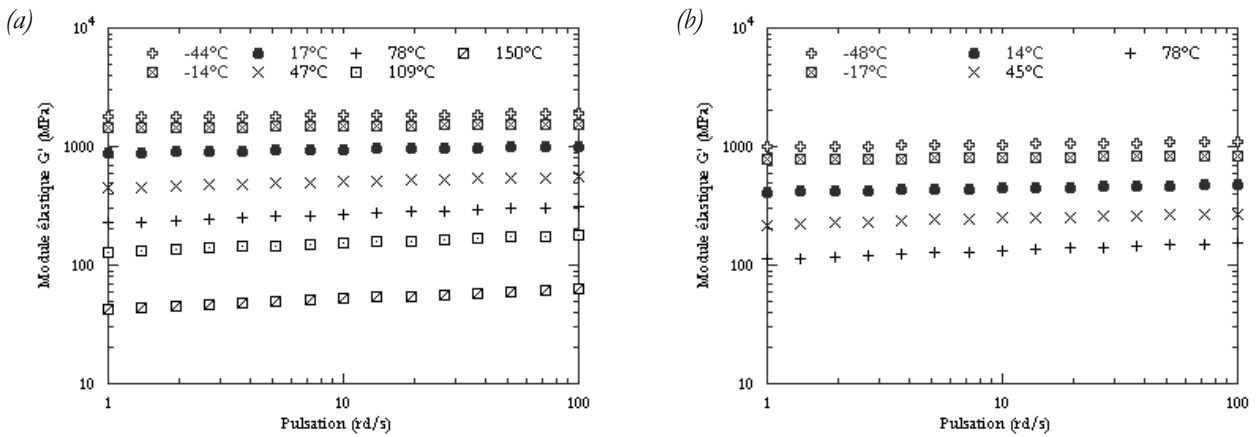
Fig. II-9 Sensibilité du module élastique du BMT222 (a) et du BA238G9 (b) à la pulsation de la sollicitation pour une vitesse de chauffage de 1^{\circ}\text{C}/\text{min} . Eprouvettes usinées dans le sens longitudinal.
