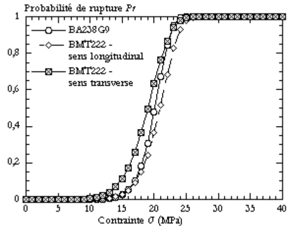
Fig. IV-17 Probabilité de rupture en fonction de la contrainte à rupture en traction corrigée des effets de la dissipation intrinsèque.
