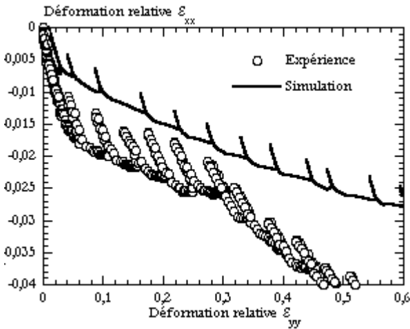
Fig. V-26 Evolution de la déformation transverse mesurée ou issue de la simulation d'essais de traction cyclique du BA238G9.
