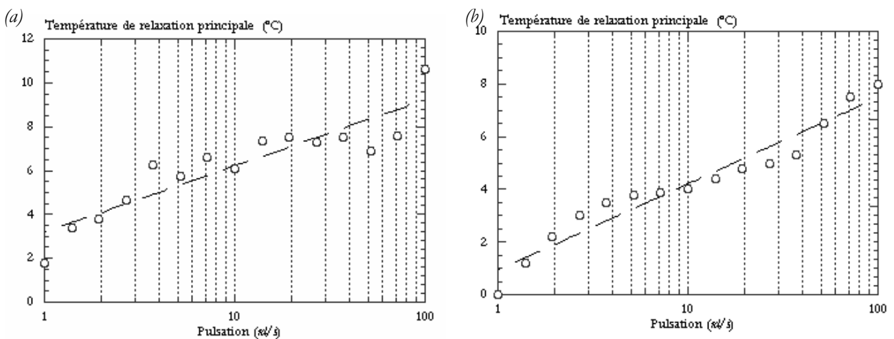
Fig. II-11 Variation de la transition principale du BMT222 (a) et du BA238G9 (b) en fonction de la pulsation. \circ : Points expérimentaux. — : Interpolation linéaire.
