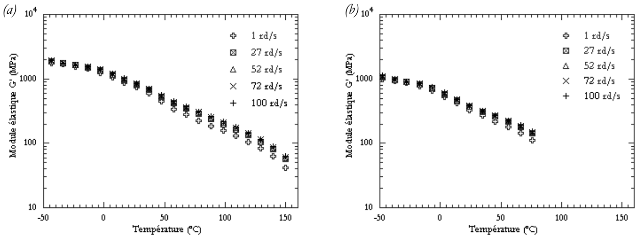
Fig. II-10 Sensibilité du module élastique à la température du BMT222 (a) et du BA238G9 (b) pour une plage de pulsation de 1 et 100 \text{rd}/\text{s} et une vitesse de chauffage de 1^{\circ}\text{C}/\text{min} . Eprouvettes usinées dans le sens longitudinal.
