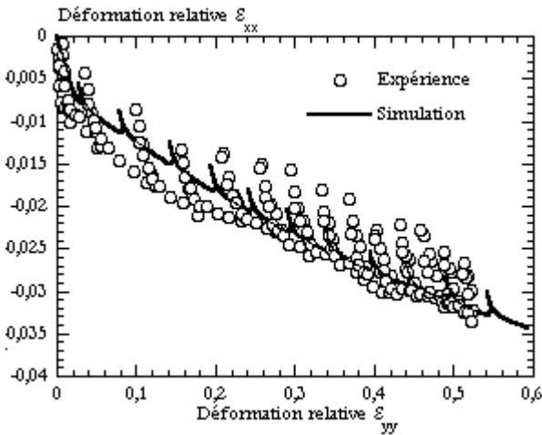
Fig. V-24 Evolution de la déformation transverse mesurée ou issue de la simulation d'essais de traction cyclique du BMT222.
