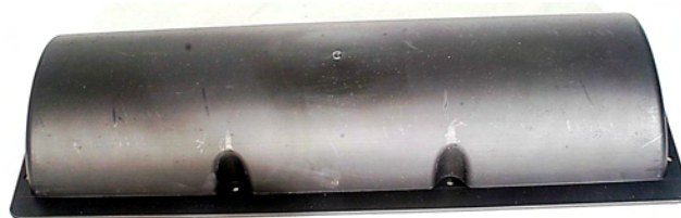
Fig. I-6 Photo d'une gouttière. Dimensions : 525 \times 185 \times 3 \text{ mm}^3 , hauteur 70 mm .
