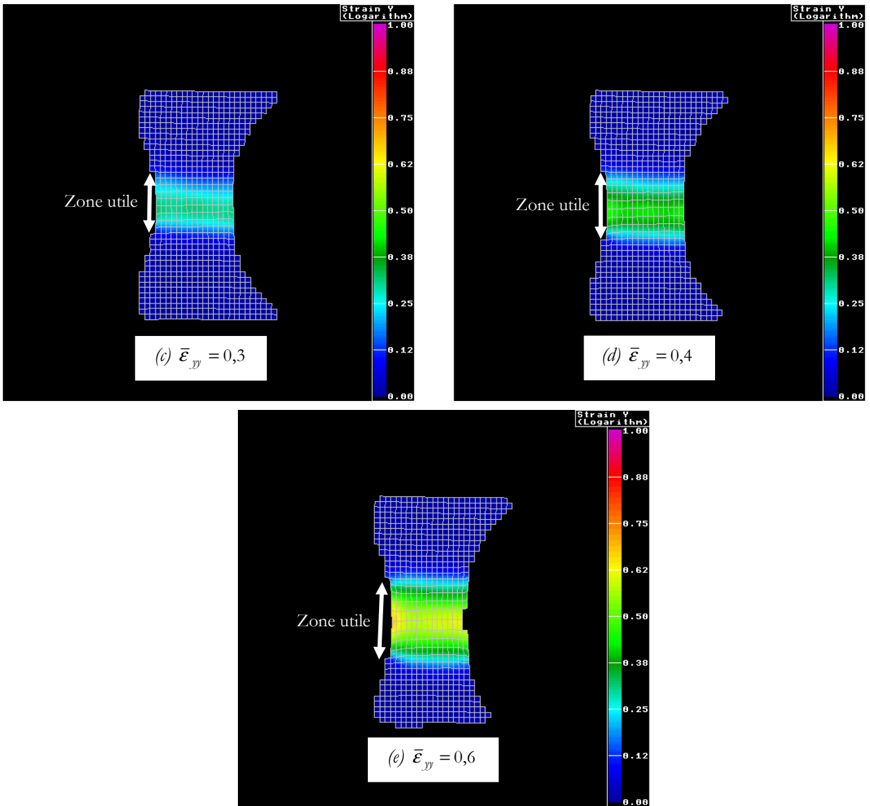
Fig. III-7 Evolution de la déformation longitudinale d'une éprouvette BMT222 au cours d'un essai de traction à 0,2 s^{-1} et à 20^{\circ}C .
