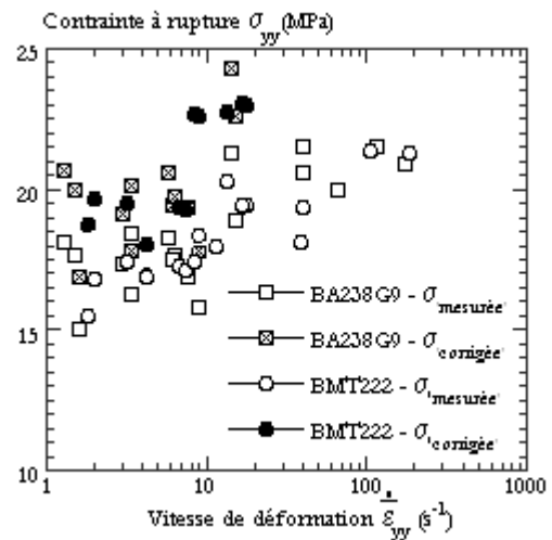
Fig. IV-11 Contraintes mesurées ou corrigées des effets de l'adoucissement thermique à rupture en tant que fonction de la vitesse de déformation longitudinale au cours d'une sollicitation en traction. Eprouvettes sollicitées parallèlement au sens d'injection.
