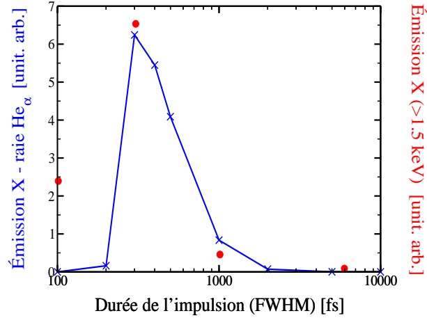
FIG. 5.9 – ( \times — \times ) Variation de l'émission X pour la raie He_{\alpha} (3,14 keV) en fonction de la durée d'impulsion. Ces résultats ont été obtenus pour une énergie par impulsion de 50 mJ et une longueur d'onde de 800 nm. Le rayon de l'impulsion en 1/e de l'intensité est de 10 \mu\text{m} , ce qui donne un éclairement crête de 1,3 \times 10^{17} \text{ W.cm}^{-2} pour une durée d'impulsion à mi-hauteur de 100 fs. (•) Données expérimentales obtenues par E. Parra et coll. pour l'émission X supérieure à 1,5 keV [Parra et al. 00].
