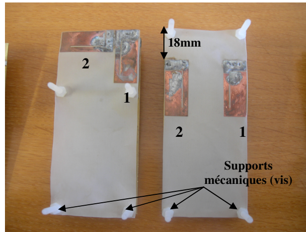
Figure 14 : Antenne de téléphone mobile à courts-circuits filaires et substrat fin (prototype 2) pour applications UMTS (à gauche la configuration orthogonale, à droite la configuration parallèle)
