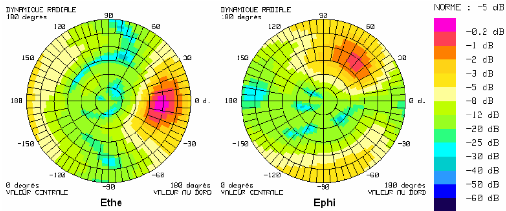
Figure 29 : Diagramme de rayonnement du premier élément (projet ERMITAGES)
