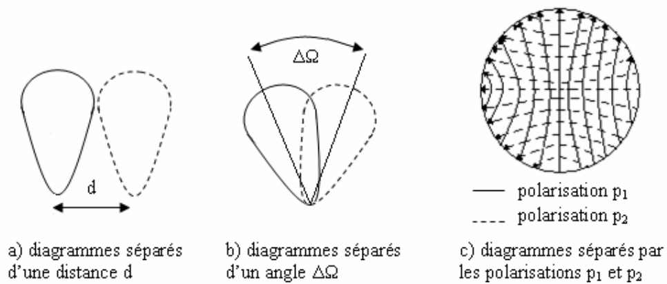
Figure 5 : Types de diversité antennaire : a) diversité d'espace, b) diversité de diagramme, c) diversité de polarisation
