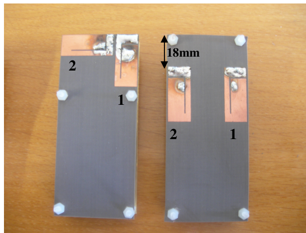
Figure 16 : Antenne de téléphone mobile à courts-circuits filaires et substrat épais (prototype 3) pour applications UMTS (à gauche la configuration orthogonale, à droite la configuration parallèle)
