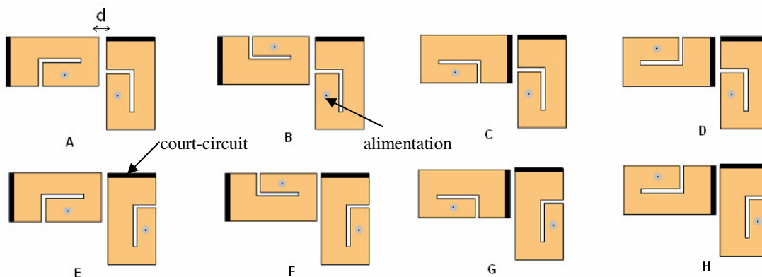
Figure 12 : Géométries possibles de l'antenne bi-patchs orthogonaux. Pour minimiser le couplage et optimiser l'adaptation, on retient la configuration H
