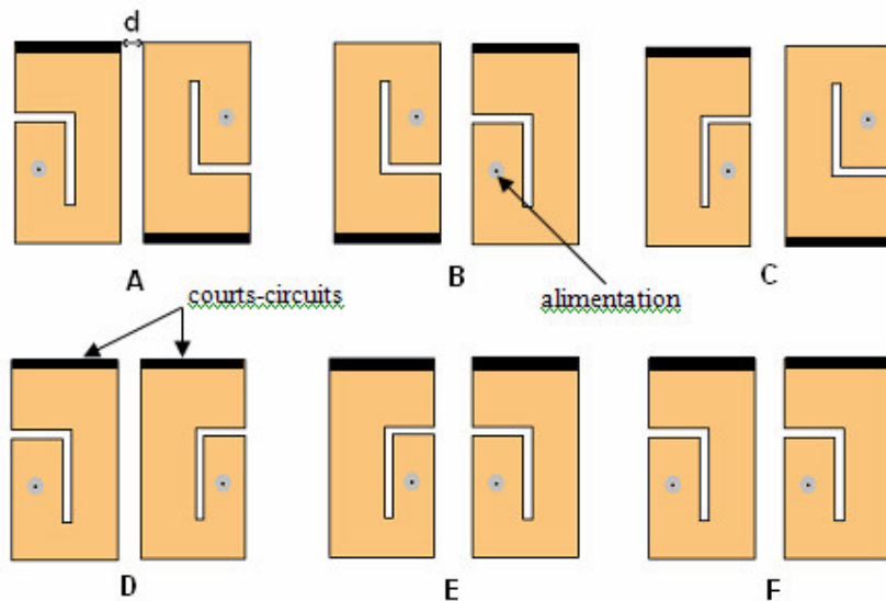
Figure 11 : Géométries possibles de l'antenne bi-patchs parallèles. Pour minimiser le couplage, on choisit la configuration D
