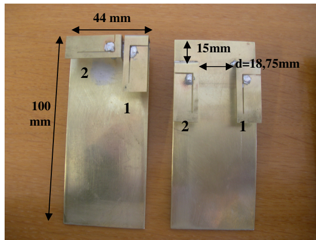
Figure 13 : Antenne de téléphone mobile à courts-circuits plans (prototype 1) pour applications UMTS (à gauche la configuration orthogonale, à droite la configuration parallèle)
