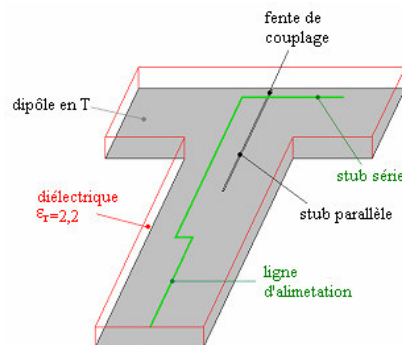
Figure 44 : Dipôle en T
