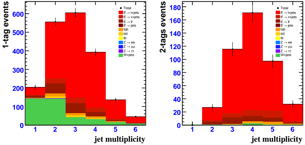
FIG. 7.2.21 – Nombre d'événements sélectionnés dans le canal \mu + jets , en fonction du nombre de jets sélectionnés, avec exactement un jet étiqueté b (à gauche) et deux jets étiquetés b (à droite). Ces nombres d'événements sont normalisés à une luminosité intégrée de 100 \text{ pb}^{-1} . Seuls les événements ayant au moins trois jets sont comptabilisés pour l'estimation de \sigma(t\bar{t}) . Le dernier intervalle de multiplicité est inclusif.
