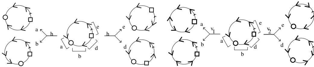
Fig. 6.12. Examples of transformations h, v_1, v_2 .
