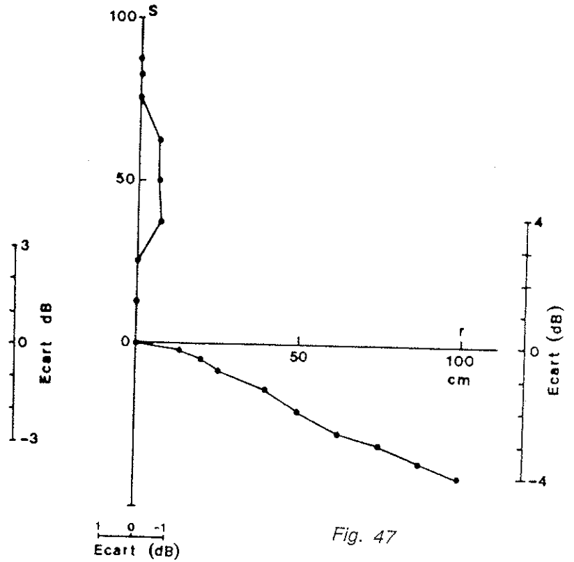
Figures 46, 47: Mesures de directivité de la source (chambre sourde)
