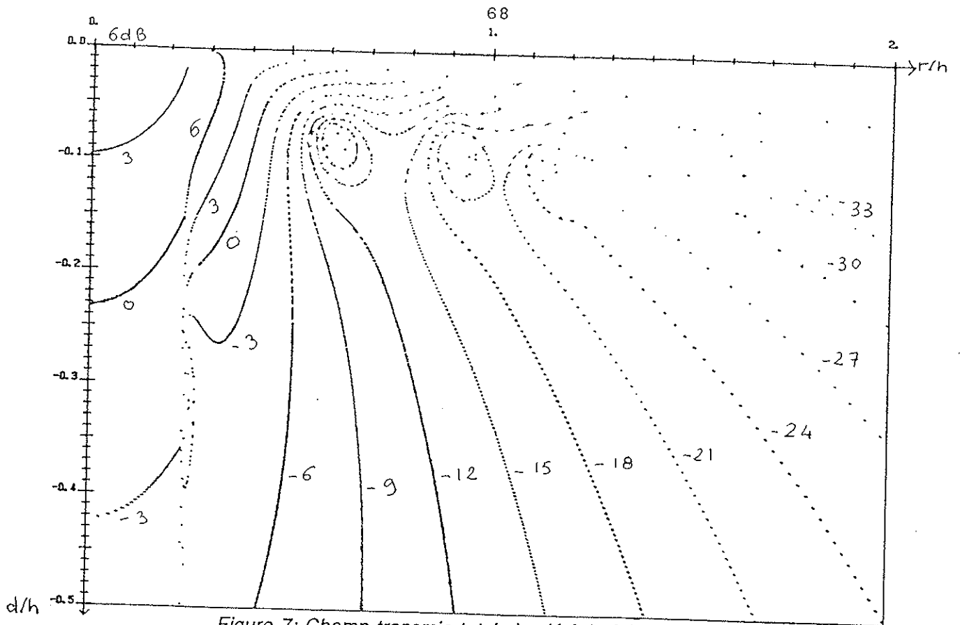
Figure 7: Champ transmis total simulé à la fréquence 3kHz.
