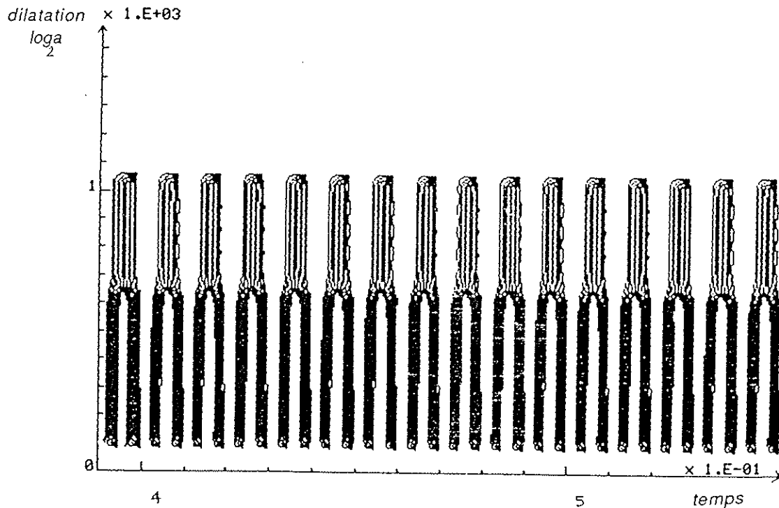
Figure 3.p: Phase de la transformée en ondelettes de la somme de 2 sinusôides de 100Hz et 200Hz. Mêmes paramètres que la figure 3.m.
