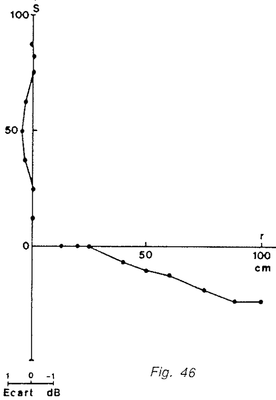
Figures 46, 47: Mesures de directivité de la source (chambre sourde)
