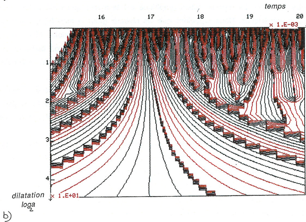
Figure 17.a: Module de la transformée en ondelettes du signal source.
