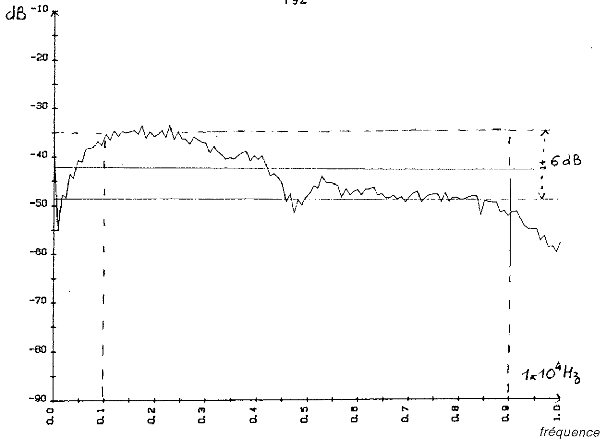
Figure 15.a: Spectre du signal source. (Réponse constante à ±6dB).
