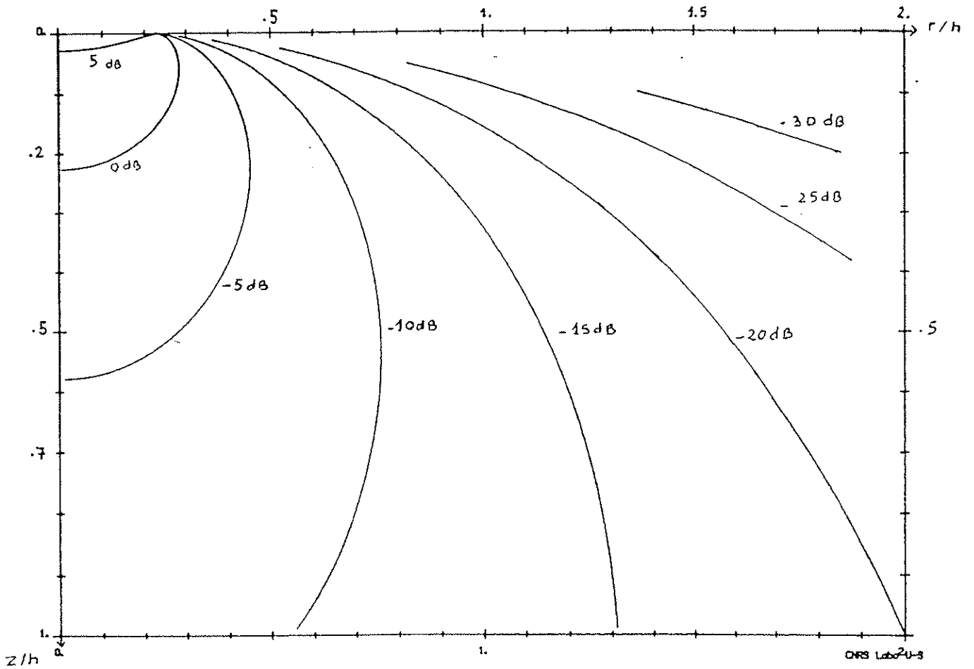
Figure 4: Courbes d'isoatténuation de l'onde géométrique réfractée selon (2.33), en fonction des variables réduites r/h , z/h (coordonnées de l'hydrophone). Discrétisation par pas de 5dB. (Méthode asymptotique).
