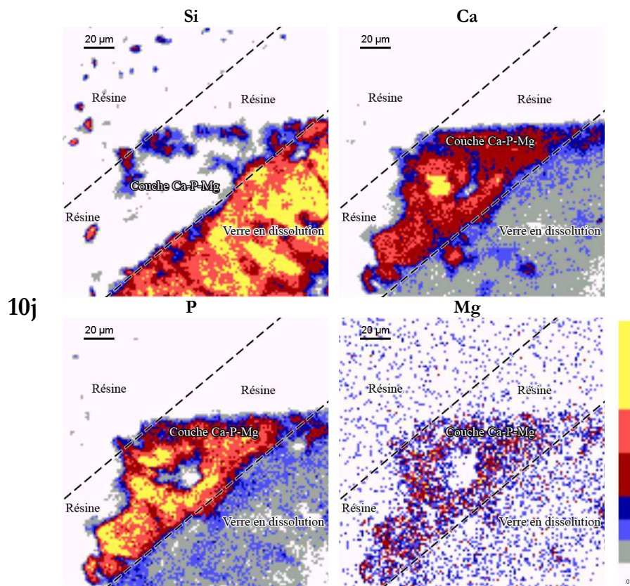
Figure 7-8: distribution des éléments silicium, calcium, phosphore et magnésium dans une pastille de verre B67,5 de composition \text{SiO}_2\text{-CaO-P}_2\text{O}_5 après 10 jours d'interaction avec le milieu biologique.
