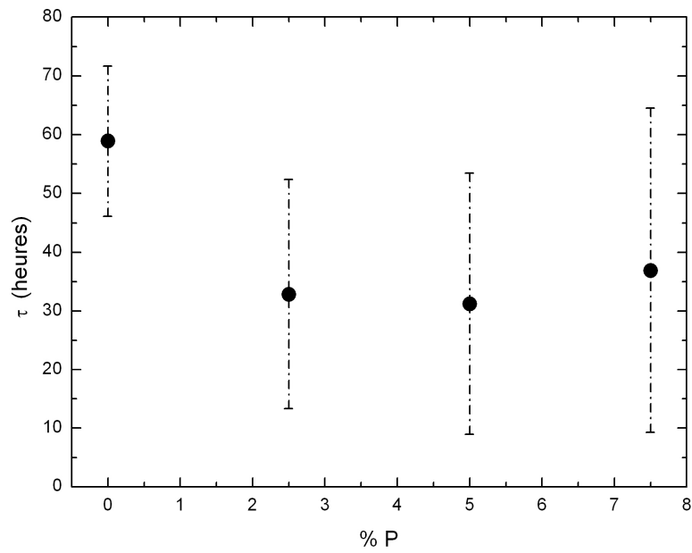
Figure 10-5: évolution du paramètre \tau en fonction de la teneur en phosphore dans les pastilles de verre bioactif.
