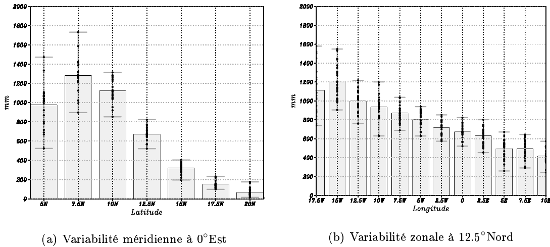
FIG. 6.1: Cumul annuel des précipitations sur la longitude 0^{\circ} Est entre 5^{\circ} Nord et 20^{\circ} Nord (barres) et variabilité interannuelle (points) entre 1968 et 1990 (a), idem pour la latitude de 12^{\circ}5 Nord et entre -17.5^{\circ} Est et 10^{\circ} Est (b).
