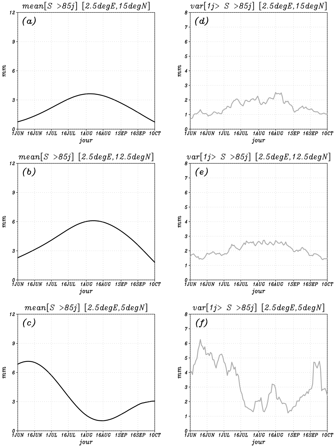
FIG. 6.8: Signaux de pluies filtrés dans les gammes de périodes au dessus de 85 jours a , b , c ) ou entre 1 et 85 jours (d, e, f) aux latitudes 5°, 12.5° et 15° Nord et la longitude 2.5°E pour l'année 1976.
