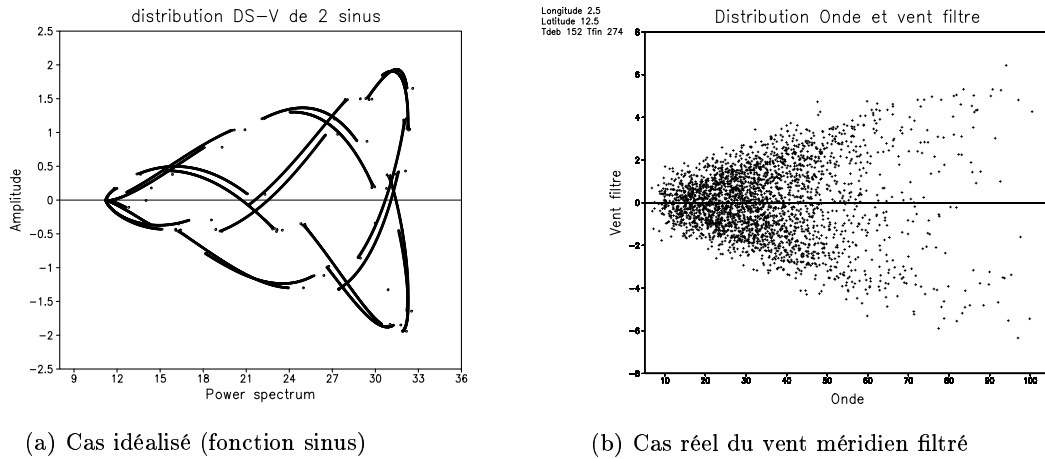
FIG. 4.7: Distribution des indices DS de l'analyse en ondelettes suivant soit la fonction sinus (cas idéalisé), soit du vent méridien à 700 hPa (en m^2 \cdot s^{-2} ) en fonction de l'amplitude du vent méridien filtré à 700 hPa.
