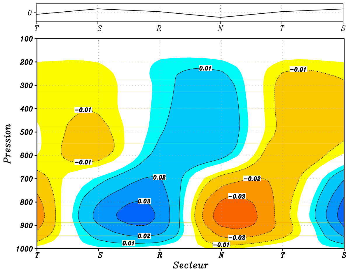
FIG. 9.9: Profil vertical des vitesses verticales totales suivant les secteurs sur le point de grille 17.5^\circ Est, 12.5^\circ Nord (en Pa.s^{-1} ). Les secteurs sont identifiés par le vent meridien ( haut )
