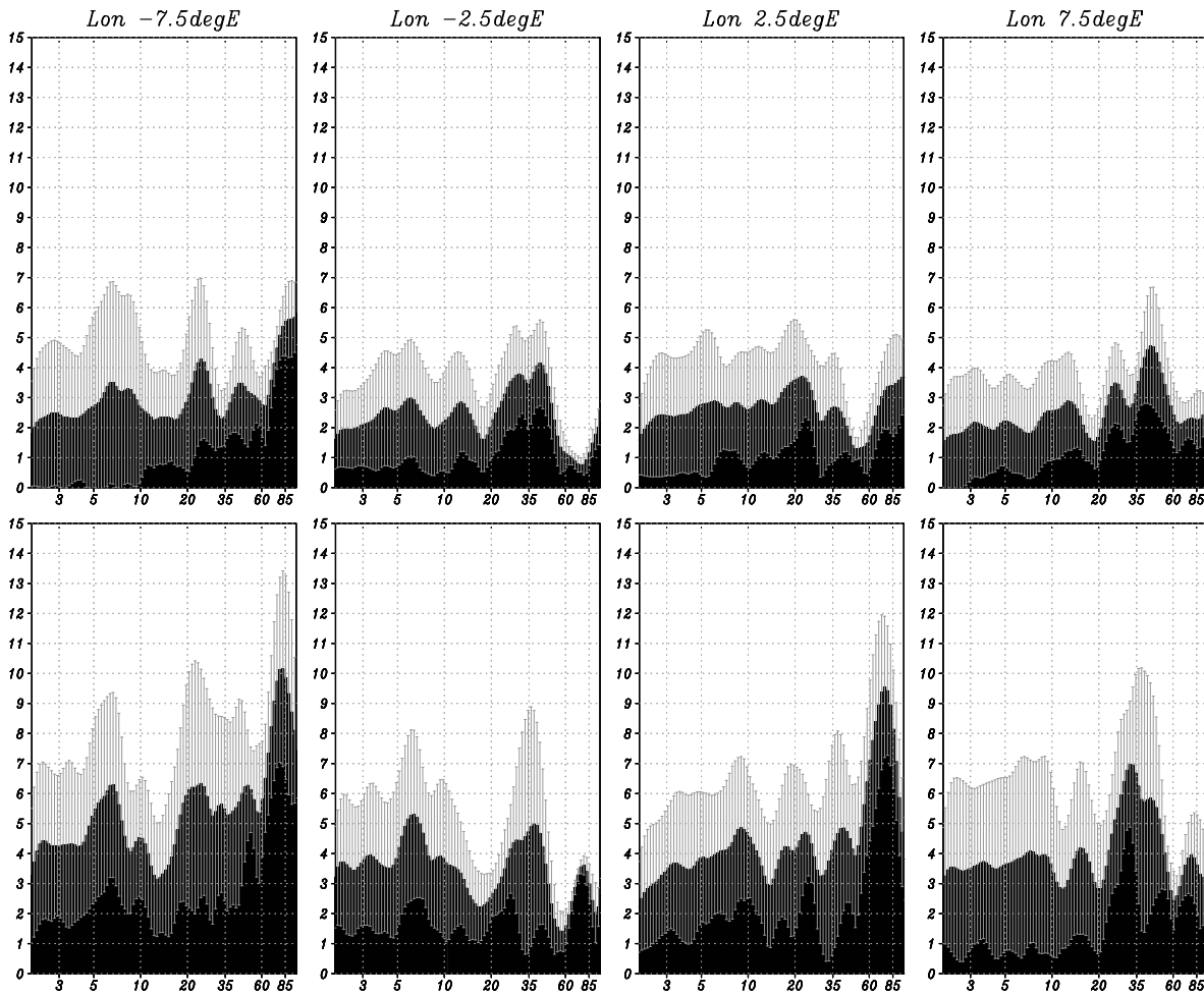
FIG. 6.7: Moyenne des densités spectrales du signal de pluie ( barres ), et le seuil de significativité à 95 % ( barres d'incertitudes ) sur la région Sahélienne, entre -7.5^{\circ}E;7.5^{\circ}E et 12.5^{\circ}N(bas);15^{\circ}N(haut) pour l'année 1976.
