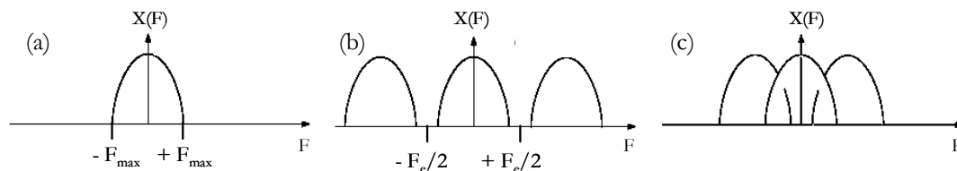
Figure 2.3 : (a) Spectre en fréquence du signal non-échantillonné. (b) Effet de l'échantillonnage sur le spectre du signal : périodisation du spectre à la fréquence F_E=1/T_E (c) Répartition spectrale lorsque la cadence d'échantillonnage n'est pas suffisante : repliement de spectre.
