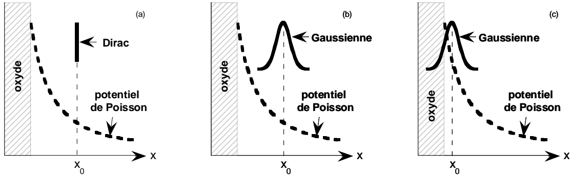
Figure 2.1 : Produit de convolution pour un paquet d'ondes représenté par un Dirac (a) ou par une distribution gaussienne (b et c) à différentes positions x_0 .
