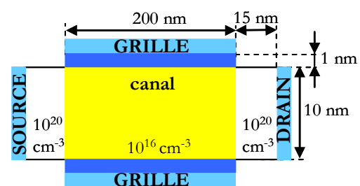
Figure 2.9 : Dispositif double-grille simulé.
