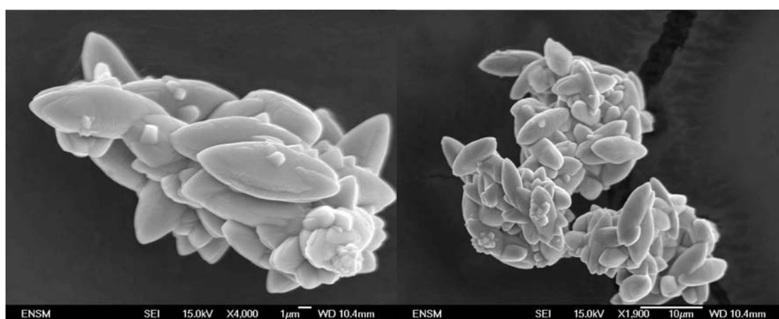
Figure 4.10- Photos MEB du \text{SrMoO}_4 en fin de précipitation obtenue à 500 \text{min}^{-1} (conditions de précipitation : 25°C, 25 \text{mol.m}^{-3} , hélice Mixel TT).
