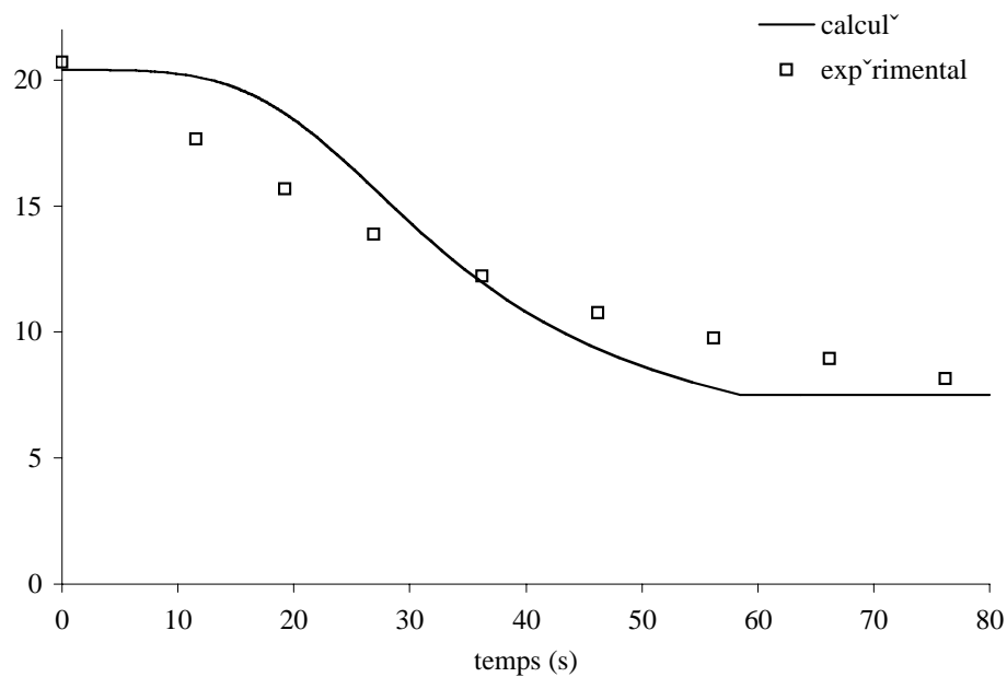
Figure 5.14 - Evolution de la concentration calculée et expérimentale (conditions de précipitation : 25 \text{ mol.m}^{-3} , 50^\circ\text{C} , 350 \text{ min}^{-1} , heliciel Mixel TT).
