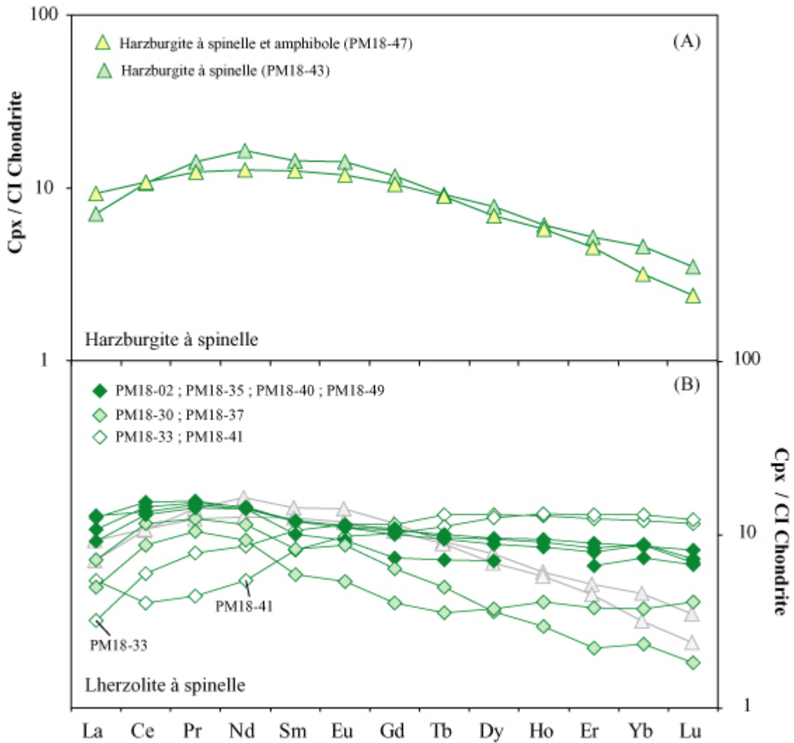
Figure VI-21 : Diagrammes des terres rares (REE) des clinopyroxènes des péridotites à spinelle de Pali Aike. En (A), les spectres sont ceux des clinopyroxènes de la harzburgite anhydre ( HS_A , PM18-43) et de la harzburgite à amphibole ( HS_{HA} , PM18-47). En (B), les spectres correspondent aux cpx des lherzolites à spinelle anhydres de Pali Aike. La variation de couleur des losanges est faite pour montrer clairement les trois types de spectres différents observés. Les spectres en gris clairs sont ceux des cpx présentés en (A). La normalisation est faite aux chondrites CI de Mc Donough et Sun (1995).
