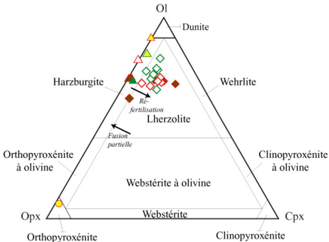
Figure VI-11 : Diagramme de Streickeisen (1973) dans lequel est reporté les échantillons de la Laguna Timones (Pali Aike).
