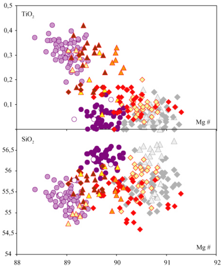
Figure VI-14: Diagramme TiO_2 et SiO_2 vs Mg\# [ Mg / (Mg + Fe_{Tot}) * 100 ] des orthopyroxènes des enclaves ultramafiques à grenat de Pali Aike. Les symboles en gris correspondent aux compositions des orthopyroxènes des enclaves à spinelle présentées dans la Figure VI-12.
