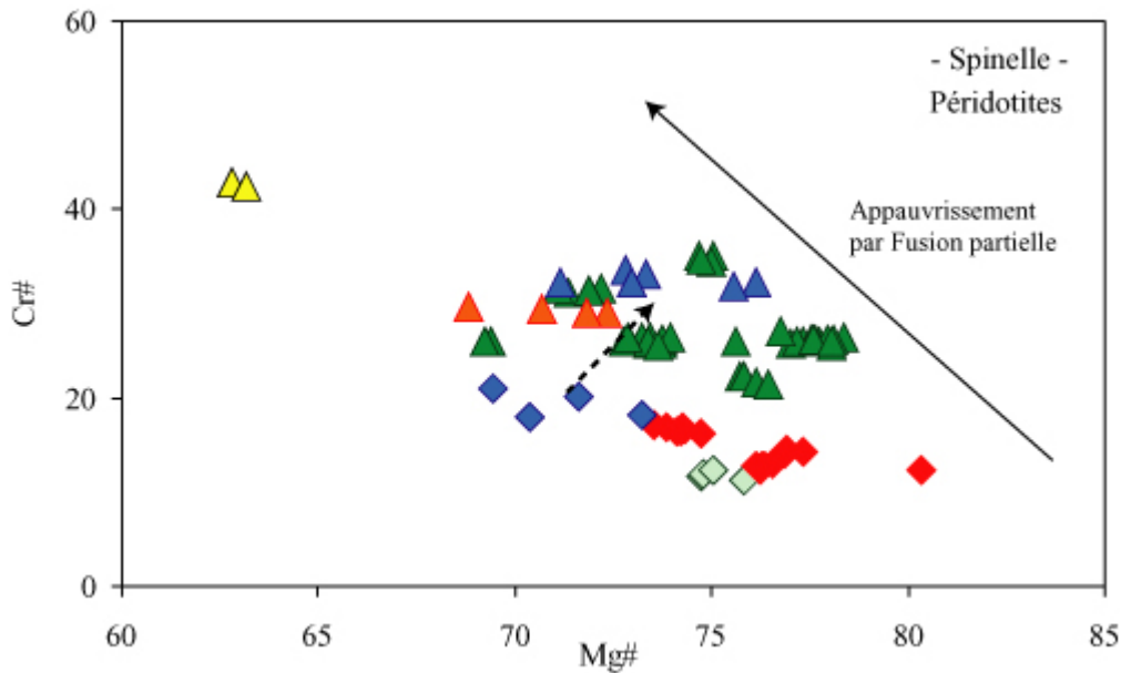
Figure IV-17: Diagramme Cr\# [= Cr / (Cr+Al) \times 100 ] vs Mg\# [= Mg / (Mg+Fe_{Tot}) \times 100 ] dans les spinelles des péridotites de la zone Nord Patagonienne. La légende en figure IV-12. La flèche noire représente le trend contrôlé par le processus de fusion partielle (Hellebrand et al. , 2001)
