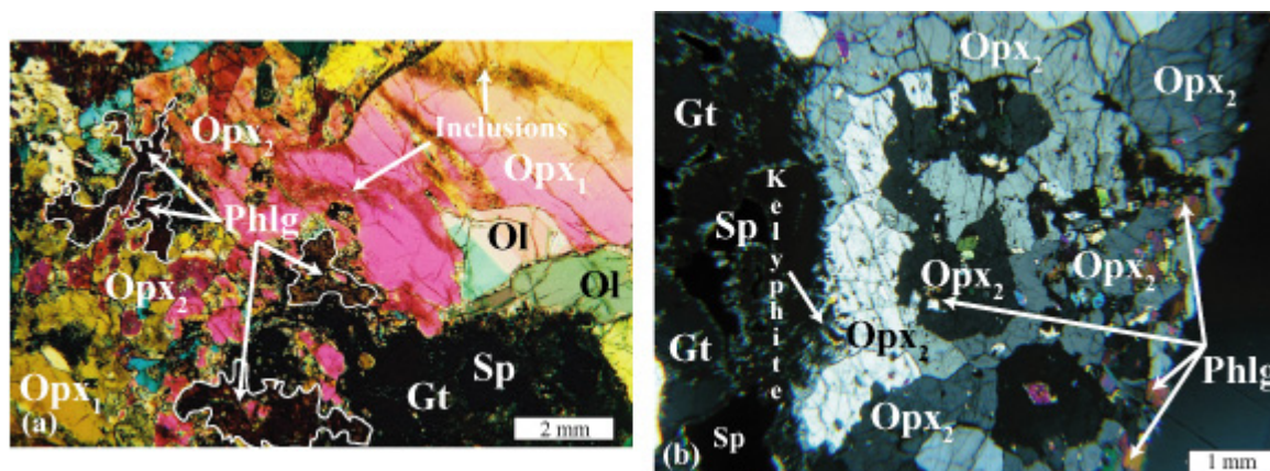
Figure VI-9 : Au cœur de la veine, les orthopyroxènes sont automorphes (Opx-1, a) ou xénomorphes (Opx-2,b). Les opx automorphes sont démantelés en un amas de grains xénomorphes (a). Ces dégénérescences sont associées aux phlogopites interstitielles. Les orthopyroxènes nommés opx-2, également associés aux phlogopites, semblent correspondre aux orthopyroxènes dégénérés, mais de plus grande taille (b). Les orthopyroxènes (opx-2) ont cristallisé dans la couronne kélyphitique du grenat (b).
