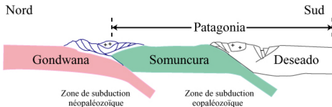
Figure II-3: Coupe Schématique de la collision N-S des microplaques Somoncuro et Deseado (Ramos, 2002).
