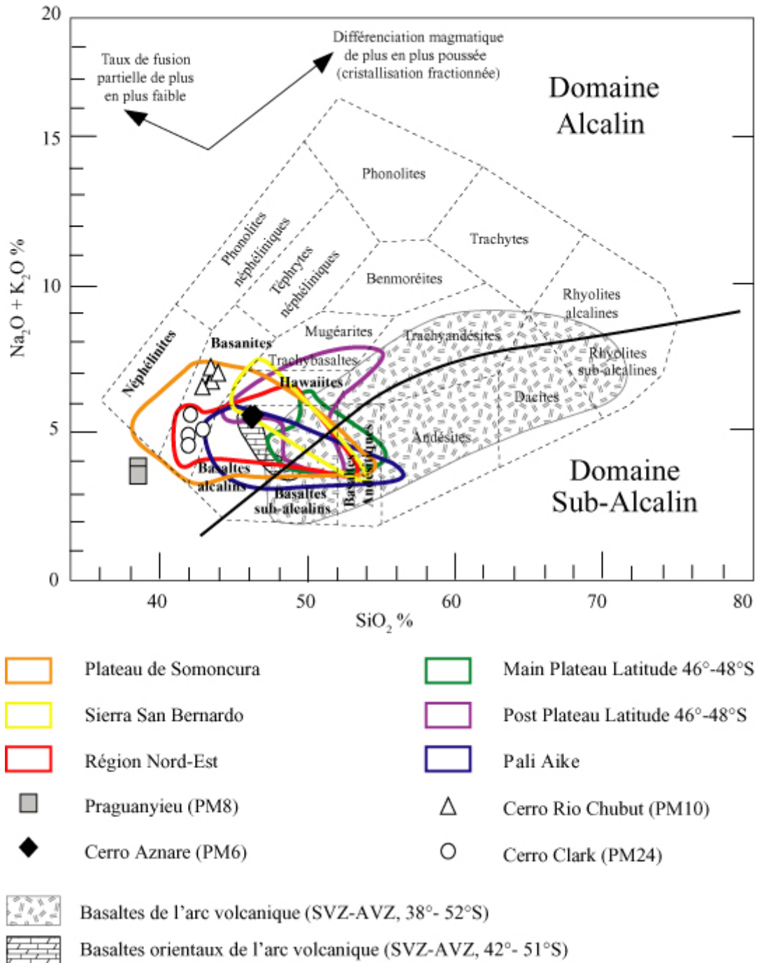
Figure III-2 : Classification de Cox et al. (1979), basée sur le diagramme alcalins ( \text{Na}_2\text{O}+\text{K}_2\text{O} ) vs silice (dit de Harker, 1909), permettant de visualiser les grands domaines magmatiques. Les symboles (carré, triangle, diamant et cercle) représentent les laves hôtes, contenant des enclaves mantelliques, de cette étude. Tous les champs représentés dans ces diagrammes, représentent des basaltes porteurs d'enclaves mantelliques, à
