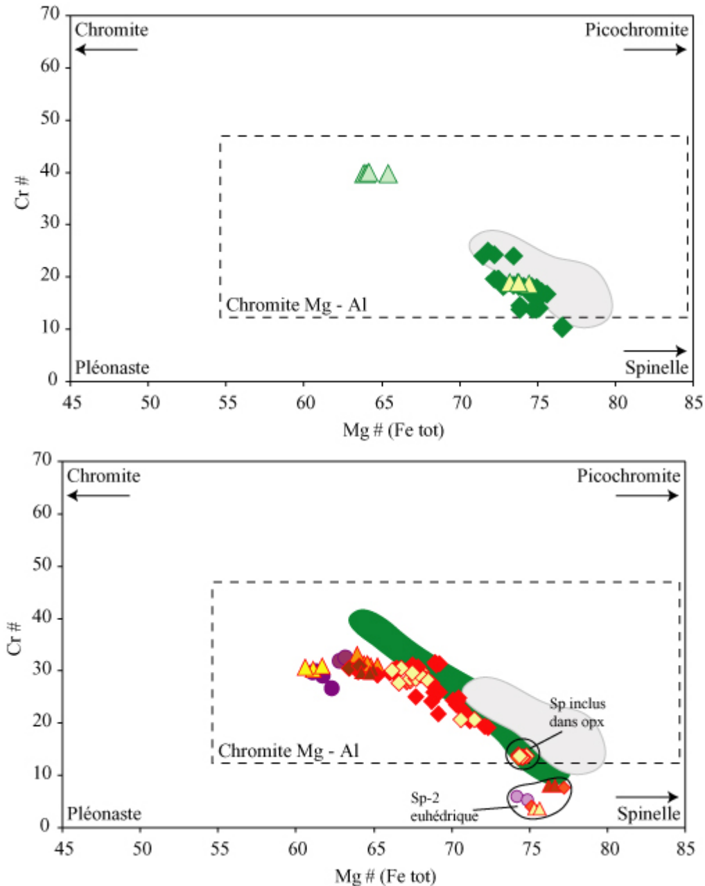
Figure VI-17: Diagramme Cr# [= Cr / (Cr+Al)*100] vs Mg# [= Mg / (Mg+Fe Tot )*100] des spinelles des péridotites à spinelle de Pali Aike (en haut) et des péridotites à grenat et de l'orthopyroxénite de Pali Aike (Laguna Timones, en bas). Le champ gris représente la composition des spinelles des péridotites anhydres de Tres Lagos. Le champ vert (en bas) représente les spinelles des péridotites à spinelle de Pali Aike (cette étude).
