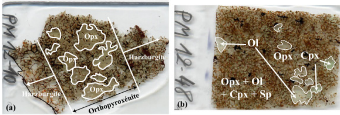
Figure IV-9: Photographies des sections épaisses de l'échantillon composite PM12-10 (a) et de la lherzolite PM12-48 (b). Nous notons l'altération rouge typique des minéraux des échantillons de Cerro de Los Chenques. Les orthopyroxènes au cœur de l'orthopyroxénite sont de grandes tailles, aux bords courbes, comparés à ceux contenus dans l'encaissant (harzburgite). Dans PM12-48 (b), des olivines, des orthopyroxènes et des clinopyroxènes de grandes tailles par rapport au reste de l'échantillon sont dépourvues de l'altération rouge.
