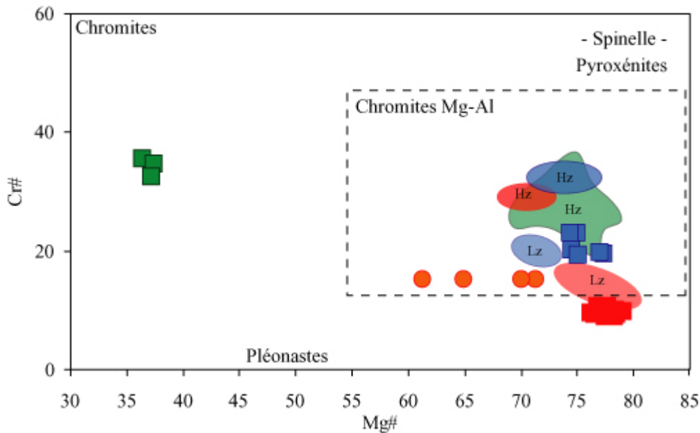
Figure IV-18: Diagramme Cr# [= Cr/(Cr+Al)*100] vs Mg# [= Mg/(Mg+Fe Tot )*100] dans les spinelles des pyroxénites de la zone Nord Patagonienne. Les champs rouge (PM12), vert (PM10) et bleu (PM8) représentent les spinelles des péridotites (Hz : harzburgites ; Lz : Lherzolites) de la Figure IV-18. Un complément de légende est fait en annexe (marque page A). La nomenclature est d'après Haggerty (1981).
