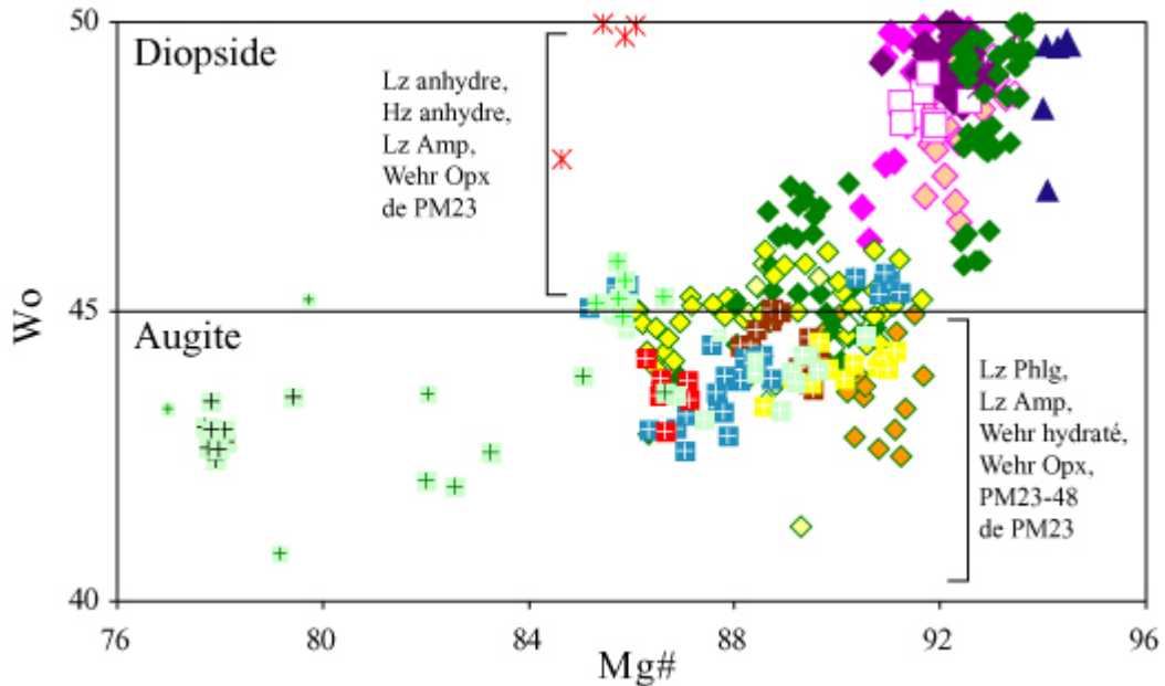
Figure V-19 : Diagramme Wo [ Ca / (Ca + Fe_{Tot} + Mg) * 100 ] vs Mg# [ Mg / (Mg + Fe_{Tot}) * 100 ] des clinopyroxènes des enclaves de Cerro Clark et de Gobernador Gregores. Pour des Wo compris entre 45 et 50 %, les clinopyroxènes sont des diopsides, alors que ceux avec Wo < 45\% sont des augites d'après la classification de Morimoto et al. (1988).
