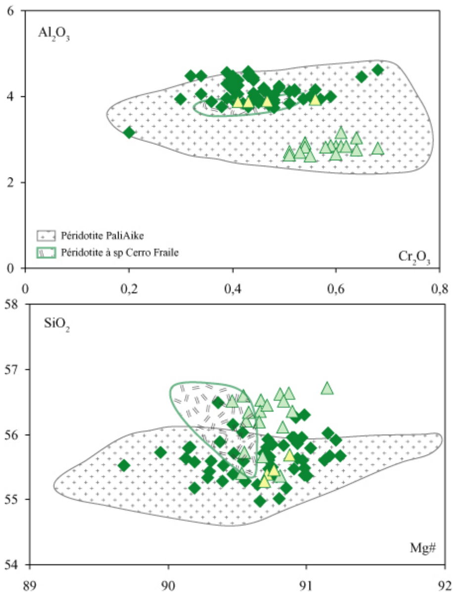
Figure VI-12 : Diagrammes Al 2 O 3 vs Cr 2 O 3 et SiO 2 vs Mg# [ \text{Mg} / (\text{Mg} + \text{Fe}_{\text{Tot}}) * 100 ] des orthopyroxènes des enclaves ultramafiques à spinelle de Pali Aike (PM18, Laguna Timones). Le champ cerclé de vert correspond aux orthopyroxènes de Cerro Fraile (Kilian et al. , 2002), situé à moins de 25 km de l'arc volcanique (~50°S). Le
