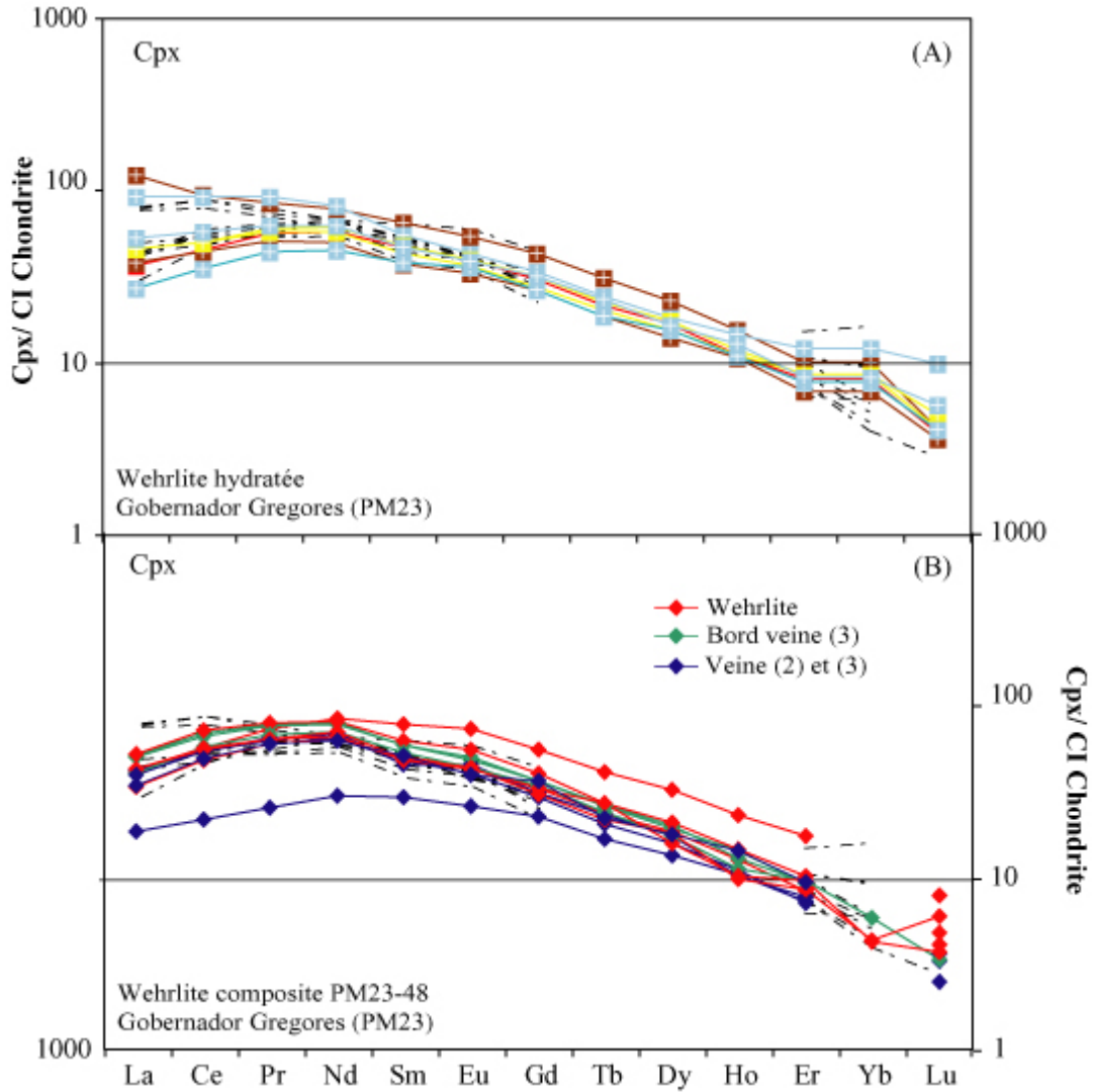
Figure V-32 : Diagrammes des terres rares (REE) des clinopyroxènes des wehrlites hydratées (A) et de la wehrlite composite PM23-48 (B) de Gobernador Gregores (PM23). Les pointillés représentent les spectres des cpx des lherzolites hydratées de Gobernador Gregores, définis comme riche en titane par Rivalenti et al. (2004a). La normalisation est faite aux CI chondrites de Mc Donough et Sun (1995). Le complément de légende est disponible en annexe.
