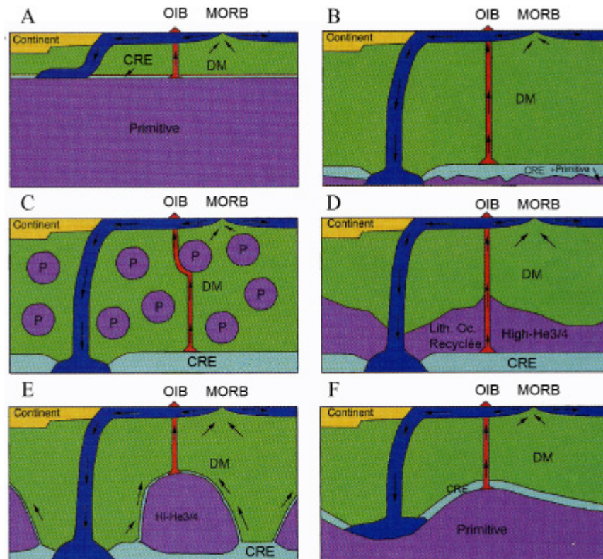
Figure I-2: Localisations possibles des réservoirs mantelliques et de leurs relations à la dynamique du manteau (Tackley, 2000). Sur ce schéma, le bleu représente les plaques océaniques et les slabs 1 , et le rouge, les plumes mantelliques chaudes. Les réservoirs géochimiques sont les suivants : en vert, le manteau appauvri (DM) ; en violet, les zones à fort rapport ^3\text{He}/^4\text{He} (« primitive ») et en bleu clair, la Croûte Recyclée Enrichie (CRE). A - modèle typique géochimique stratifiée à 660 km de profondeur (Hofmann, 1997). B - modèle typique géodynamique : homogène excepté à la base du manteau avec des mélanges de CRE et du manteau primitif. C - modèle des gouttes primitives avec un niveau à la base de CRE (Becker et al. , 1999). D - modèle de recyclage complet (Albarède, 1998 ; Coltice et Ricard, 1999). E - modèle primitif d'empilement (Tackley, 1998). F - Modèle de stratification primitive profonde (Kellogg et al. , 1999).
