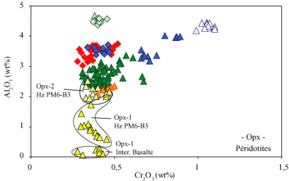
Figure IV-13: Diagramme chrome - aluminium des orthopyroxènes des enclaves péridotitiques de la zone Nord Patagonienne. La légende est présentée en annexe (marque-page A). Inter. Basalte : Interactions avec la lave hôte.
