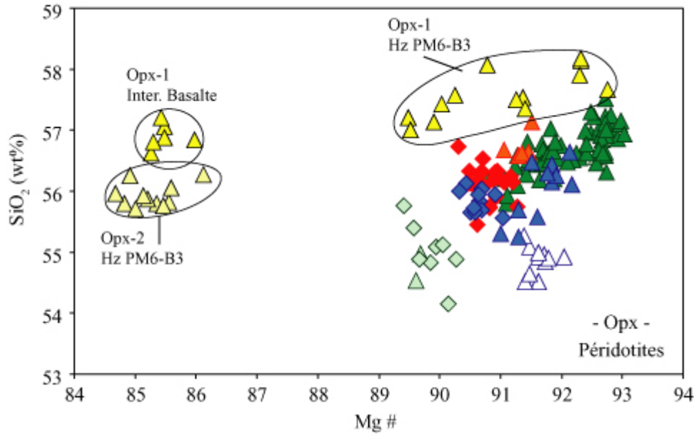
Figure IV-12: Diagramme SiO 2 vs Mg# [Mg/(Mg+FeO Tot )*100] des orthopyroxènes des enclaves péridotitiques de la zone Nord Patagonienne. La légende est présentée en annexe (marque-page A).
