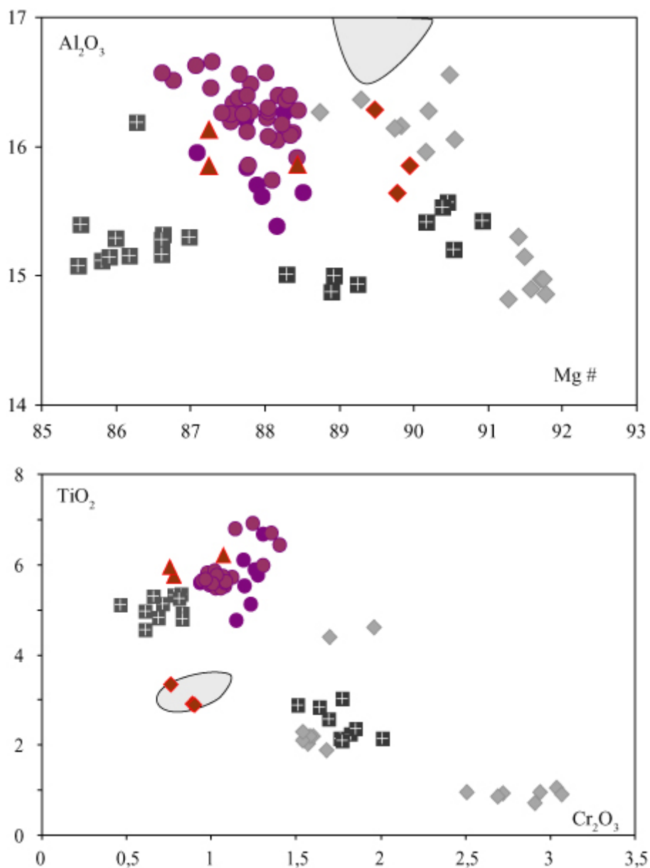
Figure VI-20: Diagrammes binaires Al_2O_3 vs Mg\# [ (Mg / (Mg + Fe_{Tot})) \times 100 ] et TiO_2 vs Cr_2O_3 des phlogopites de la lherzolite PM18-36 (losange), de la harzburgite PM18-24 (triangle) et de l'orthopyroxénite PM18-01 (rond) de Pali Aike. Le champ gris correspond aux phlogopites des péridotites de Cerro Rio Chubut de la zone Nord Patagonienne (PM10, voir Chapitre IV) et les symboles gris représentent les phlogopites des péridotites de Gobernador Gregores (PM23, voir Chapitre V).
