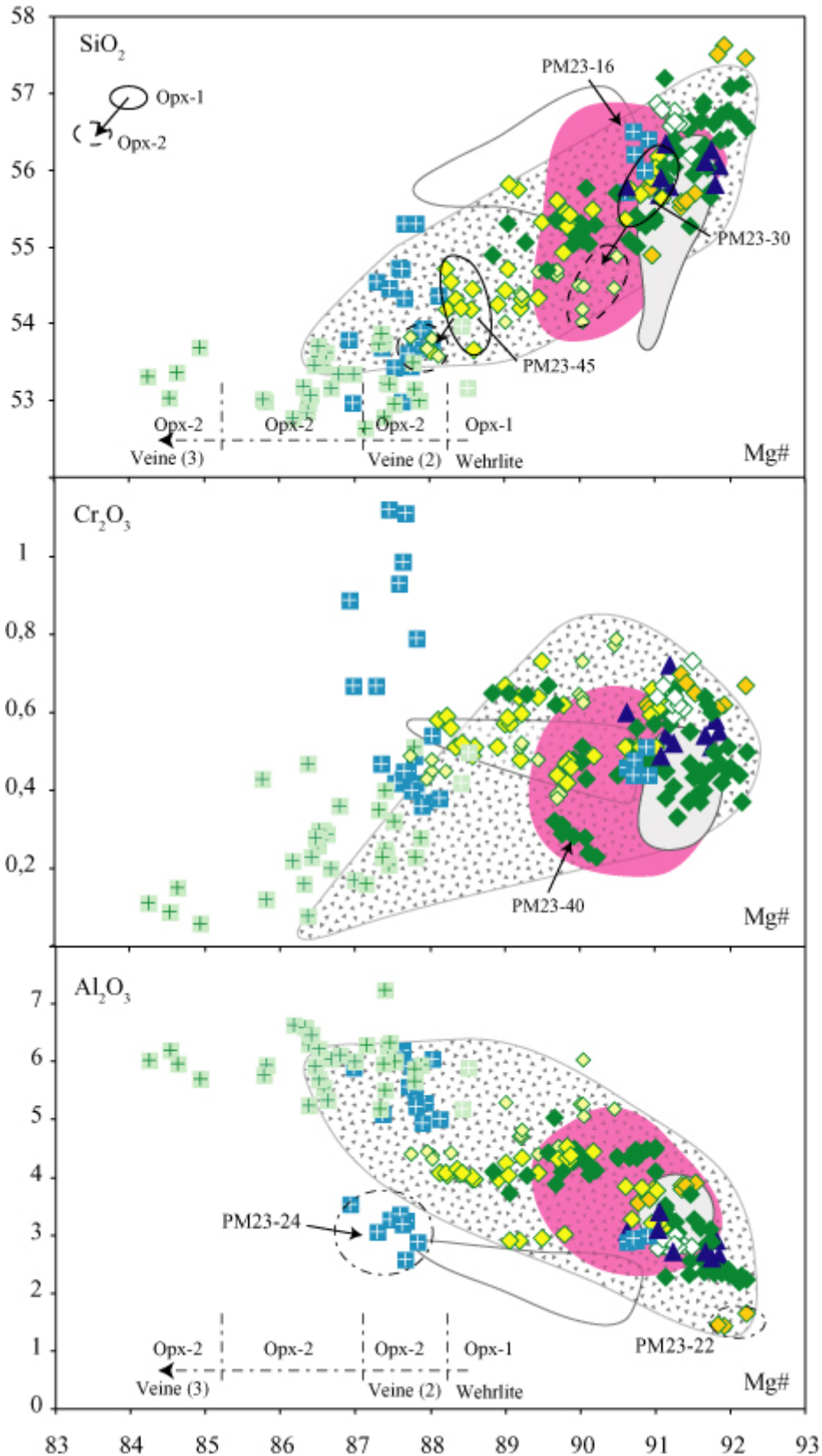
Figure V-18: Diagrammes SiO 2 , Cr 2 O 3 et Al 2 O 3 vs Mg# [ Mg/(Mg+Fe_{Tot}) * 100 ] de l'orthopyroxène dans les péridotites de Gobernador Gregores (PM23). La zone rose représente les compositions des orthopyroxènes des lherzolites de Cerro Clark (Figure V-17). Les champs blancs et tachetés représentent les compositions des opx
