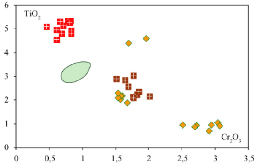
Figure V-26 : Diagrammes \text{Al}_2\text{O}_3 vs Mg# [(\text{Mg}/(\text{Mg}+\text{FeTot})) \times 100] et \text{TiO}_2 vs \text{Cr}_2\text{O}_3 des phlogopites des péridotites de Gobernador Gregores. Le champ vert correspond aux phlogopites de péridotites de Cerro Rio Chubut (PM10, voir Chapitre IV) de la zone Nord Patagonienne.
