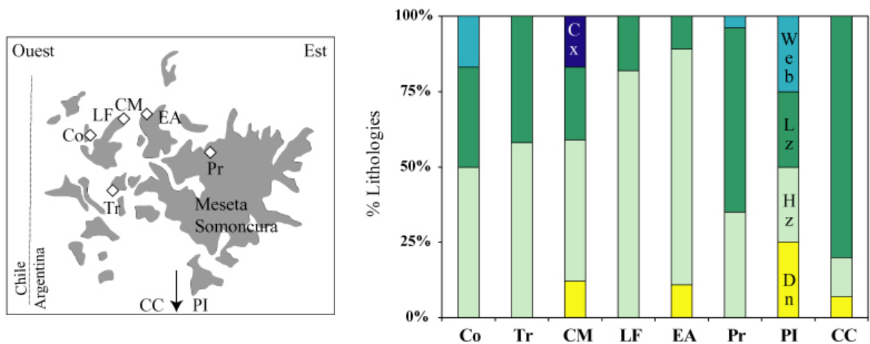
Figure IV-1 : Synthèse des différentes lithologies d'enclaves mantelliques étudiées dans les localités de la Meseta de Somoncura (carte de gauche) et de Canquel (CC et PI, Figure II-9, 13), dans les travaux de Ntaflos et al. (2001, 2002), Mallmann (2004), Rivalenti et al. (2004) et Bjerg et al. (2000a, b, 2005). Dn : Dunite ; Hz : Harzburgite ; Lz : Lherzolite ; Web : Webstérite ; Cx : Clinopyroxénite.
