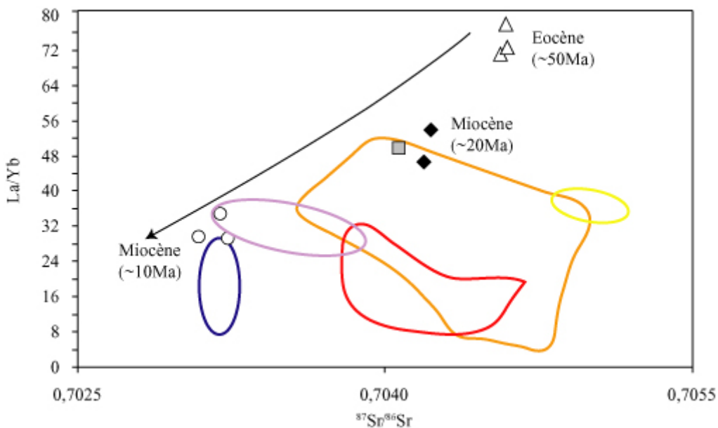
Figure III-8 : Diagramme La/Yb vs ^{87}\text{Sr}/^{86}\text{Sr} des basaltes. La légende est identique à celle de la figure III-2.
