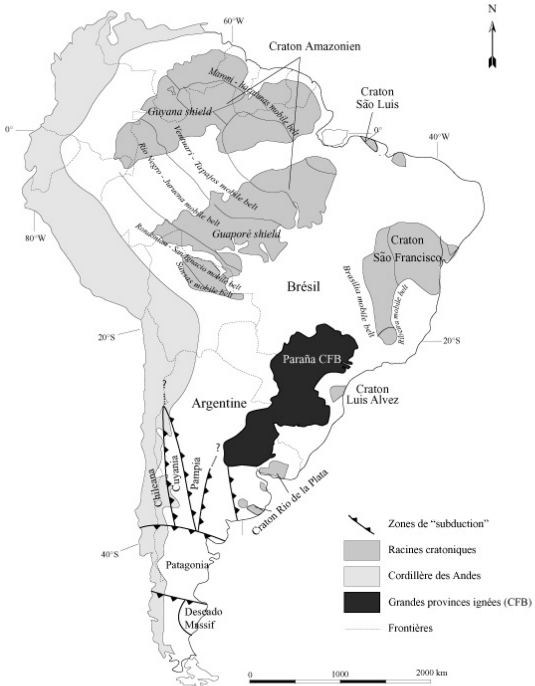
Figure II-2: Cartes d’Amérique du Sud sur laquelle sont reportées les anciens cratons du Brésil (marge sud-ouest du Gondwana), les différents « terranes » alloctones (Chilenea, Cuyania, Pampia, Patagonia, Deseado Massif ; Ramos, 1988) ainsi que les volumineux épanchements de basaltes continentaux tholeiitiques du Paraña (Kirstein et al. , 2001).
